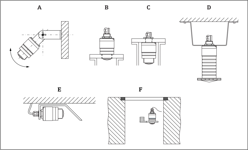
图 10 安装在墙壁上、罐顶上或安装短管中
