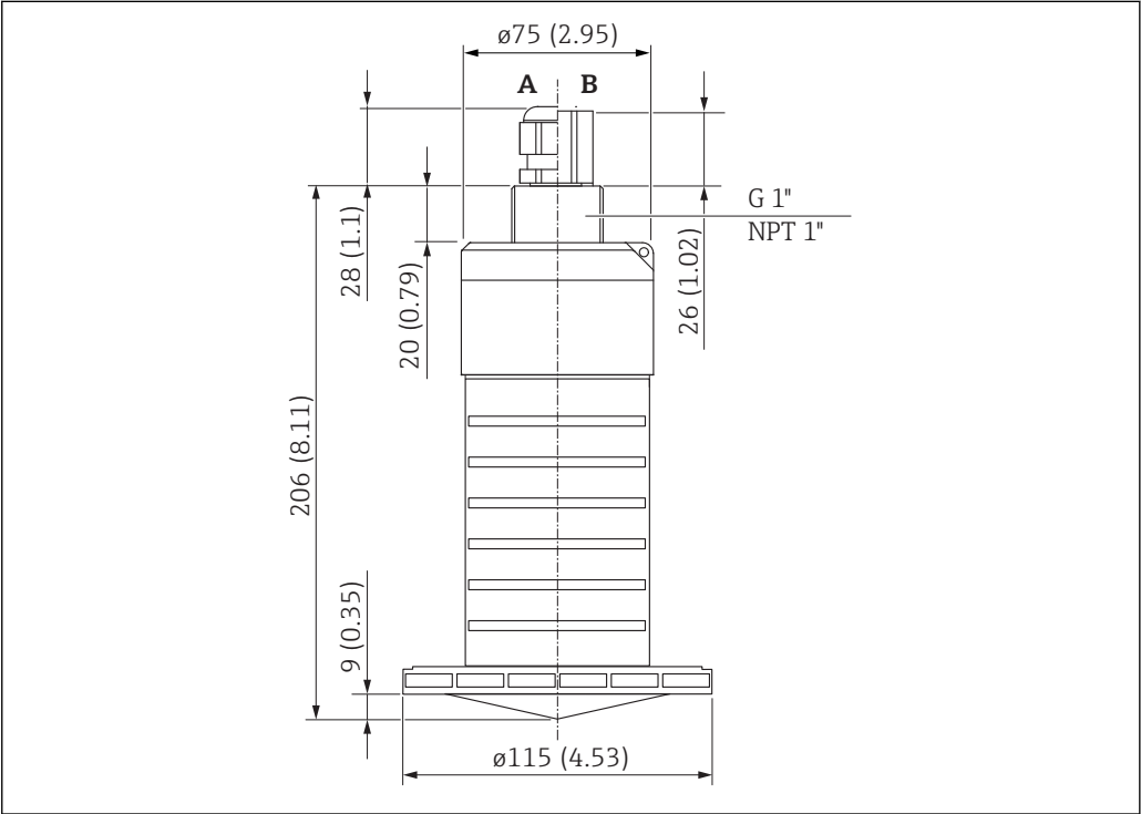
26 80 mm (3 in)口径天线的外形尺寸；单位：mm (in)
