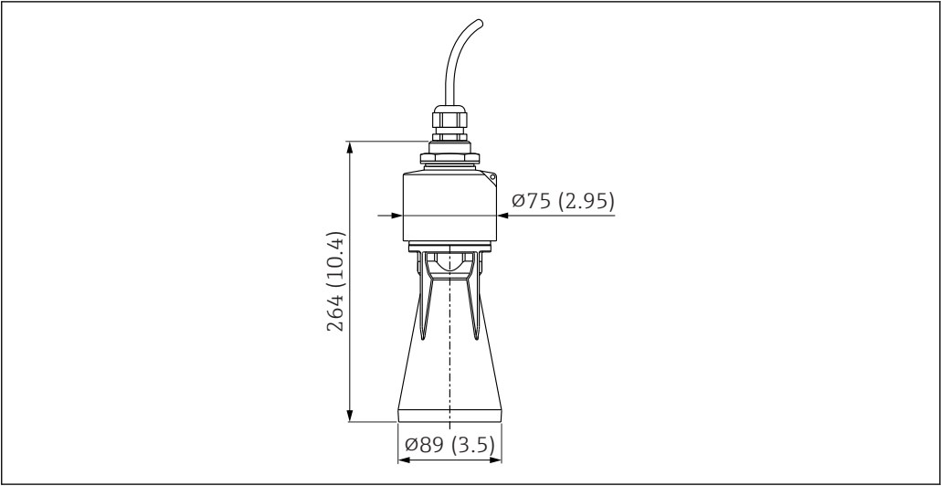
25 40 mm (1.5 in)口径天线的外形尺寸，安装有防溢管；单位：mm (in)
