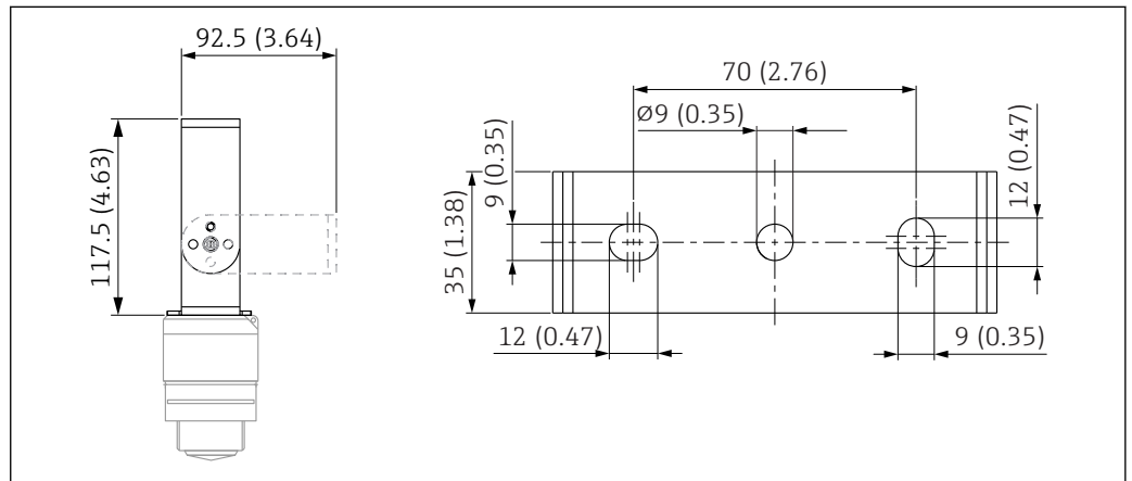
■ 40 墙装架的外形尺寸；单位：mm (in)
