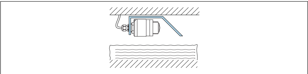
图 20 水平安装，同时安装有金属反射板
