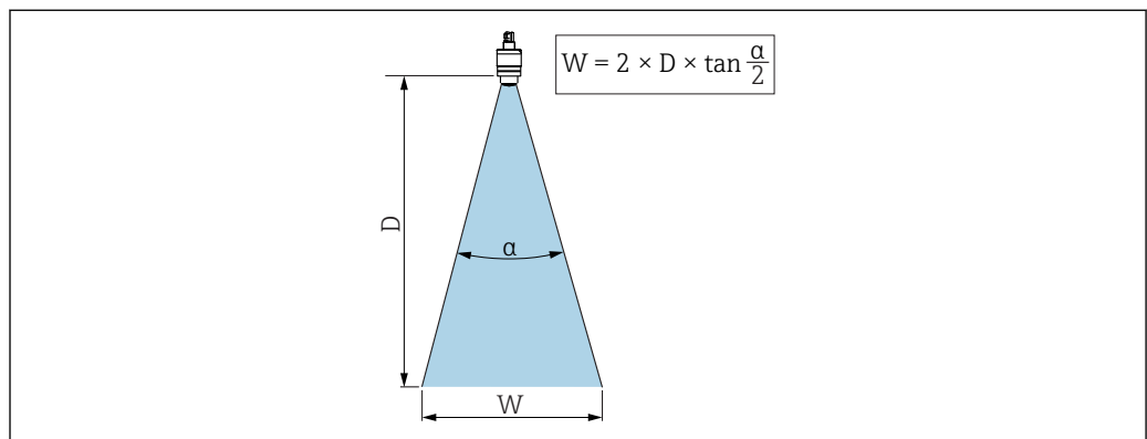
图 14 波束角 α、距离 D 和波束宽度 W 的相互关系
