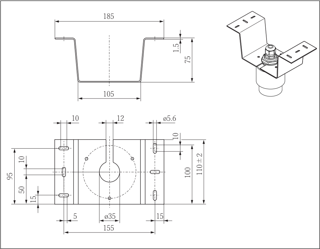
56 罐顶安装架的外形尺寸；单位：mm (in)
