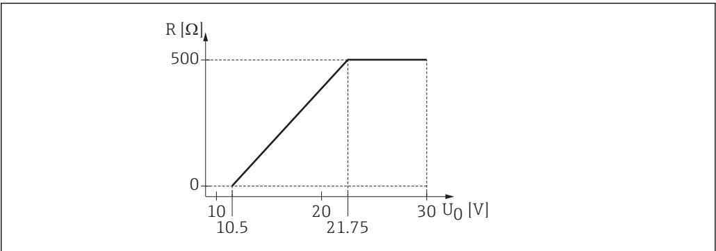
3 最大负载 R，取决于电源的供电电压 U 0
