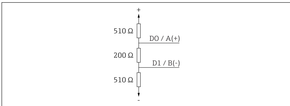
図 18 RS485-IS 仕様準拠するバス終端抵抗の図示
