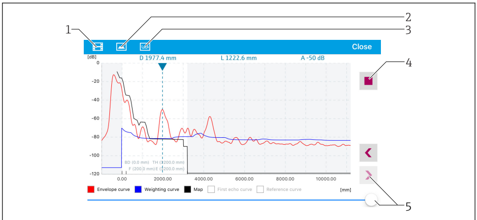
図 23 SmartBlue (iOS 版) での反射波形表示 (例)
