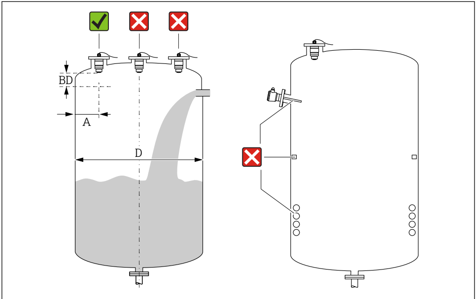
図 5 容器内の設置位置
