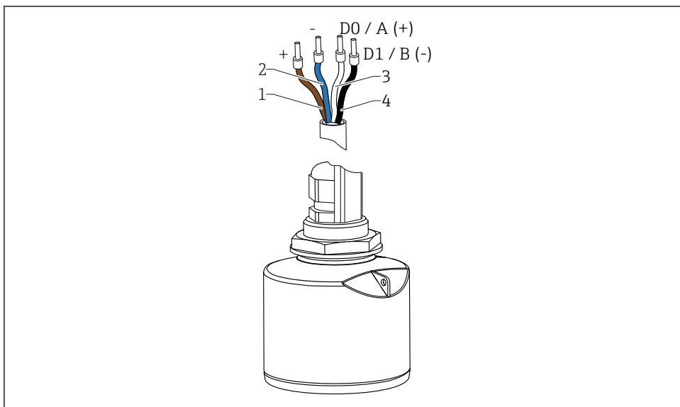
図 15 FMR20 ケーブルの割当て、Modbus
