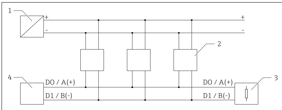
図 17 Modbus RS485 接続、複数ユーザーのブロック回路図
