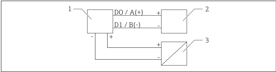
図 16 Modbus RS485 接続のブロック回路図
