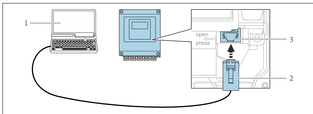
24 Подключение через служебный интерфейс (CDI-RJ45)
