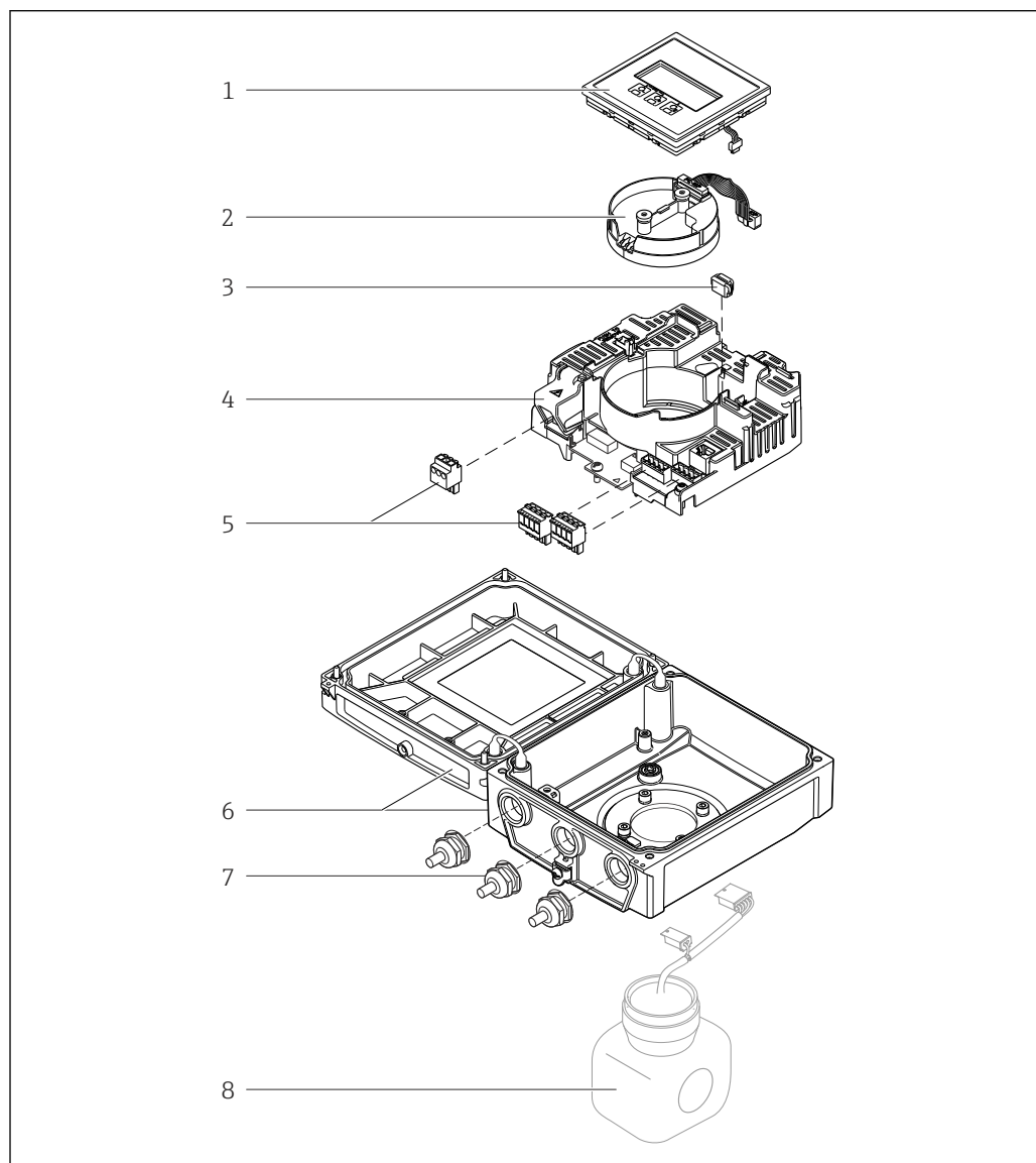
1 Важные компоненты прибора в компактном исполнении
