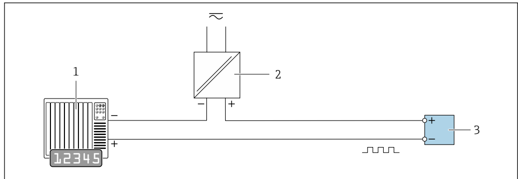
19 Пример подключения для импульсного/частотного выхода (пассивного)
