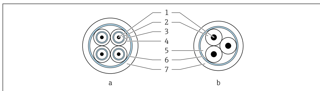
10 Поперечное сечение кабеля
