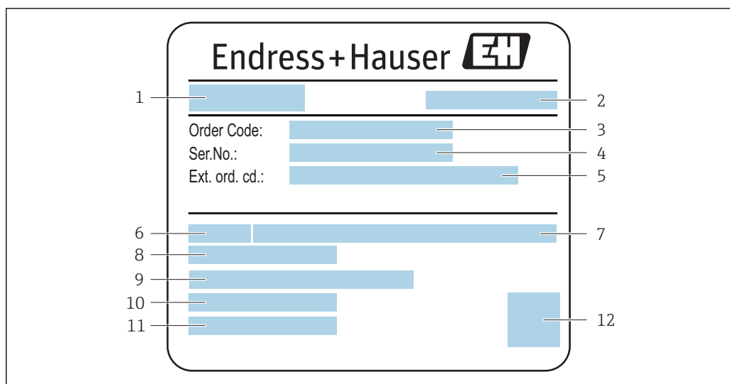
3 Пример заводской таблички сенсора
