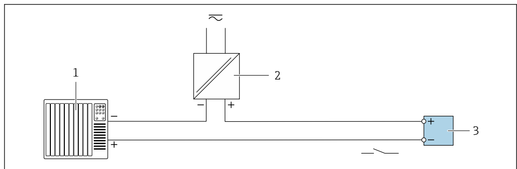
20 Пример подключения для релейного выхода (пассивного)
