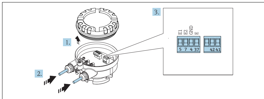
14 Сенсор: клеммный блок
