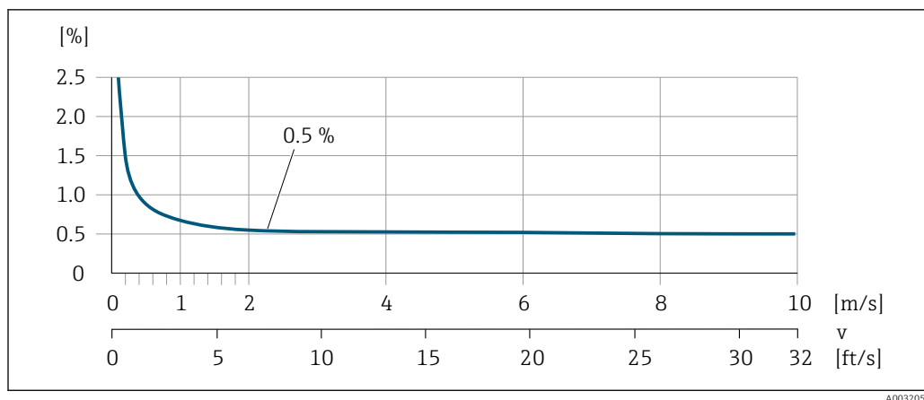
33 Максимальная погрешность измерения в % ИЗМ
