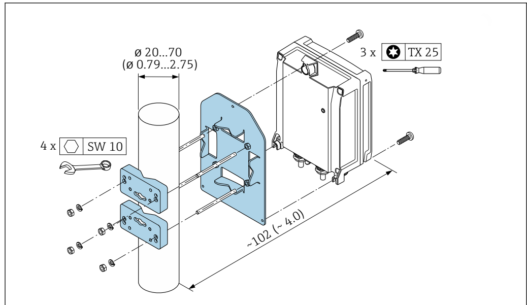
9 Единица измерения, мм (дюйм)
