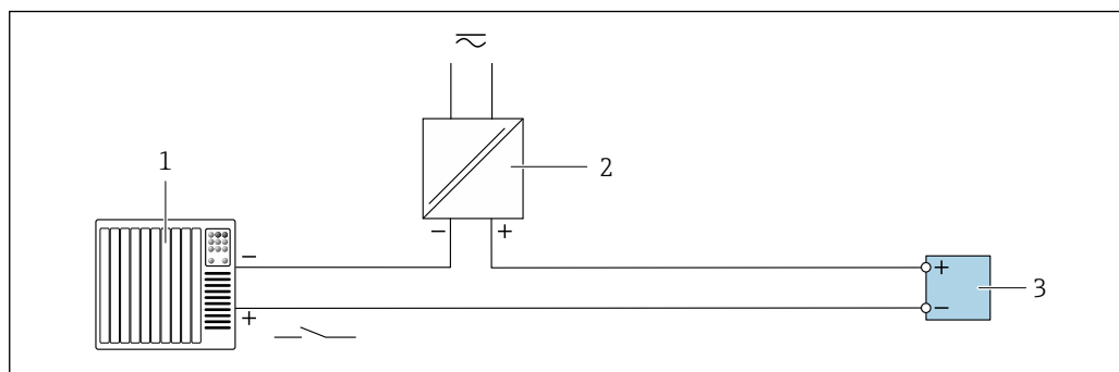
30 Пример подключения для входного сигнала состояния
