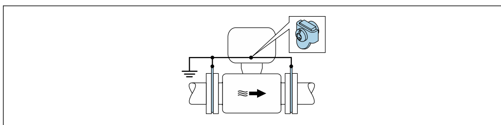
22 Выравнивание потенциалов с помощью заземляющей клеммы и заземляющих дисков
