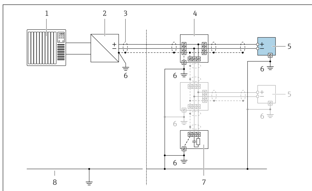
17 Пример подключения для FOUNDATION Fieldbus
