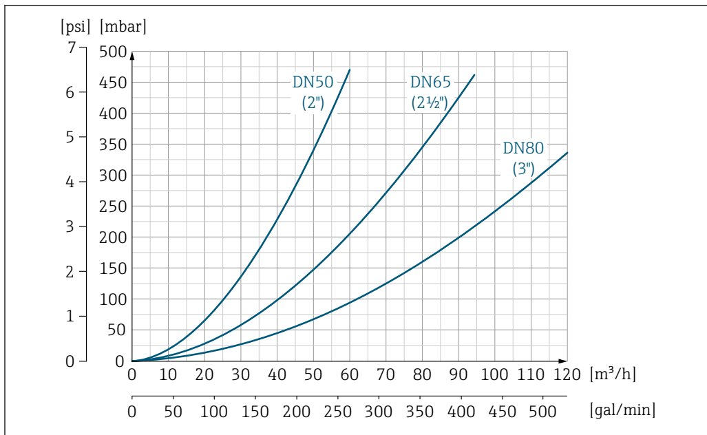
47 Падение давления DN 50–80 (2–3 дюйма) с кодом заказа для параметра «Конструкция», опция С, «Фиксированный фланец, без входных/выходных участков»
