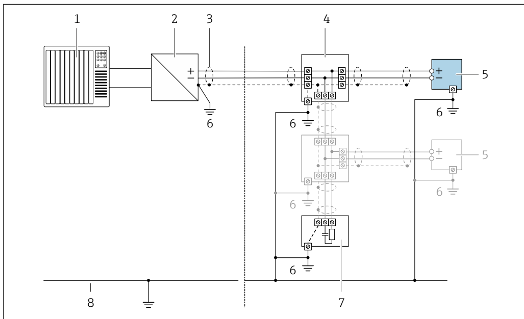
23 Пример подключения для FOUNDATION Fieldbus
