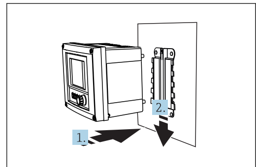
23 Dopasowanie przyrządu do płyty montażowej i zatraskowanie we właściwym miejscu
