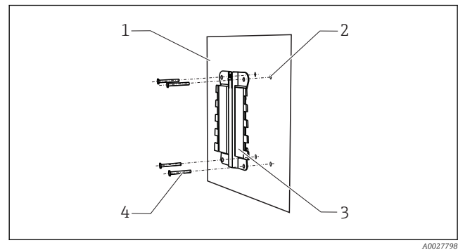
21 Montaż do ściany
