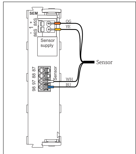
46 Podłączenie fotometru do modułu SEM
