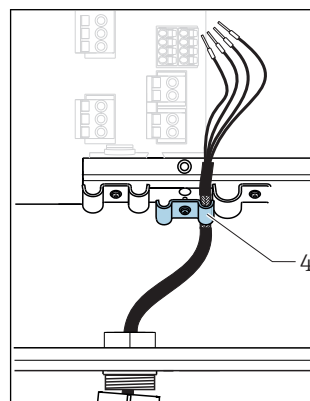
36 Wprowadzanie przewodu
