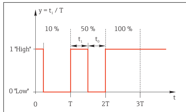
82 Typowe zastosowanie: elektrozawór
