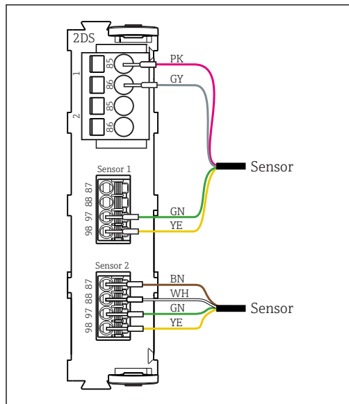
45 Podłączenie czujników Memosens z dodatkowym zasilaniem lub bez dodatkowego zasilania do modułu 2DS
