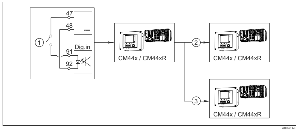
85 Przykład centralnego sterowania czyszczeniem
