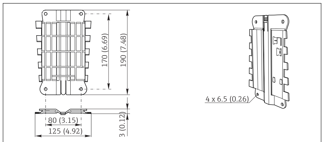
8 Płyta montażowa, wymiary w mm (calach)
