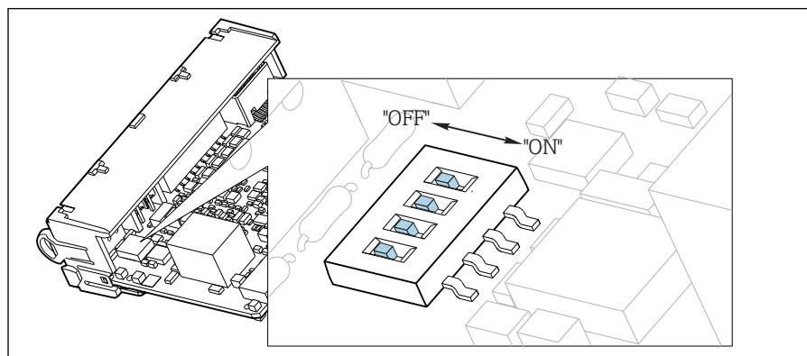
73 Mikroprzełączniki do wewnętrznej terminacji magistrali
