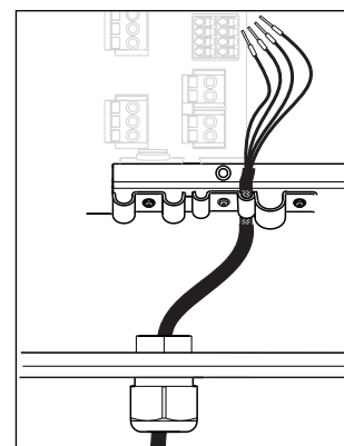
37 Dokręcanie śruby (2 Nm)
