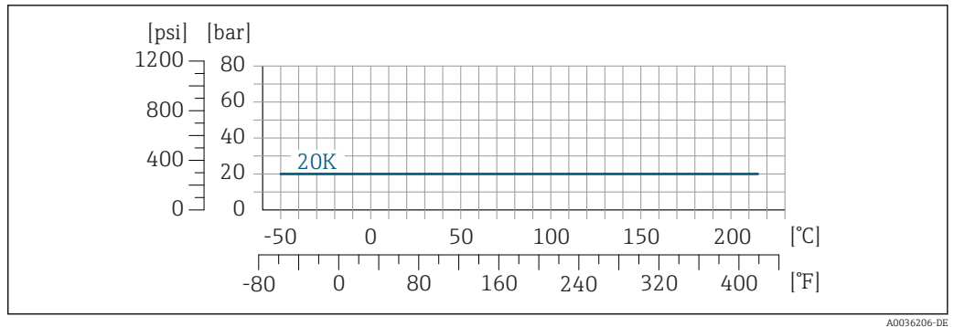
21 Losflansch mit Flanschwerkstoff: 1.4301 (F304), mediumsberührende Teile Alloy C22: 2.4602 (UNS N06022)
