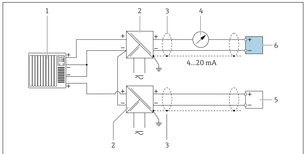
12 Anschlussbeispiel für HART-Eingang mit gemeinsamem "Minus" (passiv)
