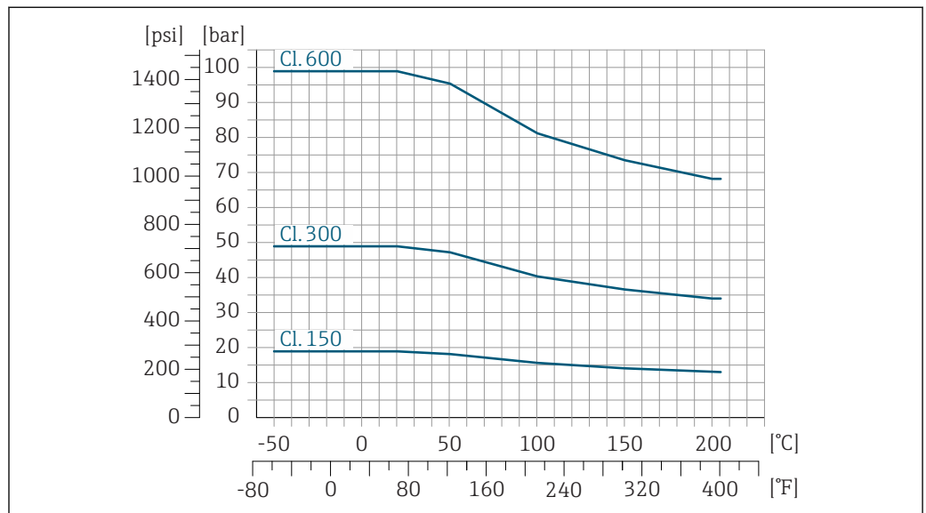
19 Losflansch mit Flanschwerkstoff: 1.4301 (F304), mediumsberührende Teile Alloy C22: 2.4602 (UNS N06022)
