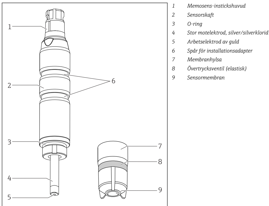
1 Sensors konstruktion
