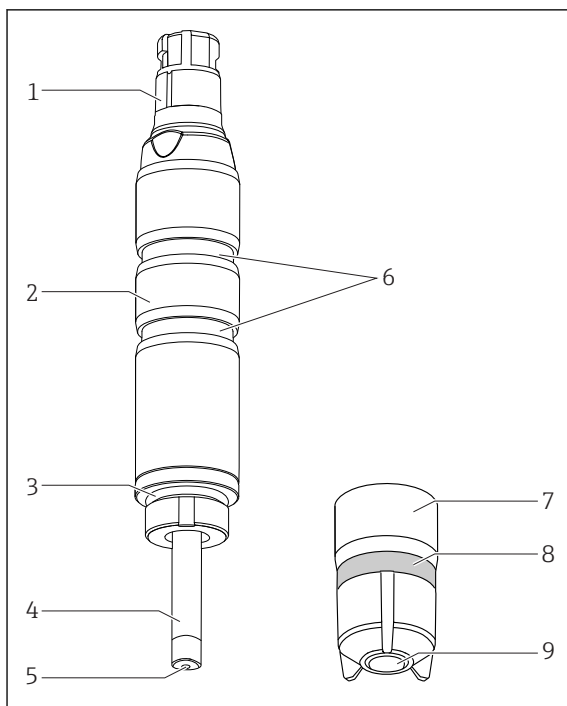
1 Sensorens opbygning
