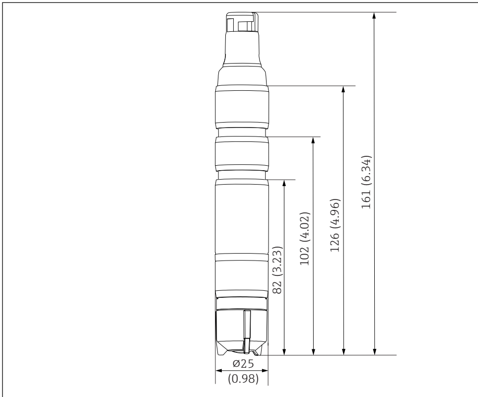
3 Méretek mm-ben (inch)
