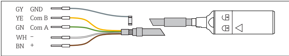
12 CYK10 /CYK20 mérőkábel
