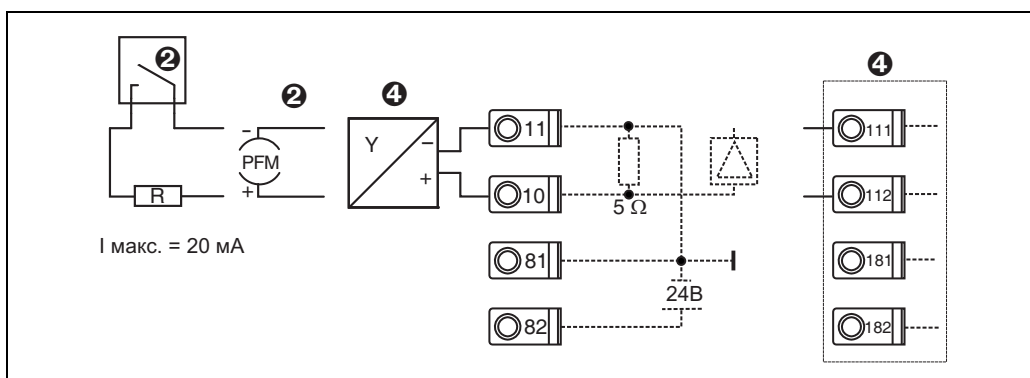
Рис. 7: Подключение активного датчика, напр. к входу 1 (Слот А I).
