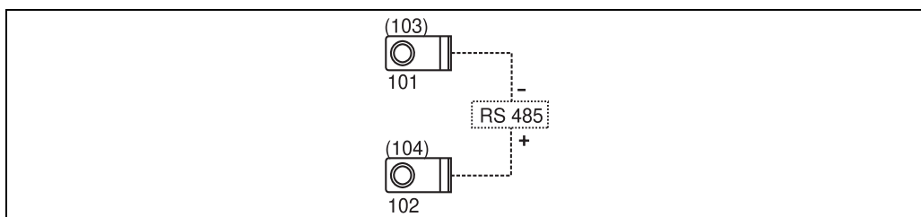
Рис. 11: Подключение интерфейса
