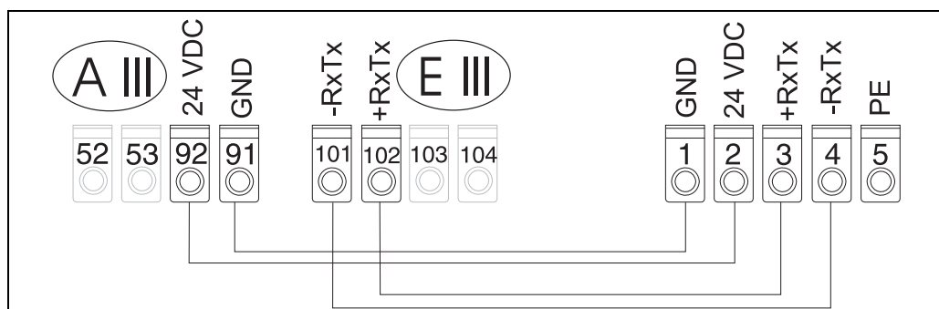
Рис. 14: Назначение клемм для подключения вынесенного дисплея/устройства управления
