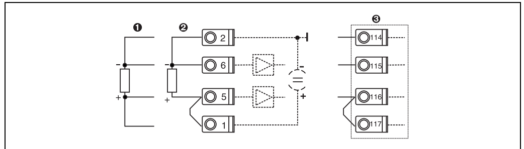
Рис. 9: Подключение датчика температуры, напр. к входу 1 (слот E I)
