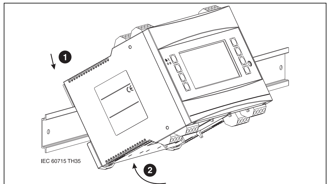
Рис. 3: Монтаж прибора на монтажной рейке
