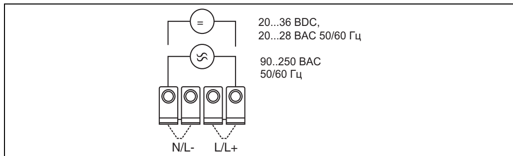
Рис. 6: Подключение электропитания
