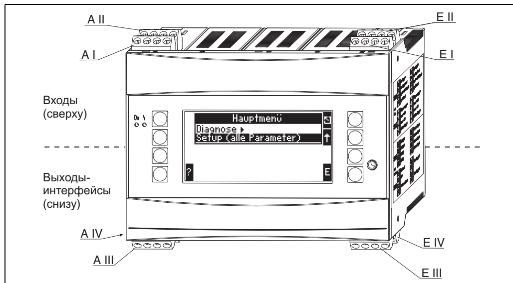
Рис. 5: Расположение слотов (стандартное исполнение)
