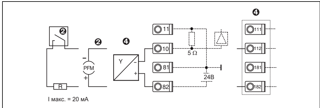
Рис. 8: Подключение пассивного датчика, напр. к входу 1 (слот A I).
