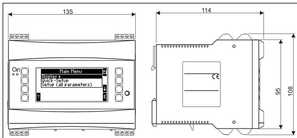
Рис. 25: Корпус для монтажа на шину по IEC 60715; размеры даны в мм
