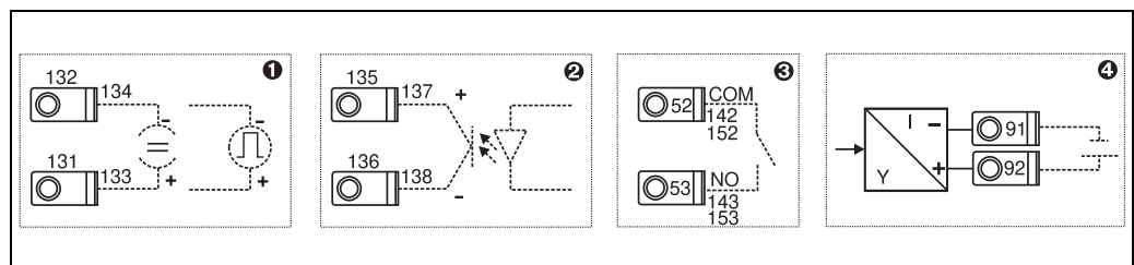
Рис. 10: Подключение выходов
