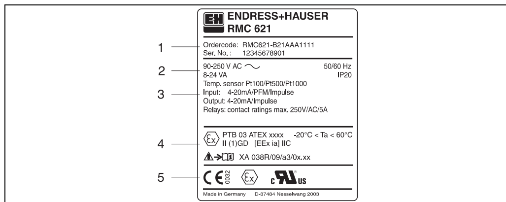
Рис. 2: Шильда контроллера (пример)
