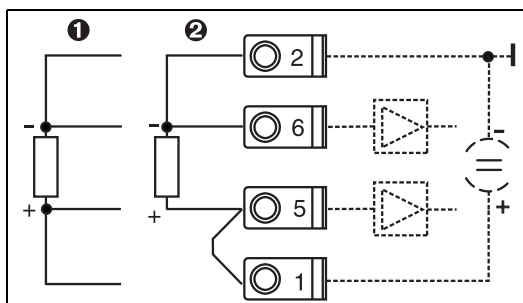
Рис. 1: Подключение датчика температуры, напр., к входу 1 (слот E1)
