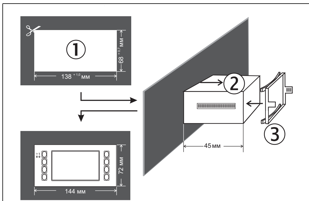
Рис. 13: Монтаж в панели
