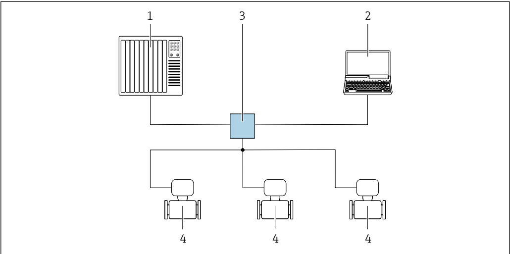
图 22 通过 PROFINET 网络实现远程操作：星形拓扑结构
