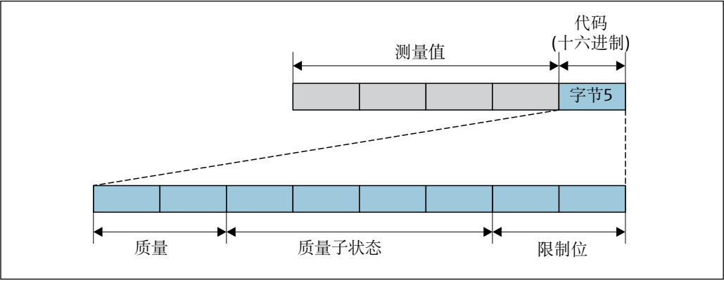
图 28 状态字节的结构
