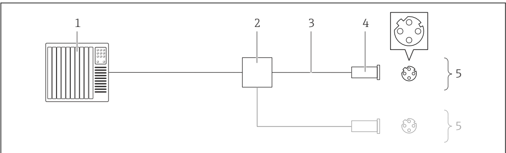
图 10 PROFINET 的连接示例
