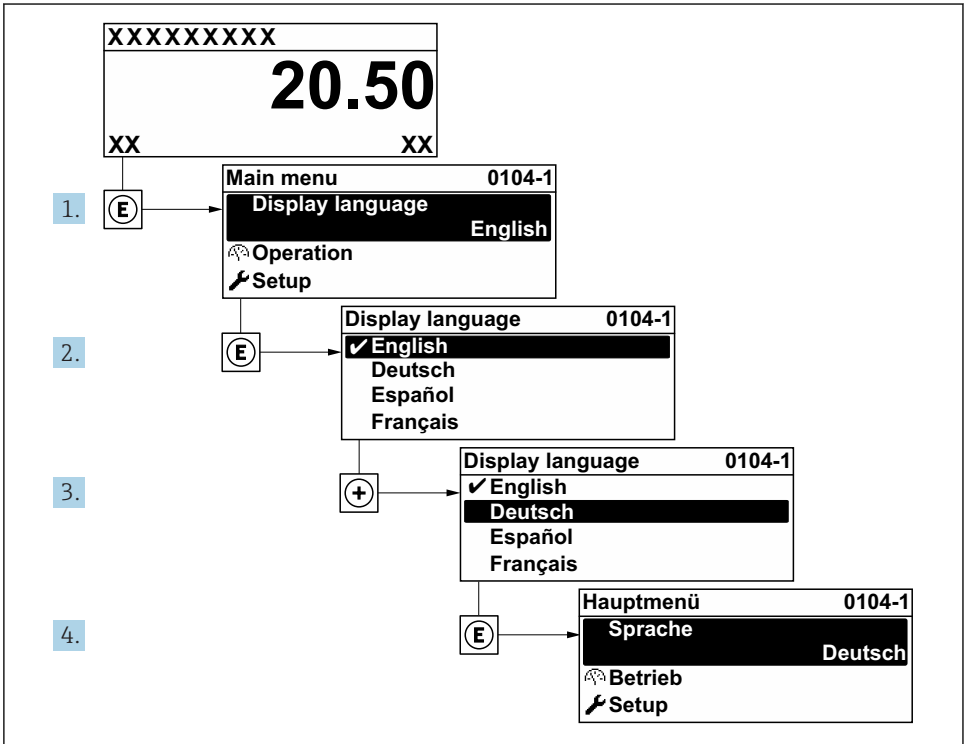
2 로컬 디스플레이의 예 사용
