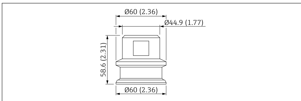
图 16 G 1"焊座，带螺纹套筒。测量单位 mm (in)
