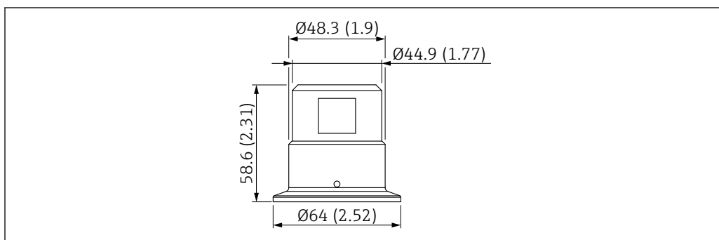
图 17 G 1"过程转接头，Tri-Clamp 2"卡箍，安装有螺纹套筒。测量单位 mm (in)
