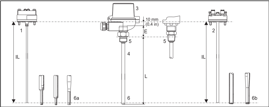
Architecture de l'appareil Omnigrad M TR11
