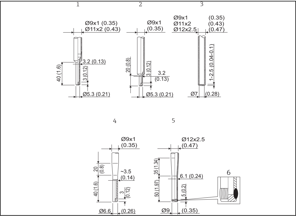
Versions d'extrémités de protecteur disponibles (rétreinte, droite, conique). Rugosité de surface maximale ≤ Ra 0,8 µm (31.5 µin)
