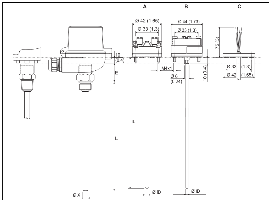
Dimensions de l'Omnigrad M TR11
