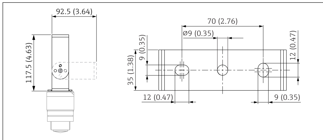
40 Dimensioni della staffa di montaggio, unità ingegneristica: mm (in)
