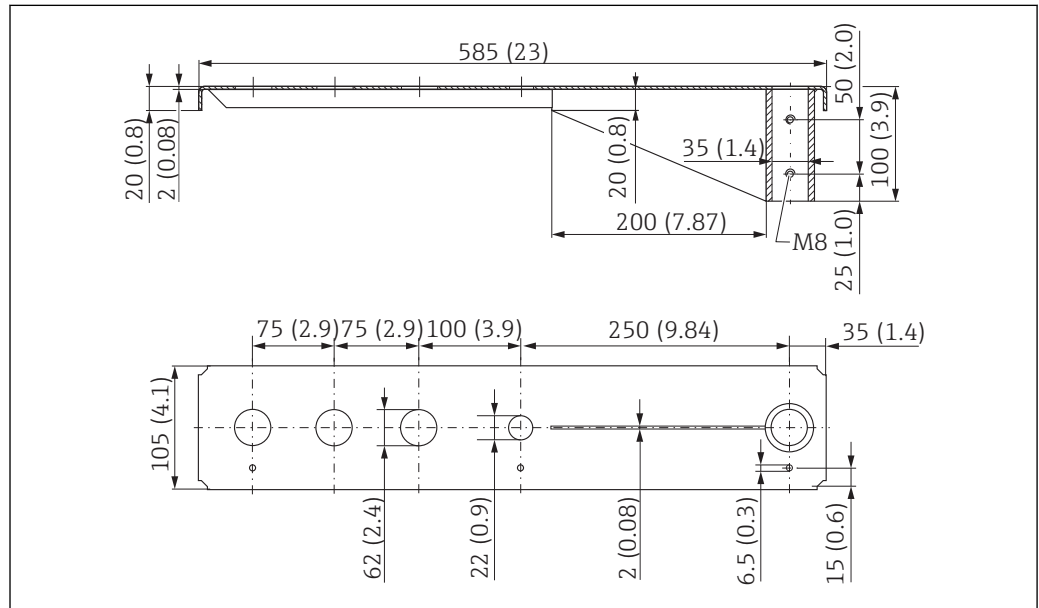
51 Dimensioni della trave a mensola (corta) con cardine per la connessione al processo del sensore G 2" su fronte. Unità di misura mm (in)
