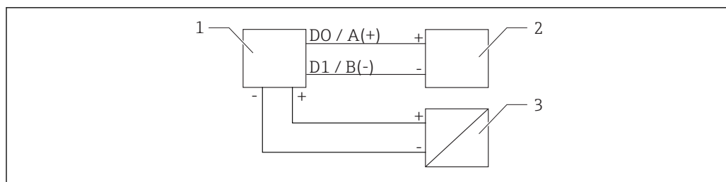
6 Schema a blocchi del circuito per la connessione Modbus RS485
