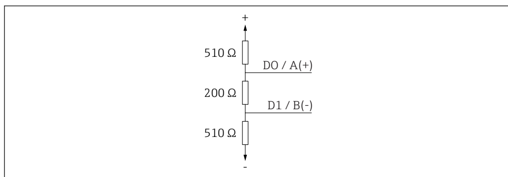
8 Rappresentazione della resistenza di terminazione del bus secondo le specifiche RS485-IS
