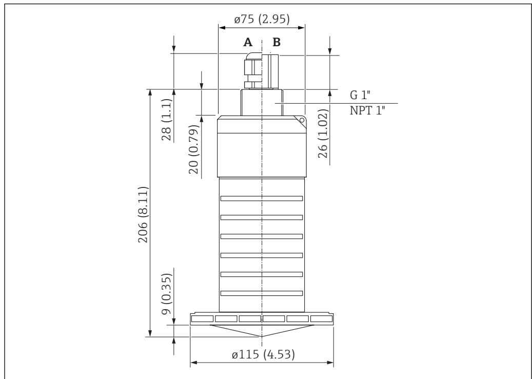
■ 26 Dimensioni dell'antenna da 80 mm (3 in); unità ingegneristica: mm (in)
