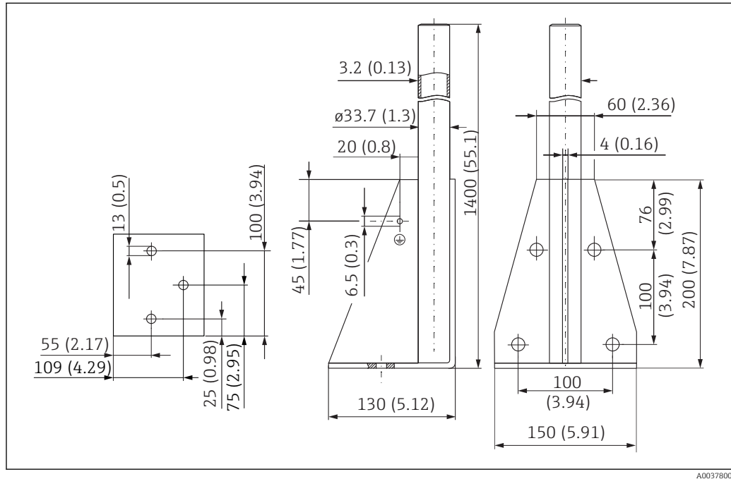
54 Dimensioni del telaio di montaggio (lungo). Unità di misura mm (in)
