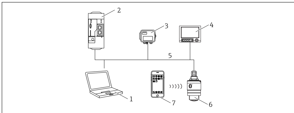
34 Opzioni per il funzionamento a distanza mediante protocollo Modbus
