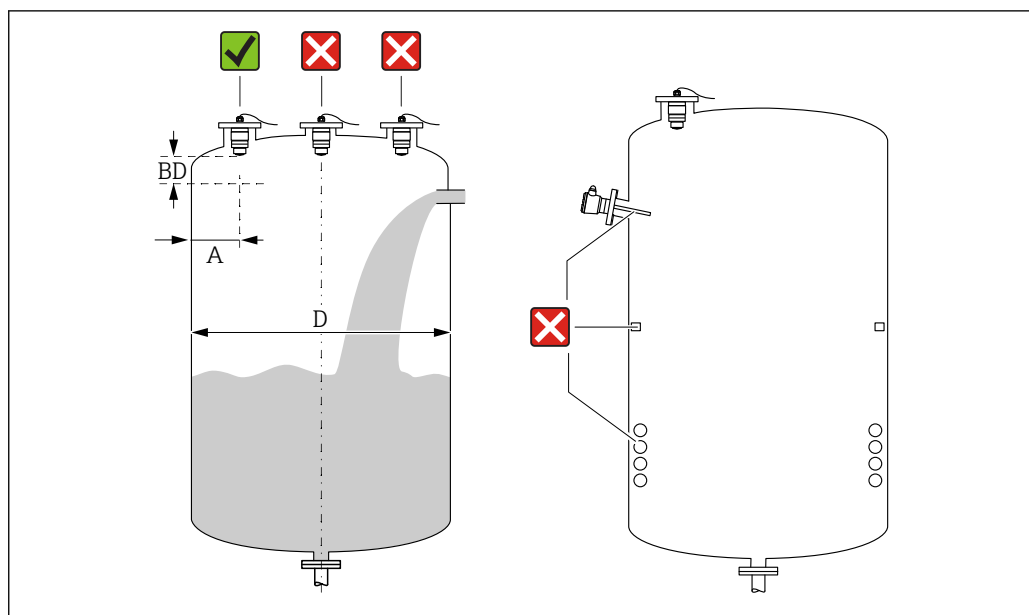
11 Posizione di installazione su un silo
