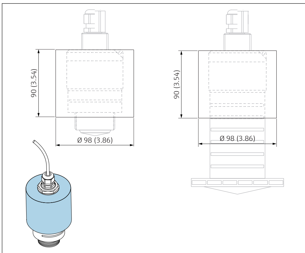
35 Dimensioni del coperchio di protezione; unità ingegneristica: mm (in)
