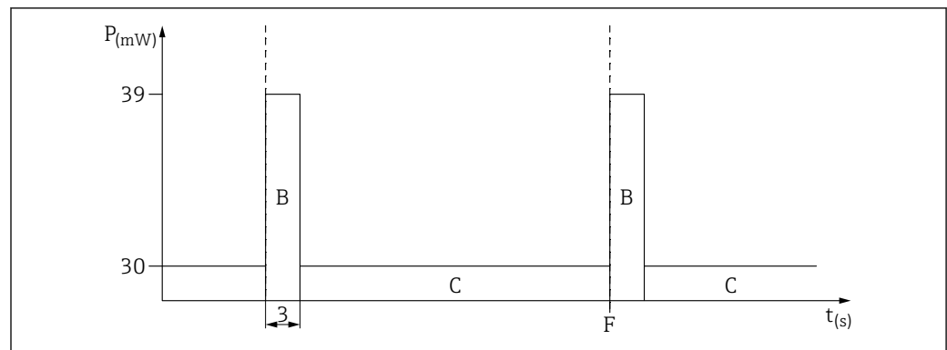
4 Consumo di energia in modalità single shot sempre attivata
