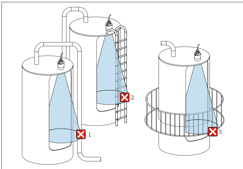
15 Misura in un recipiente di plastica con un'installazione metallica che interferisce all'esterno del recipiente
