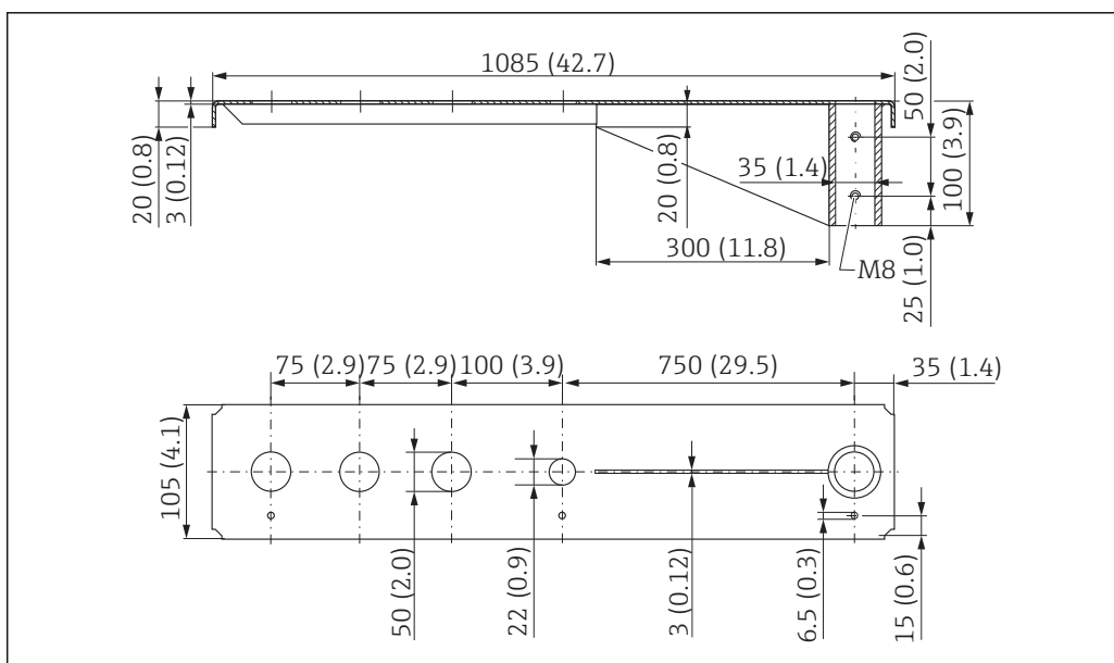
50 Dimensioni della trave a mensola (lunga) con cardine per connessione al processo del sensore G 1-½" sul lato anteriore. Unità di misura mm (in)
