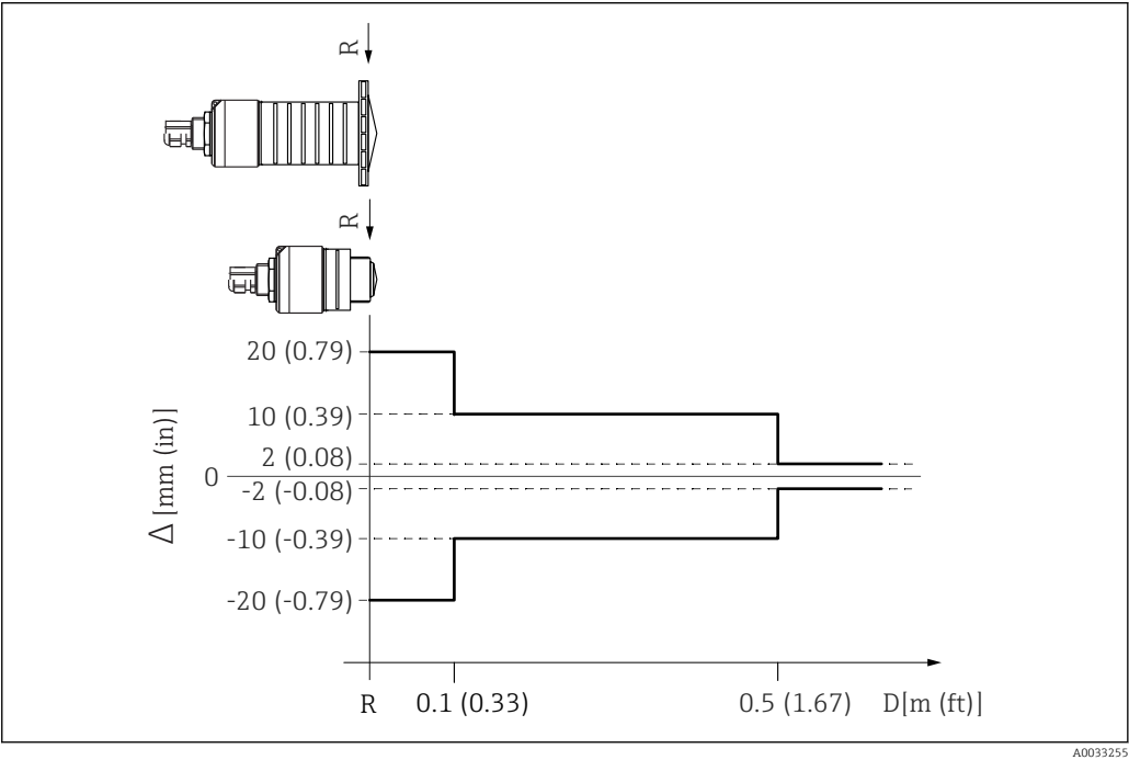
9 Errore di misura massimo in applicazioni nelle vicinanze dell'emissione; valori per versione standard Δ Errore di misura massimo R Punto di riferimento della misura di distanza D Distanza dal punto di riferimento dell'antenna
