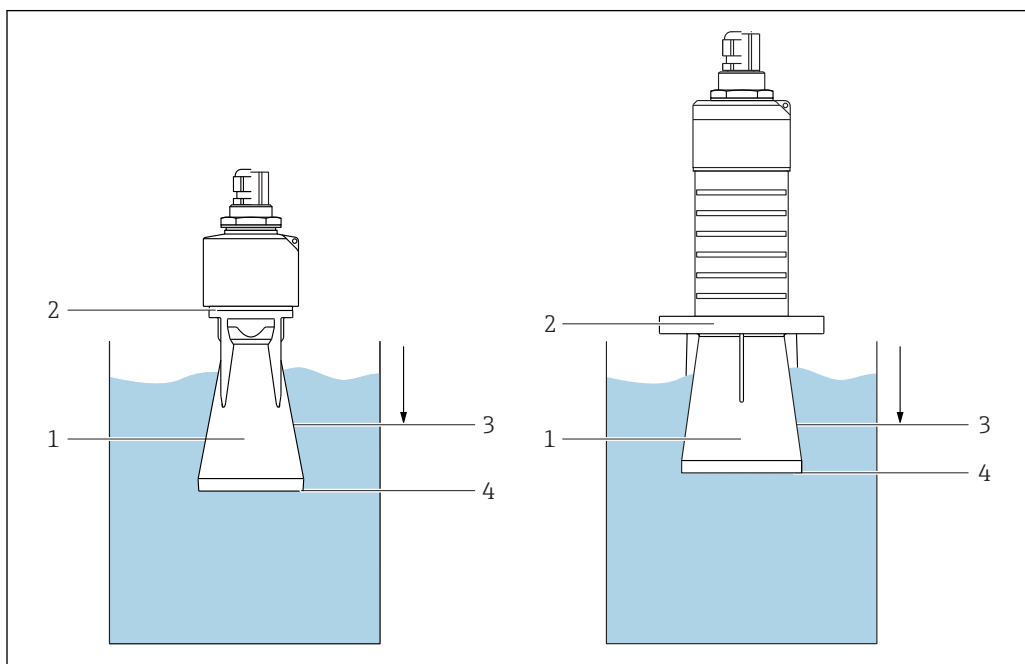
17 Funzione del tubo di protezione da allagamento
