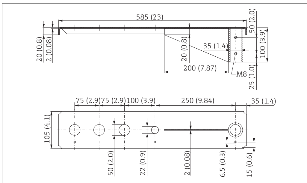
49 Dimensioni della trave a mensola (corta) con cardine per connessione al processo del sensore G 1-½" sul lato anteriore. Unità di misura mm (in)
