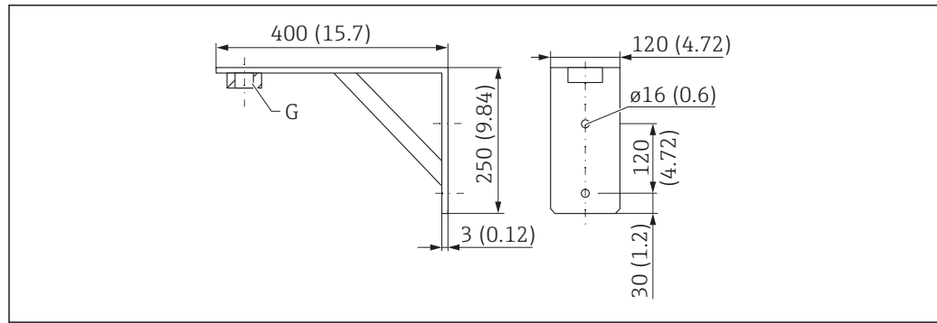
44 Dimensioni della staffa ad angolo. Unità di misura mm (in)
