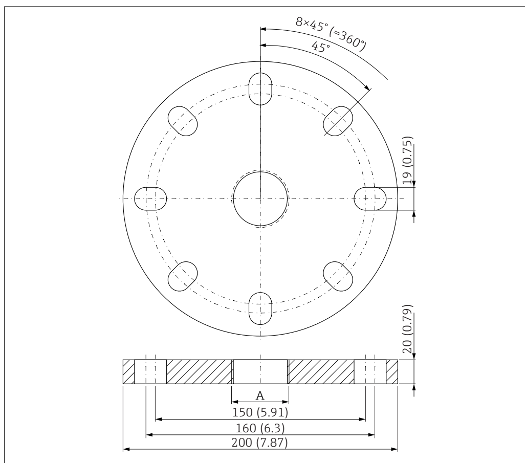
42 Dimensioni della flangia UNI 3"/DN80/80, unità ingegneristica: mm (in)
