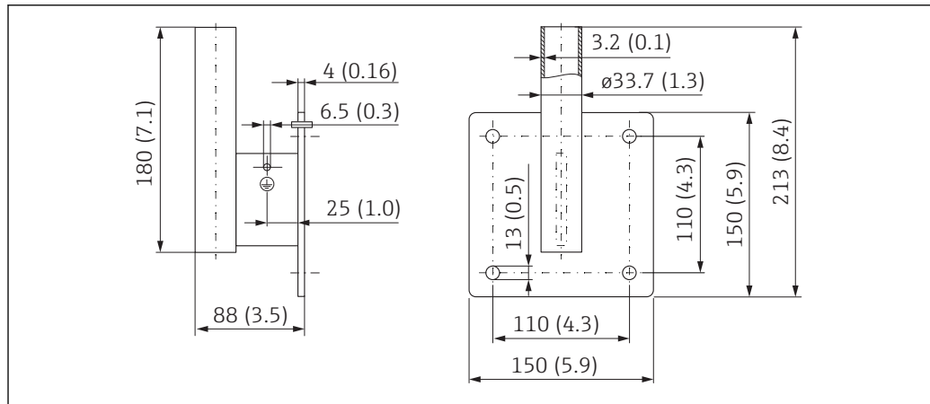
55 Dimensioni della staffa a parete. Unità di misura mm (in)
