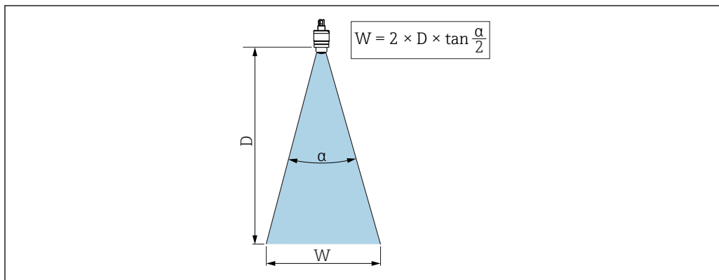
14 Rapporto tra angolo di emissione \alpha , distanza D e diametro del lobo di emissione W
