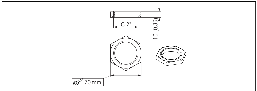
37 Dimensioni del dado di fissaggio, unità ingegneristica: mm (in)
