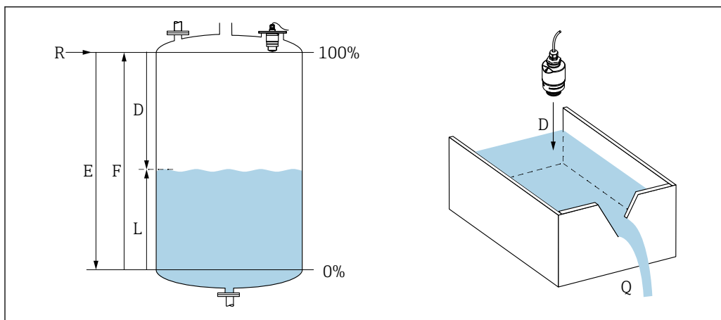
1 Parametro di taratura livello / portata
