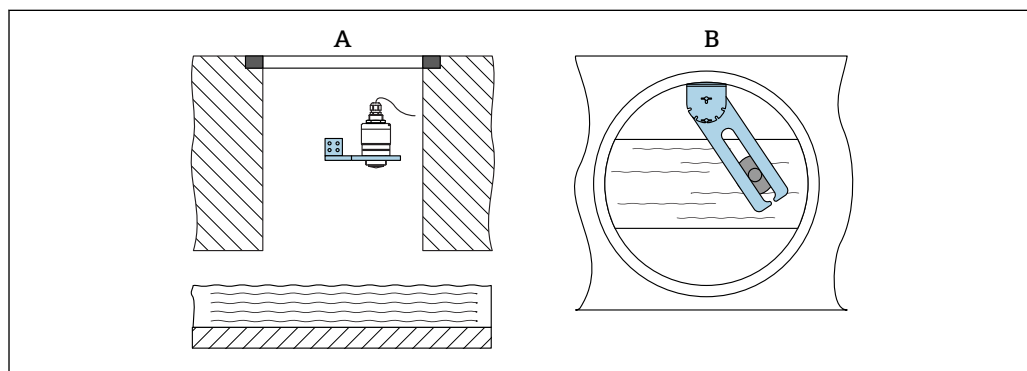
21 Montaggio in un pozzetto, orientabile e regolabile
