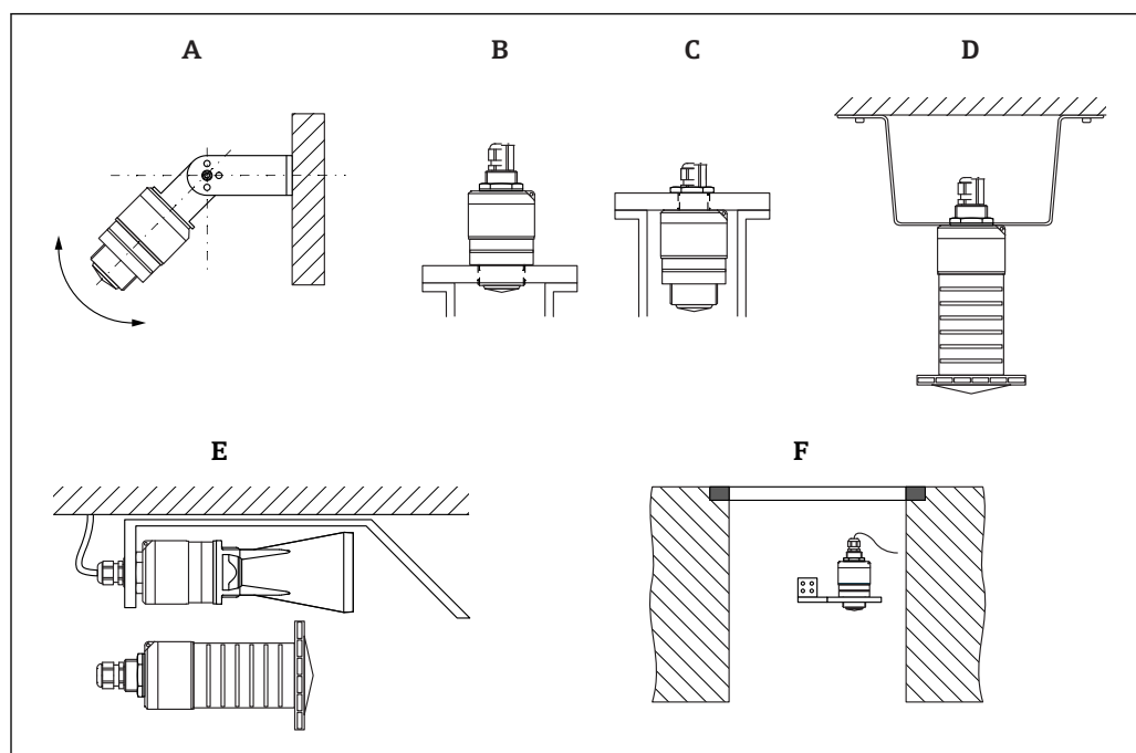
10 Installazione a parete, soletta o su trinchetto
