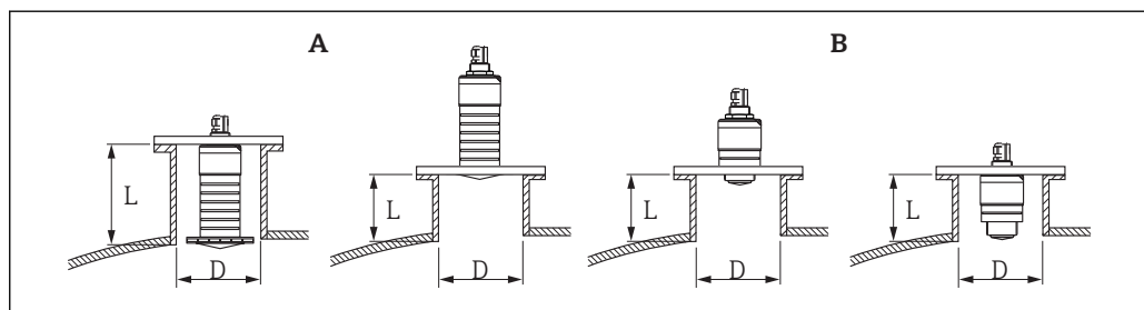
12 Installazione su tronchetto
