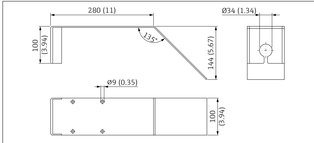
58 Dimensioni staffa di montaggio orizzontale per pozzetti per fognatura. Unità di misura mm (in)
