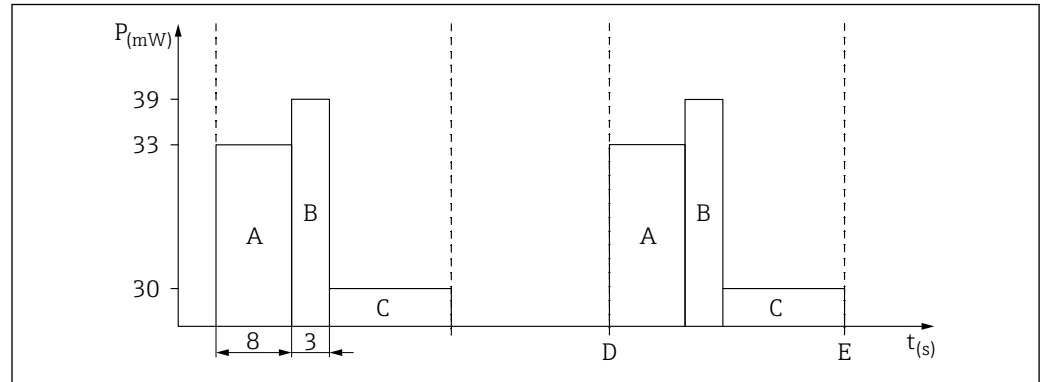
3 Consumo di energia in modalità single shot attivata/disattivata mediante RTU
