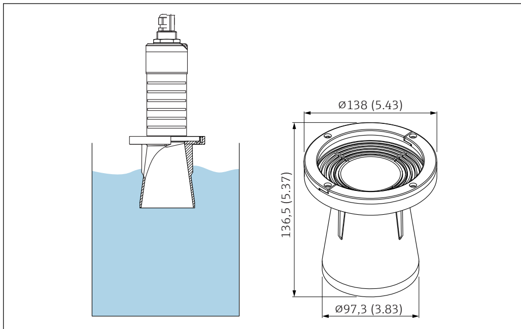
39 Dimensioni del tubo di protezione da allagamento 80 mm (3 in); unità ingegneristica: mm (in)
