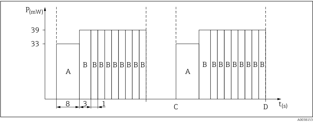
5 Consumo di energia in modalità di misura continua attivata/disattivata mediante RTU
