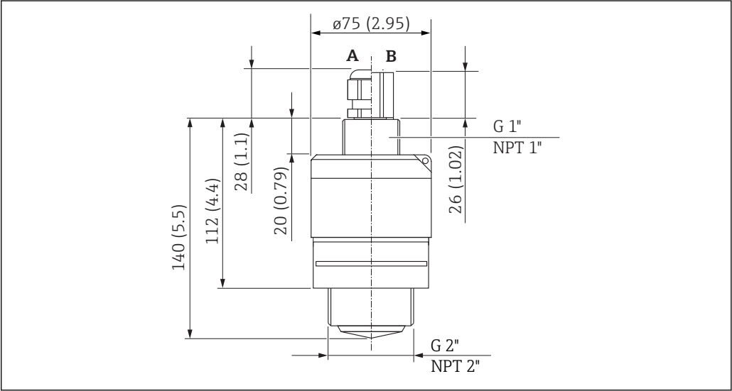
24 Dimensioni della filettatura della connessione al processo G 2" o MNPT 2", unità ingegneristica: mm (in)
