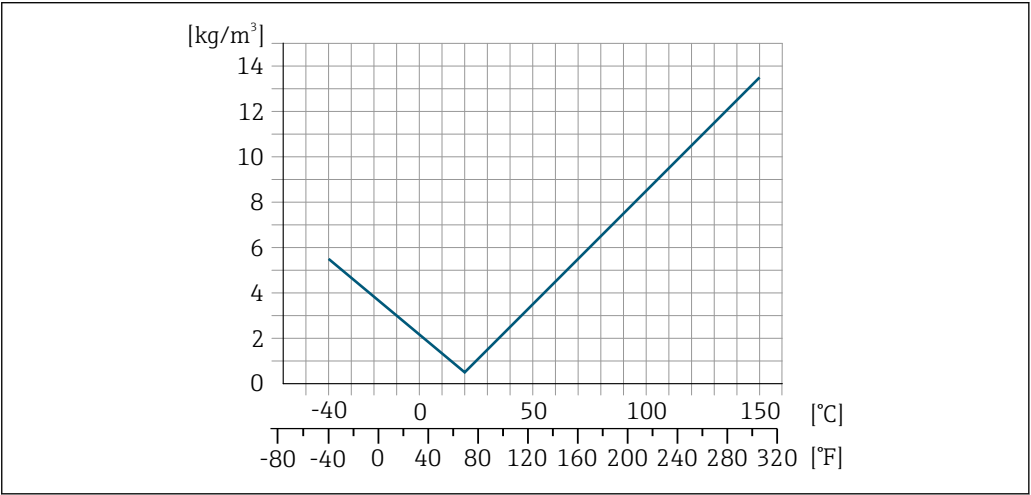
33 Calibración de densidad de campo, por ejemplo a +20 °C (+68 °F)
