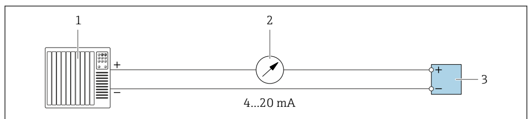
Fig. 12 Ejemplo de conexión de salida de corriente de 4-20 mA (activa)
