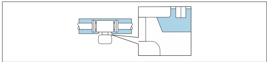
7 Aislamiento térmico con cuello extendido al aire libre
