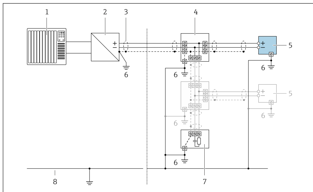
9 Ejemplo de conexión de PROFIBUS PA
