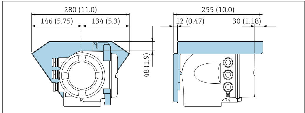
図 9 Proline 500 用の保護カバー、単位 mm (in)
