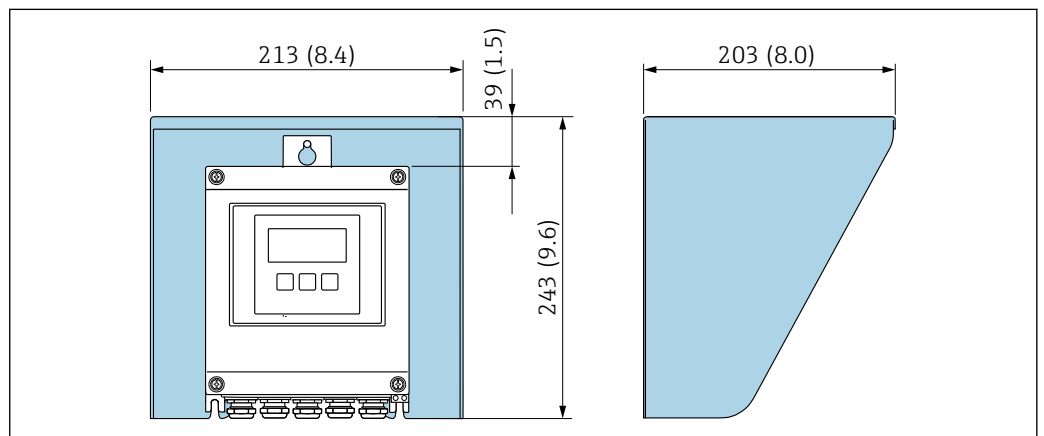
8 Proline 500 – デジタル用の保護カバー、単位 mm (in)
