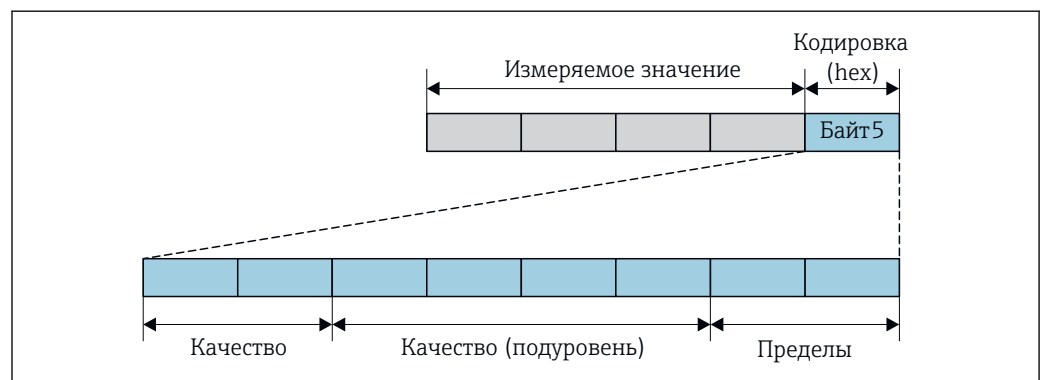
28 Структура байта кодирования
