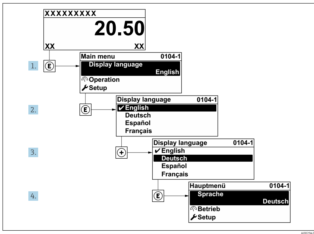
23 Пример индикации на локальном дисплее
