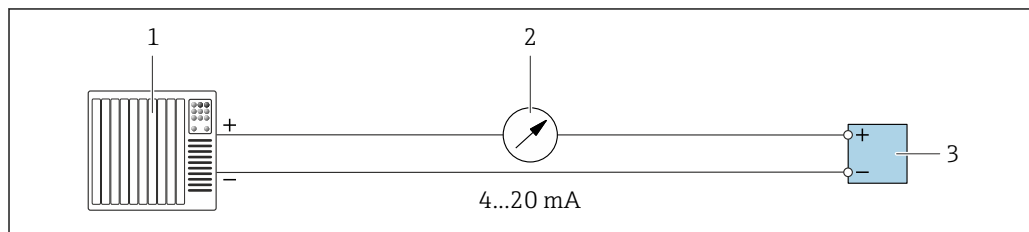
10 Пример подключения для токового выхода 4–20 мА (активного)
