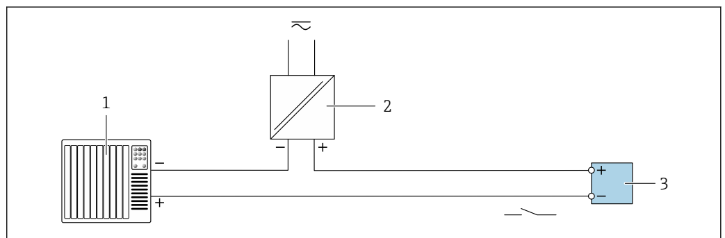
■ 16 リレー出力（パッシブ）の接続例
