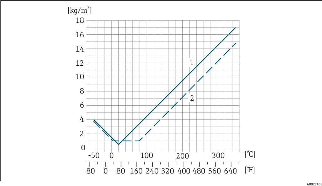
1 現場密度校正、例：+20 °C (+68 °F) 時 2 高精度密度校正
