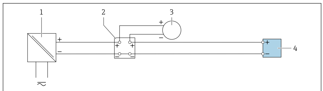
17 4~20 mA 電流入力の接続例
