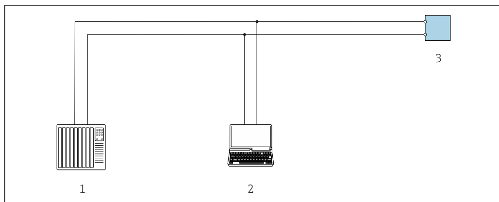
図 23 Modbus-RS485 プロトコル経由のリモート操作オプション（アクティブ）
