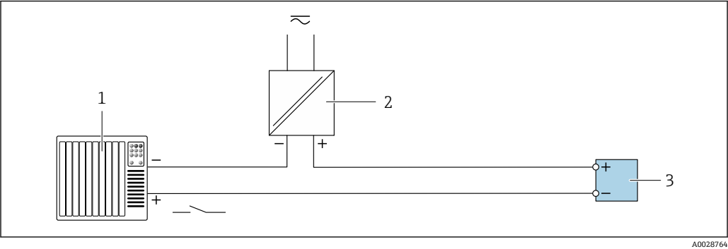
図 18 ステータス入力の接続例 1 オートメーションシステム、ステータス出力付き（例：PLC） 2 電源 3 変換器
