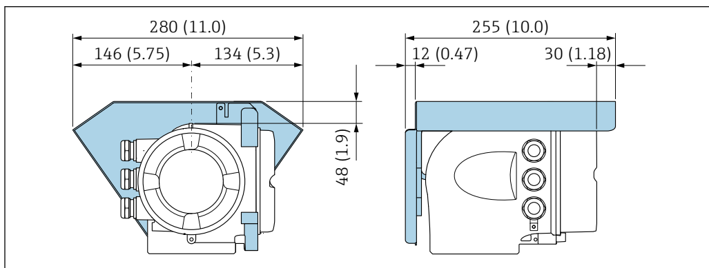
7 Единица измерения – мм (дюйм)
