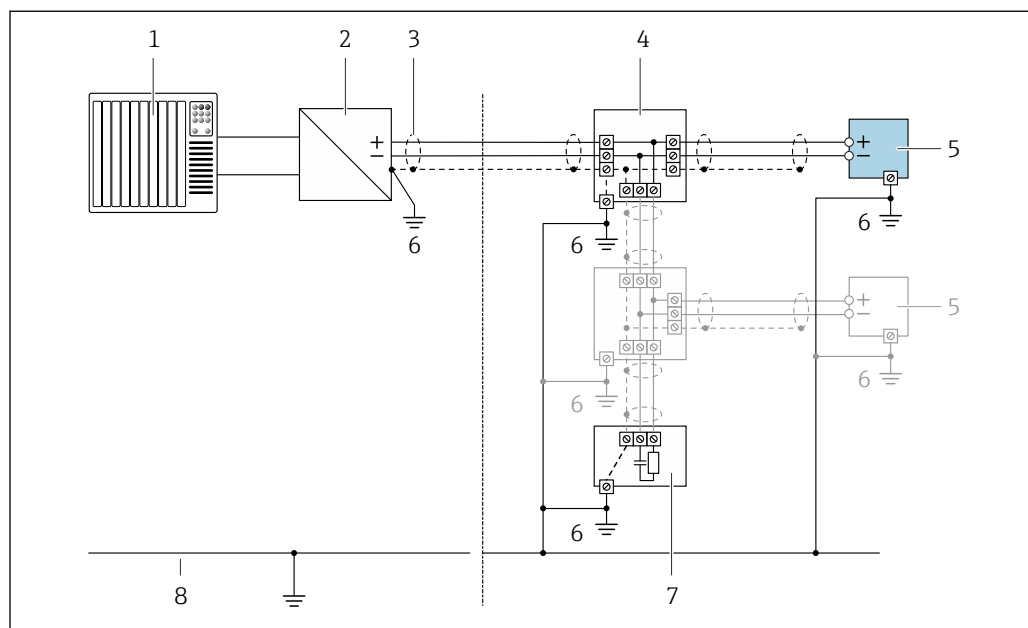
8 Пример подключения для PROFIBUS PA
