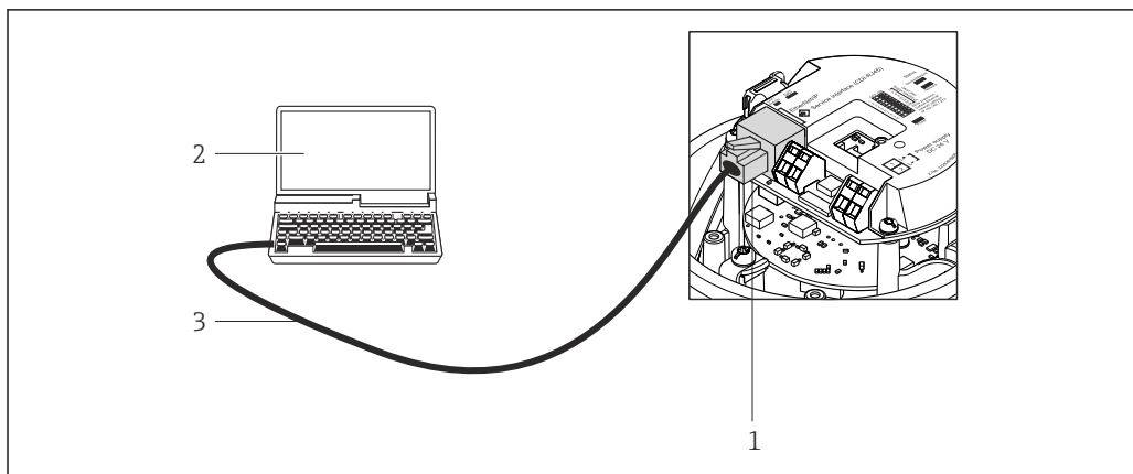
16 Подключение для кода заказа "Выход", опция L: PROFIBUS DP
