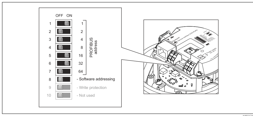
12 Назначение адресов с помощью DIP-переключателей на электронном модуле входа/выхода
