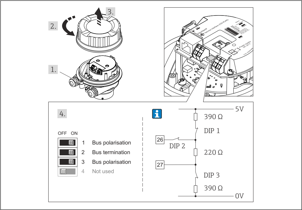
13 Терминирование с помощью DIP-переключателей на электронном модуле ввода/вывода (для скоростей передач < 1,5 Мбод)
