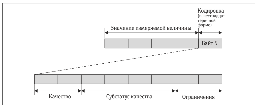
18 Структура кодирующего байта
