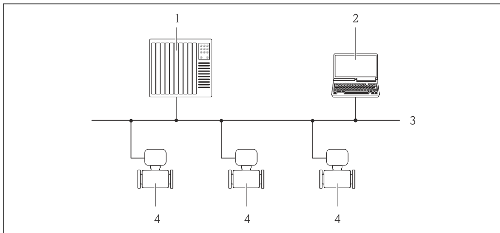
15 Варианты дистанционного управления через сеть PROFIBUS DP
