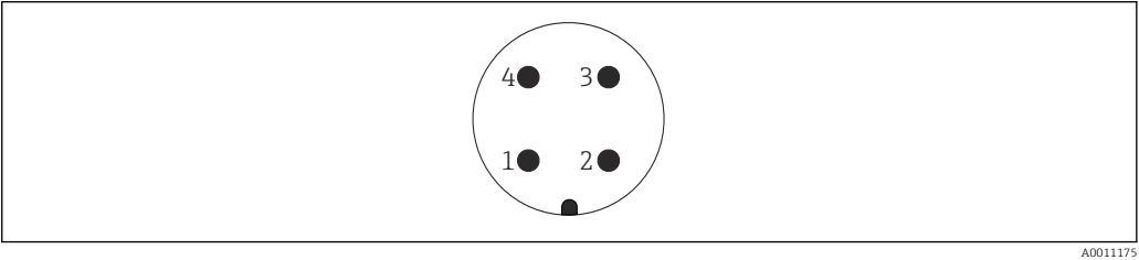
1 Signal + 2 Libre 3 Signal - 4 Terre/fil de terre
