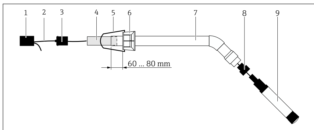
9 Nedsænkingskonstruktion CYA112 med monteret sensor
