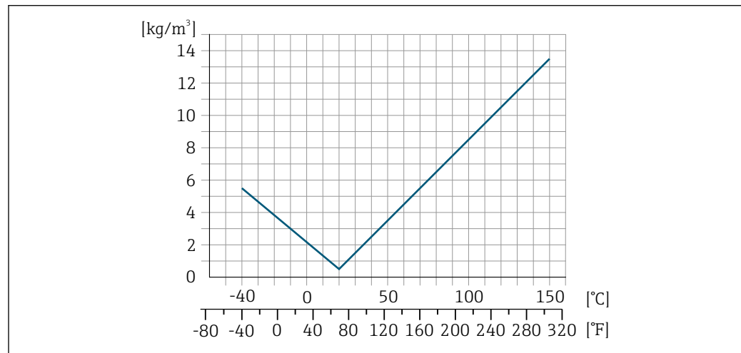
37 Kalibracja gęstości w warunkach procesowych, np. w temperaturze +20°C (+68°F)
