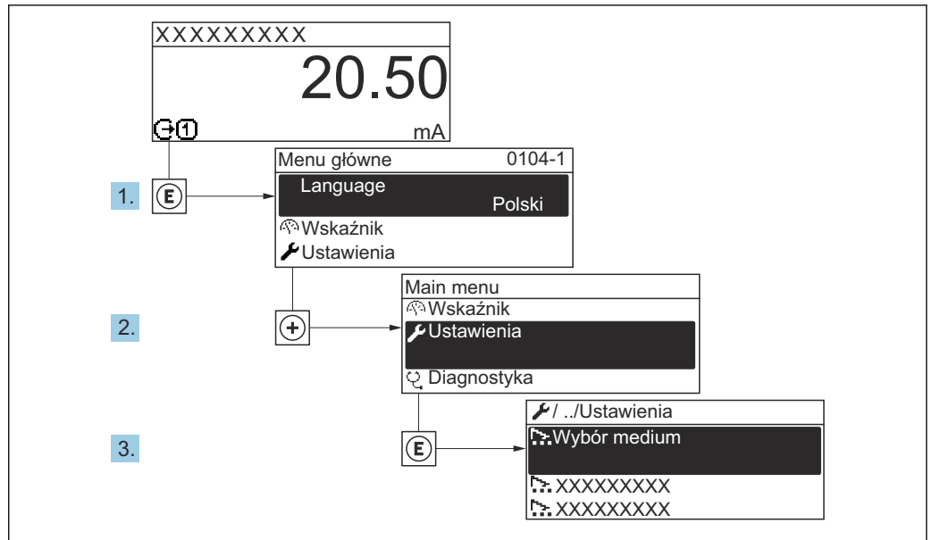
29 Przykład menu na wyświetlaczu lokalnym
