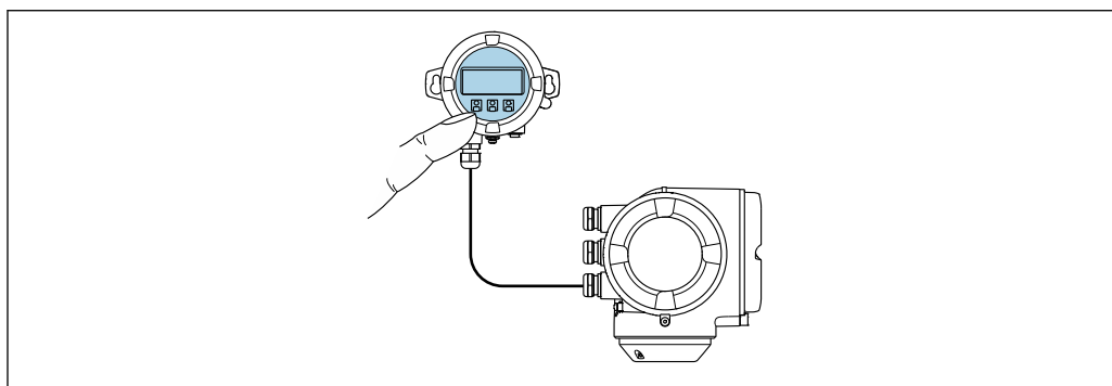
39 Obsługa za pomocą zewnętrznego wskaźnika DKX001
