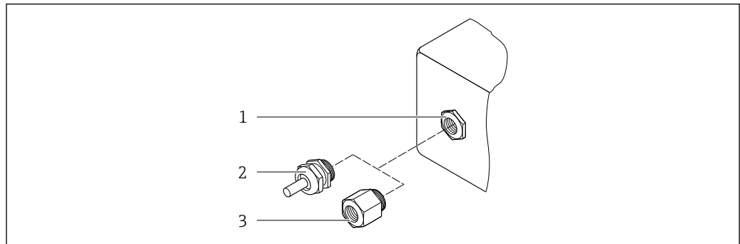
37 Możliwe wprowadzenia przewodów/dławiki kablowe
