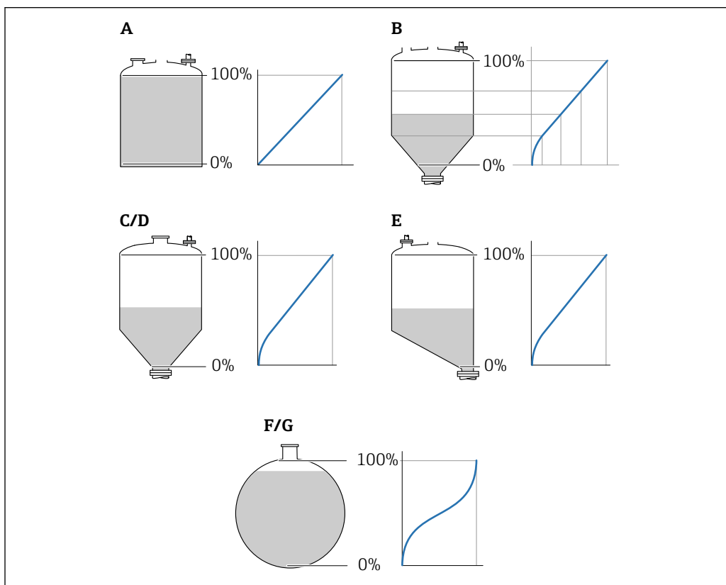
52 Типы линеаризации
