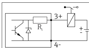
20 Подключение реле
