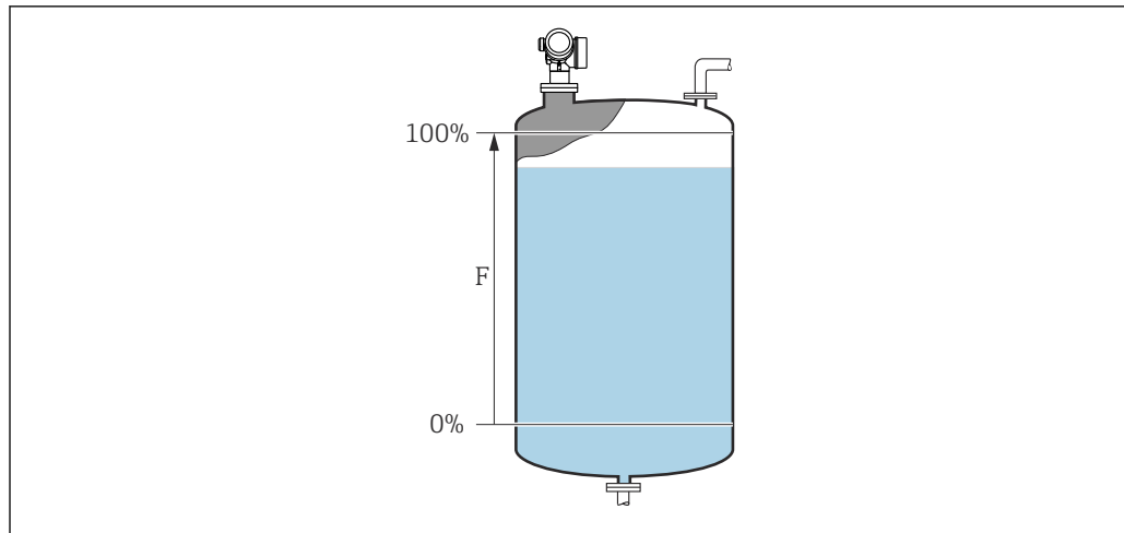
46 Калибровка полной емкости (F) для измерения уровня жидких сред
