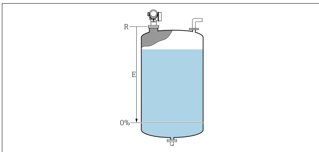
45 Калибровка пустой емкости (E) для измерения уровня жидких сред
