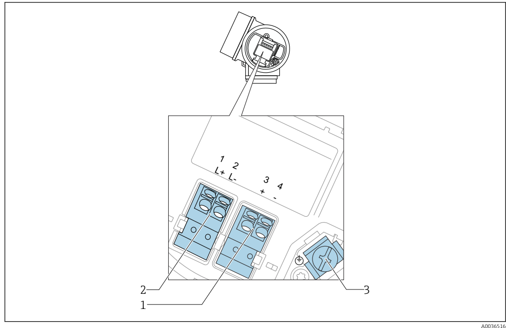
16 Asignación de terminales a cuatro hilos: 4-20 mA HART (10,4 ... 48 V DC )
