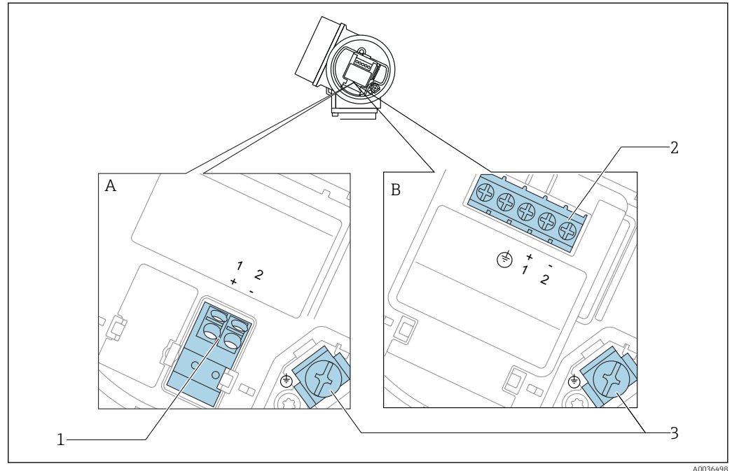
10 Asignación de terminales a 2 hilos: 4-20 mA HART
