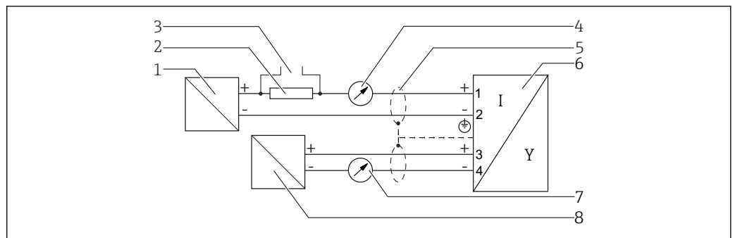
15 Diagrama en bloque a dos hilos: 4-20 mA HART, 4-20 mA
