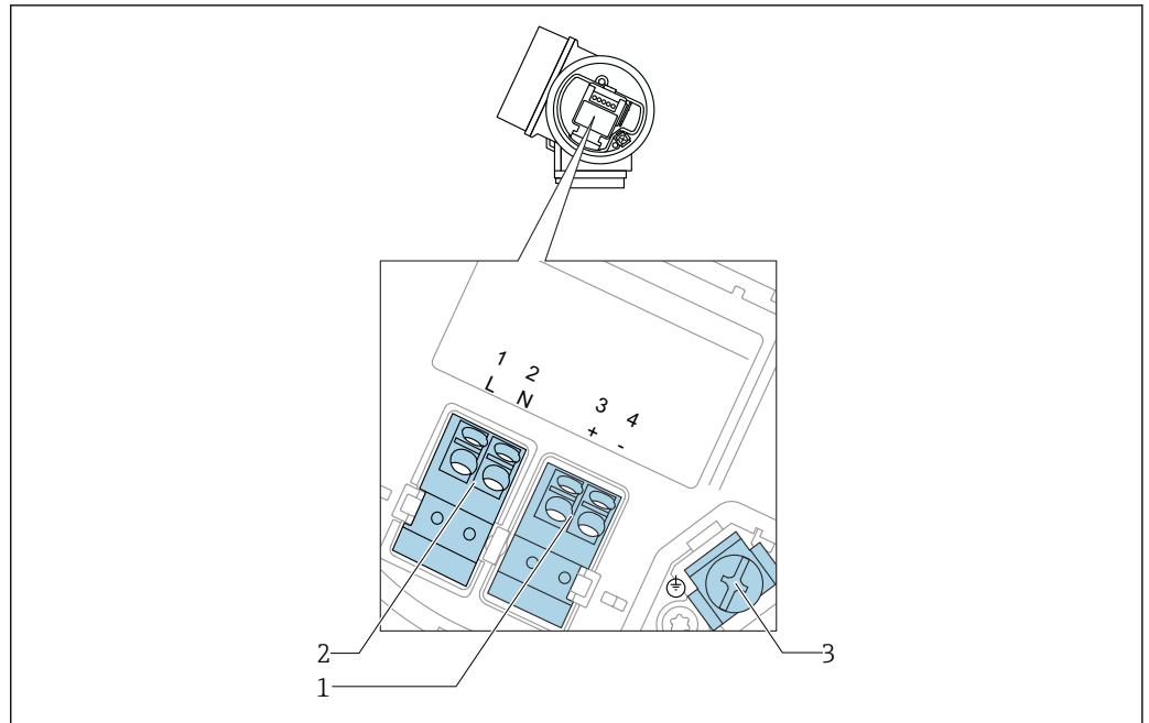
18 Asignación de terminales a cuatro hilos: 4-20 mA HART (90 ... 253 V AC )
