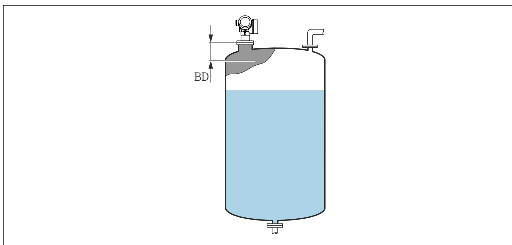
52 Distancia de bloqueo (BD) para mediciones de líquidos
