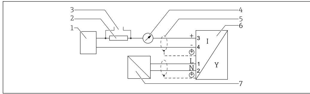
19 Diagrama en bloque a cuatro hilos: 4-20 mA HART (90 ... 253 V AC )
