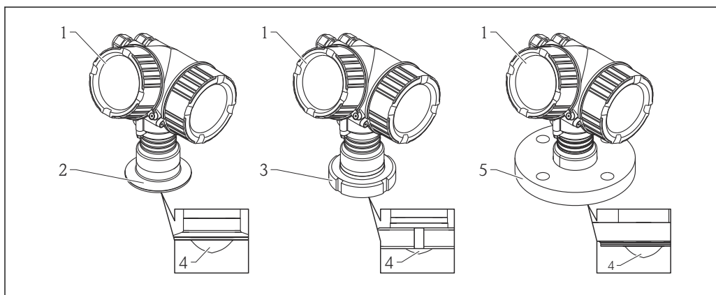
2 Diseño del Micropilot FMR52 (26 GHz)
