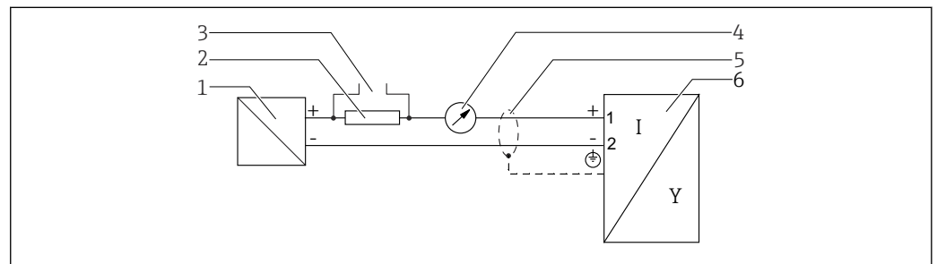
11 Diagrama en bloque a dos hilos: 4-20 mA HART
