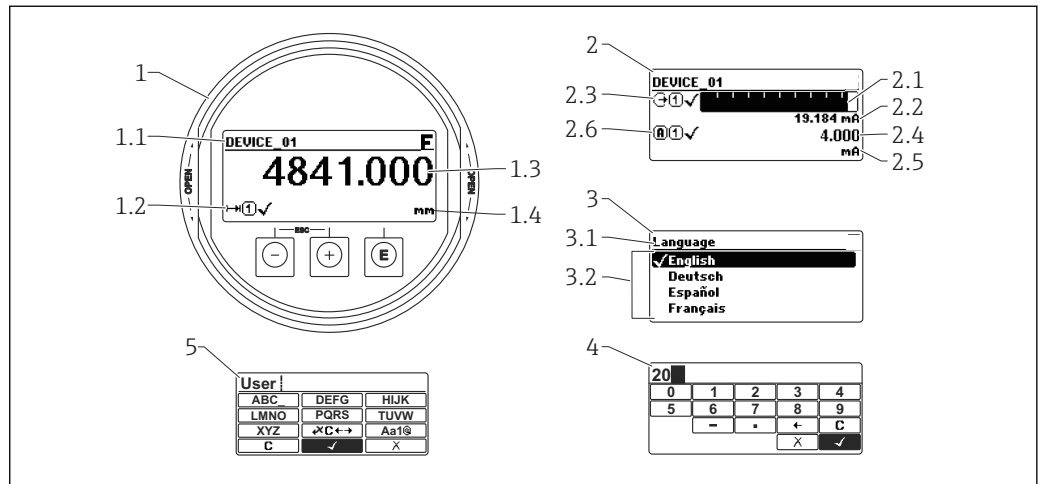
29 Aspecto del indicador y módulo para operaciones en campo
