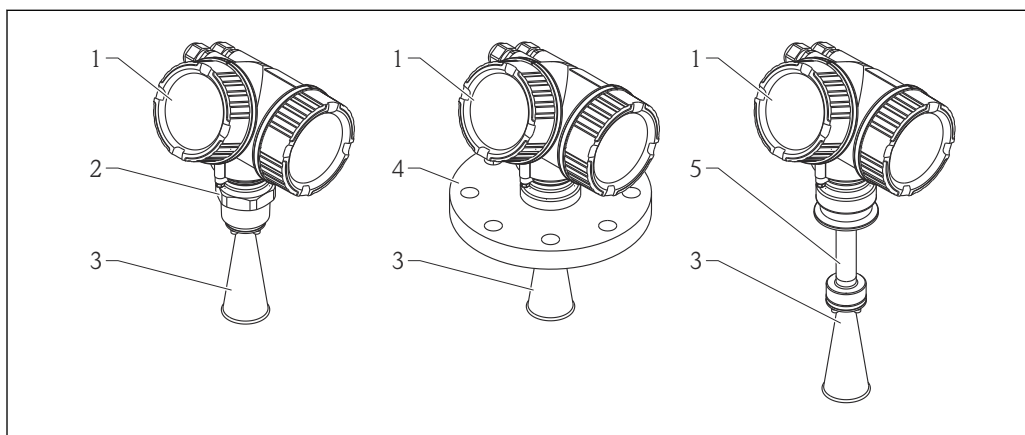
1 Diseño del Micropilot FMR51 (26 GHz)
