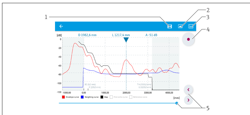
36 Visualización de la curva envolvente (ejemplo) en SmartBlue; vista en Android
