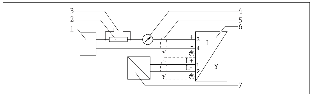
17 Diagrama en bloque a cuatro hilos: 4-20 mA HART (10,4 ... 48 V DC )
