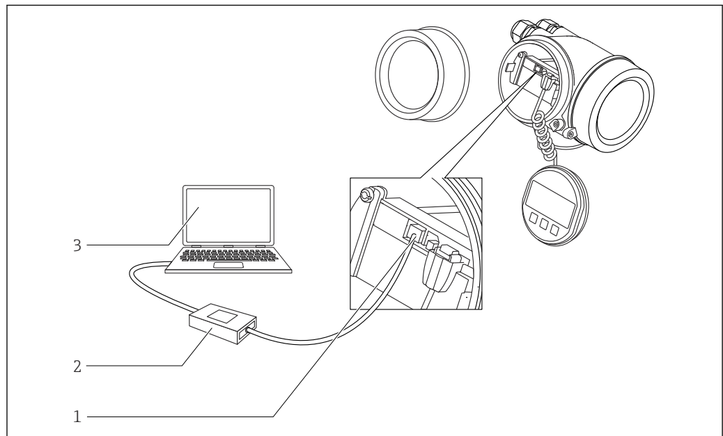
28 DeviceCare/FieldCare mediante interfaz de servicio (CDI)
