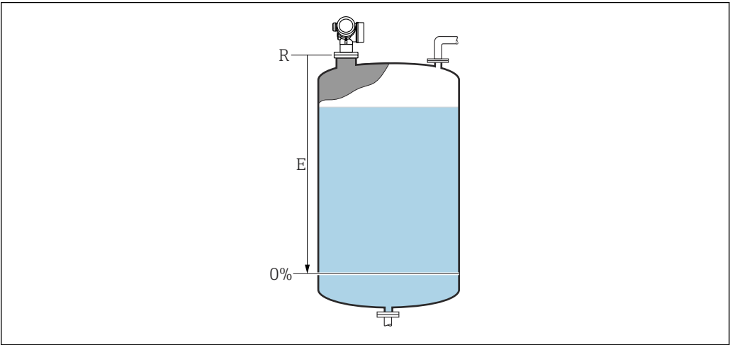
44 Calibración vacío (E) para mediciones de nivel en líquidos
