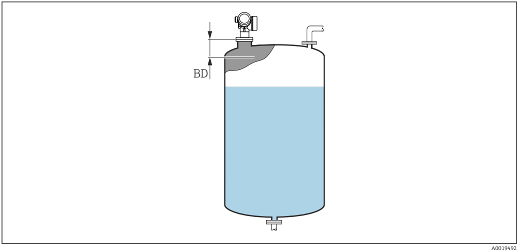
48 Distancia de bloqueo (BD) para mediciones de líquidos
