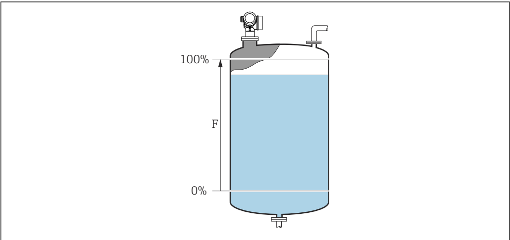
45 Calibración lleno (F) para mediciones de nivel en líquidos
