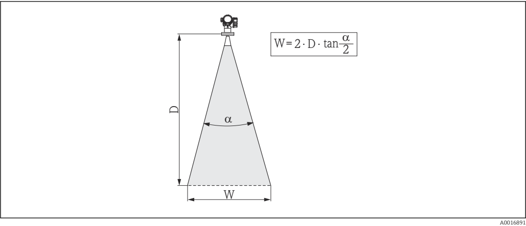
5 Relación entre ángulo de abertura del haz \alpha , distancia D y diámetro del haz W
