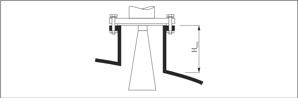
6 Altura de la tubuladura para una antena de trompeta (FMR51)
