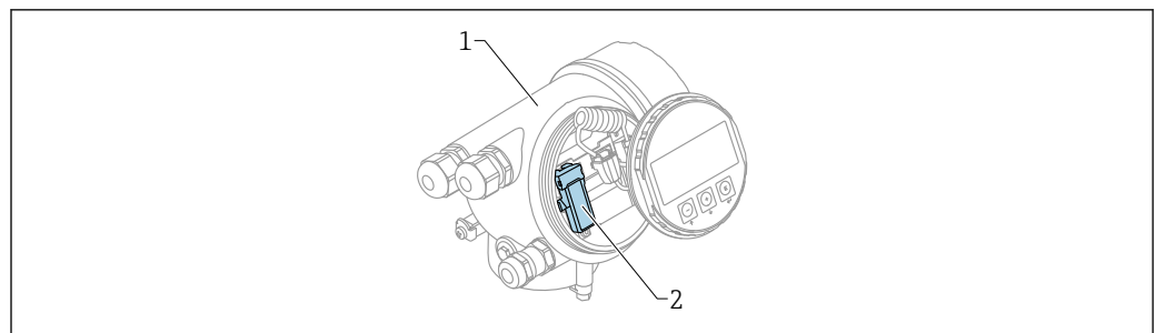
30 Dispositivo con módulo Bluetooth
