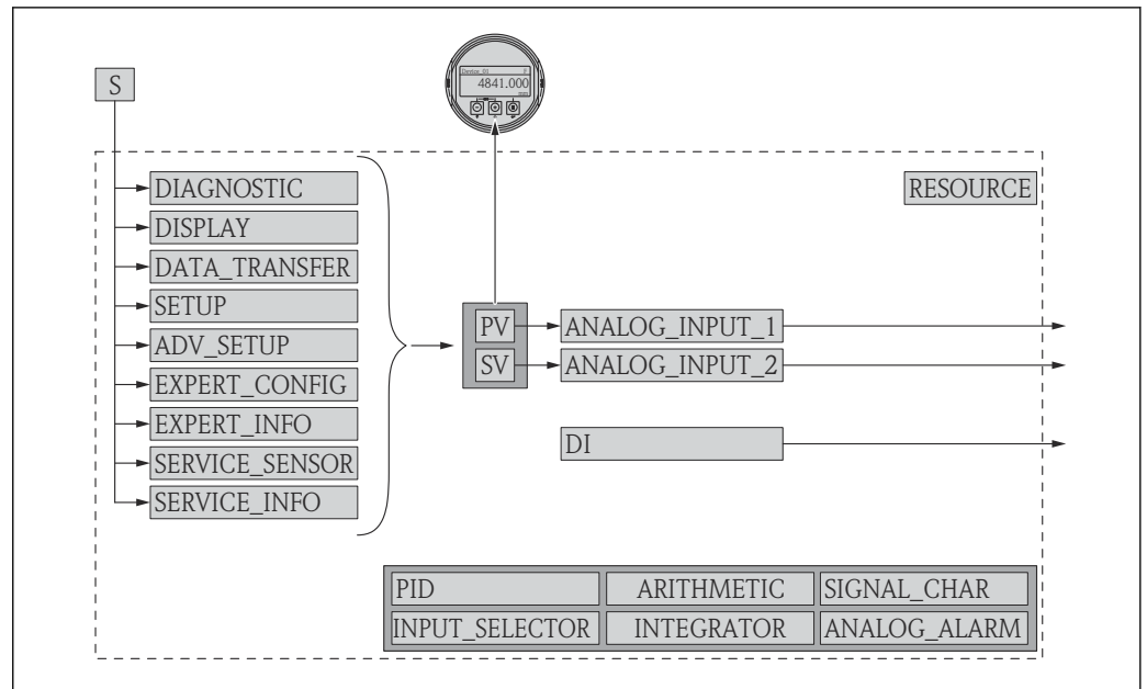
図 22 出荷時のブロック設定
