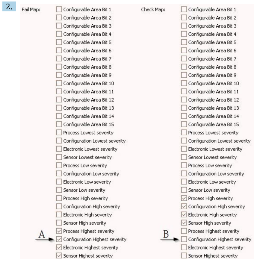
図 27 「故障マップ (Fail Map)」列と「チェックマップ (Check Map)」列のデフォルトの状態
