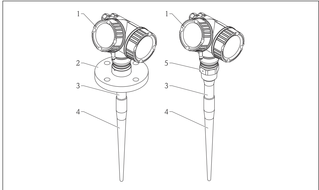
図 1 Micropilot FMR53 (6 GHz) の構成
