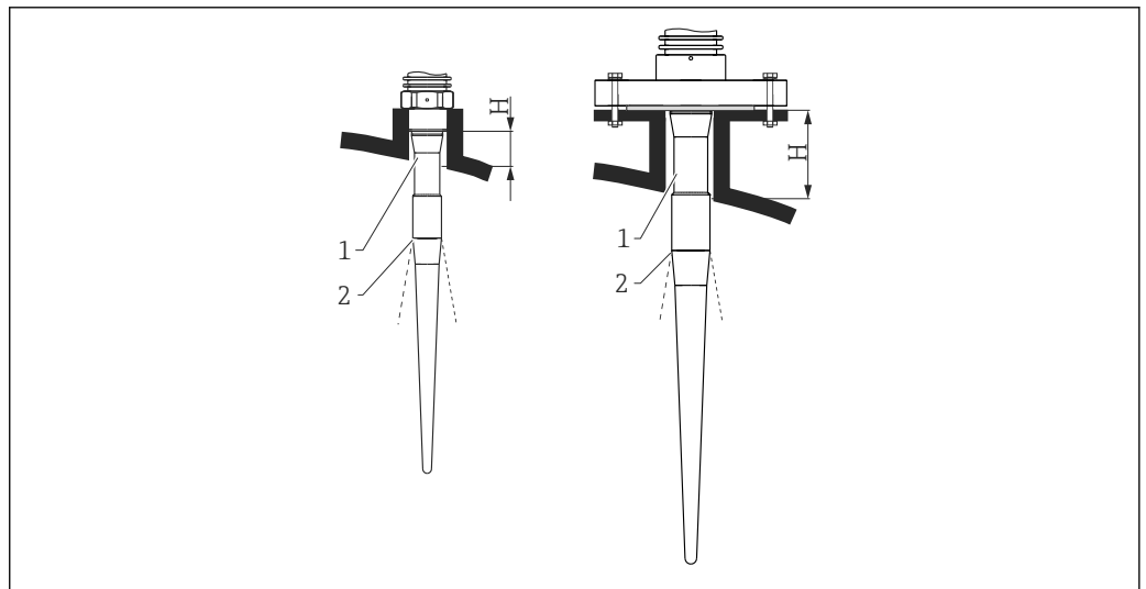
図 6 ロッドアンテナ (FMR53) のノズル高と直径
