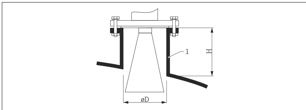
図 7 ホーンアンテナ (FMR54) のノズル高と直径
