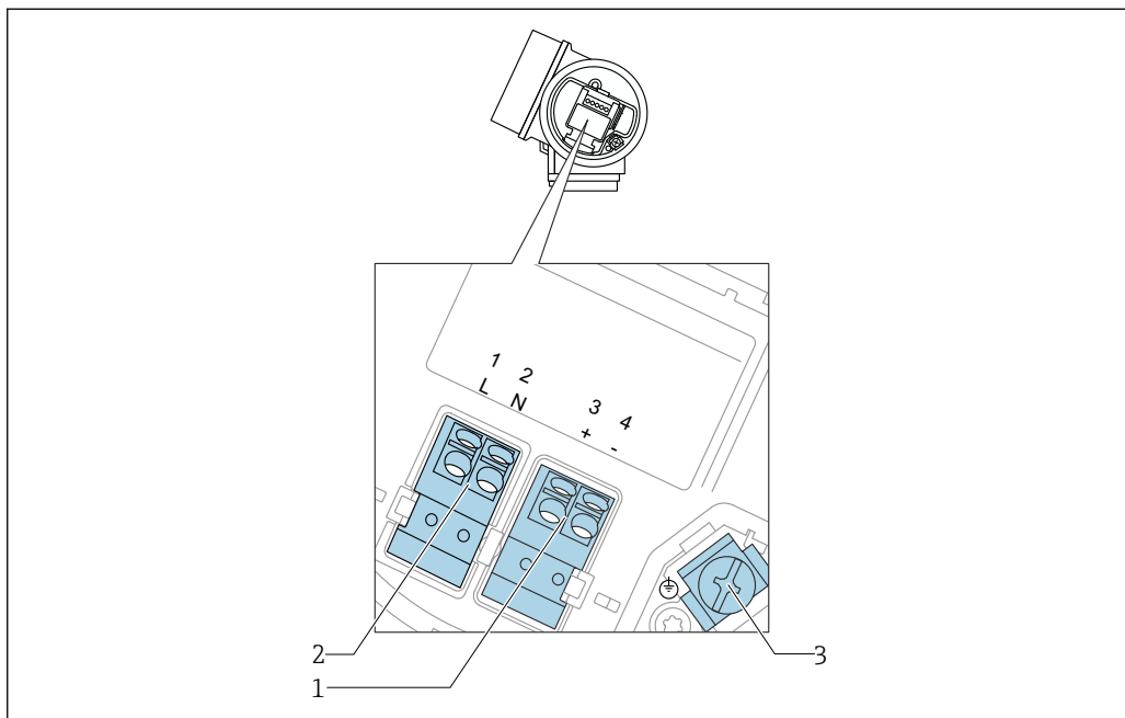
図 10 4 線式、4~20 mA HART の端子割当て (90~253 V AC )
