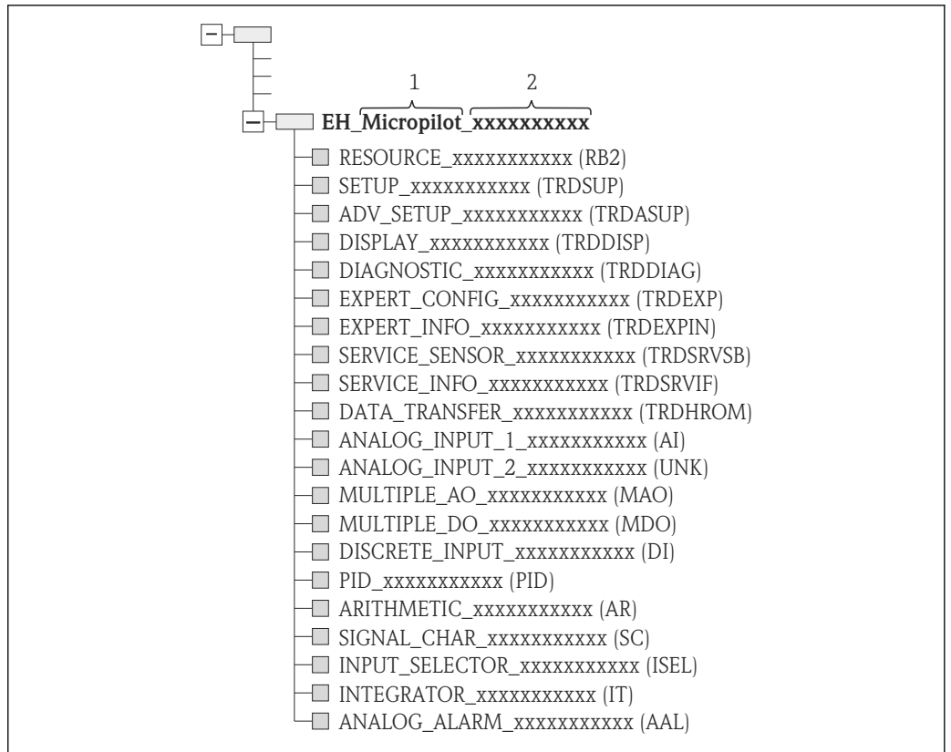
図 21 接続を確立した後の設定プログラムの標準的な表示ディスプレイ
