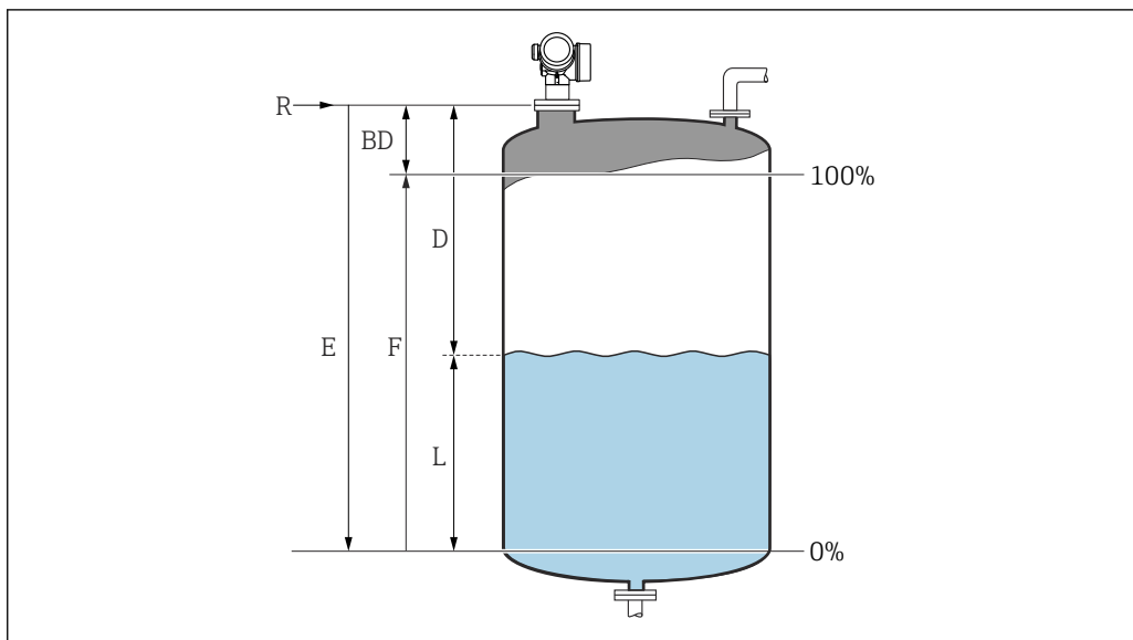
図 24 液体のレベル測定用パラメータの設定
