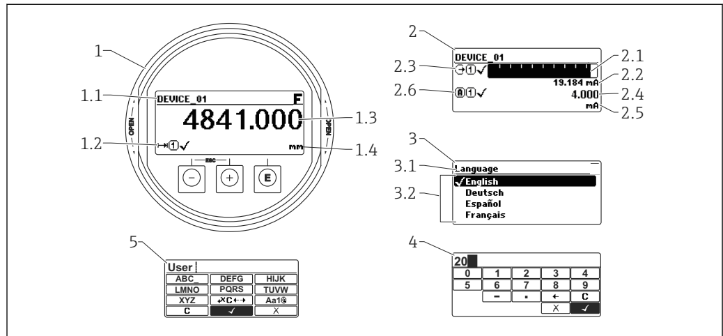
図 20 現場操作の表示部および操作モジュールの表示
