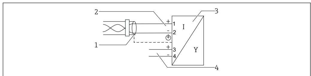
図 12 ブロック図 : PROFIBUS PA / FOUNDATION フィールドバス
