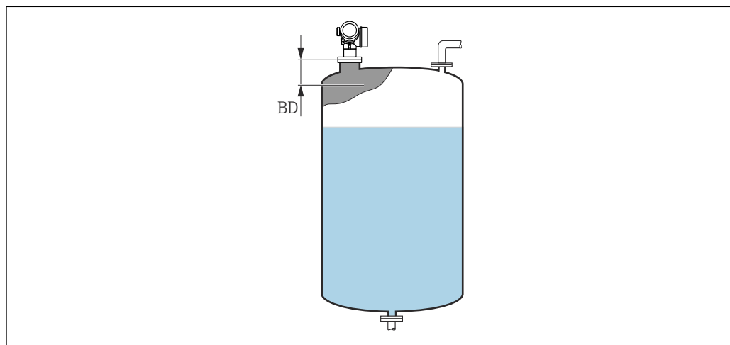
図 40 液体計測の不感知距離 (BD)
