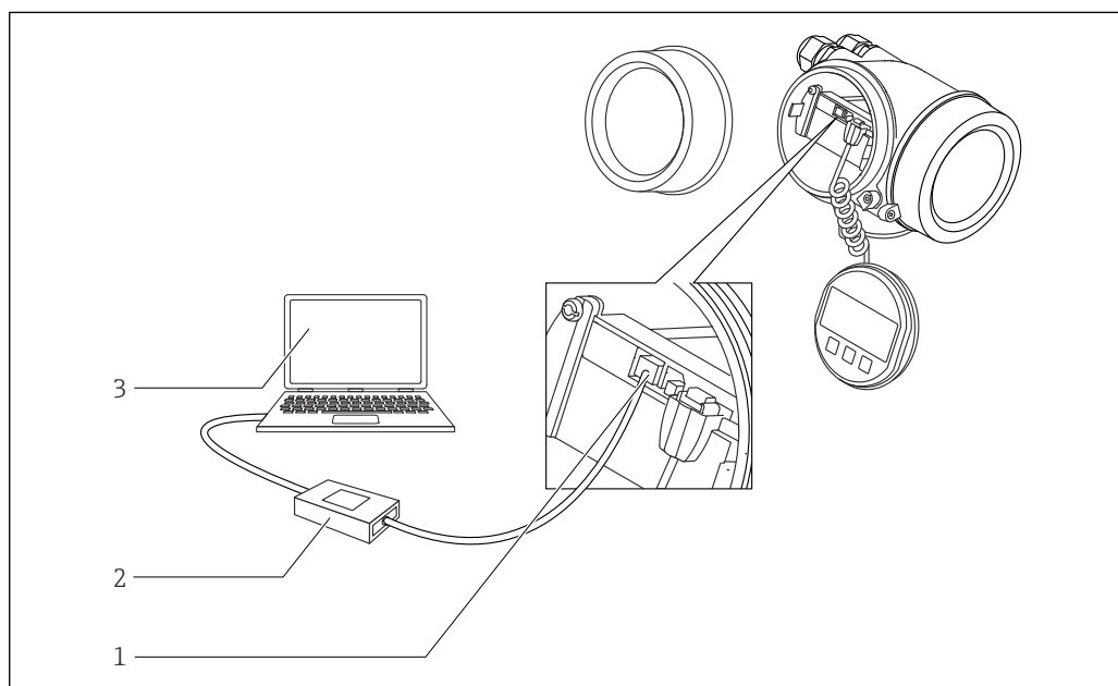
図 19 サービスインターフェイス（CDI）経由の DeviceCare/FieldCare
