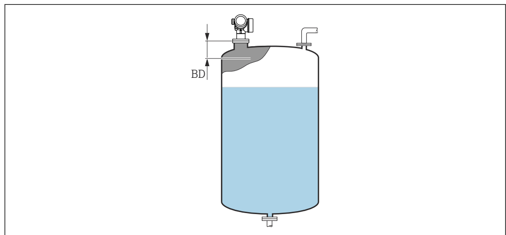
④ 36 液体計測の不感知距離 (BD)
