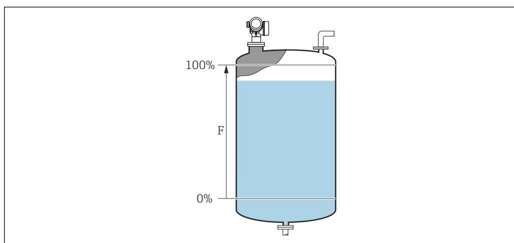
図 33 液体レベル測定用の満量校正 (F)
