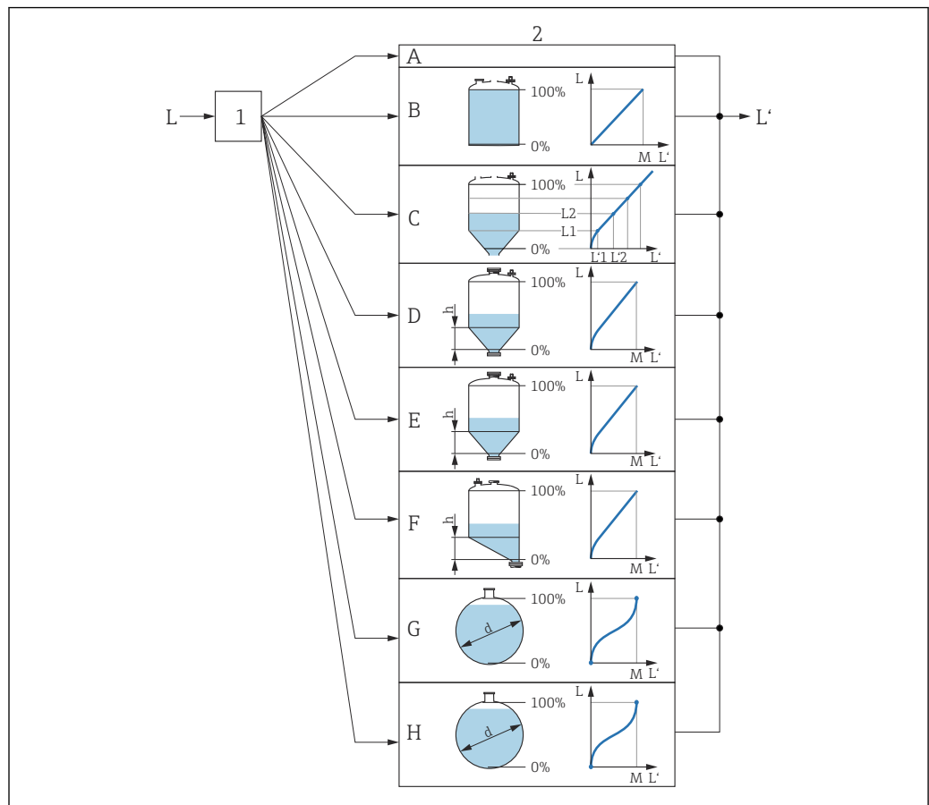
図 38 リニアライゼーション：レベルおよび界面の高さ（該当する場合）を容量または質量に変換します。これは容器の形状に応じて異なります。
