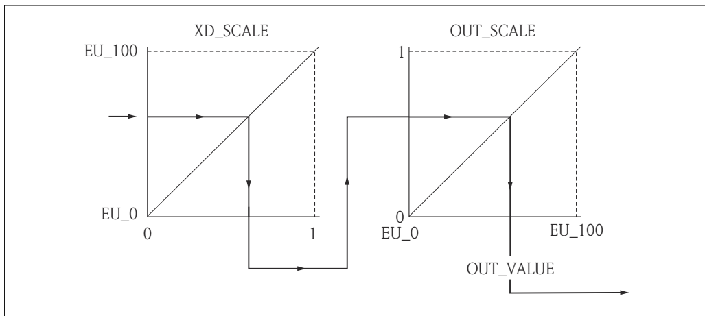
図 26 AI ブロックでの測定値のスケーリング
