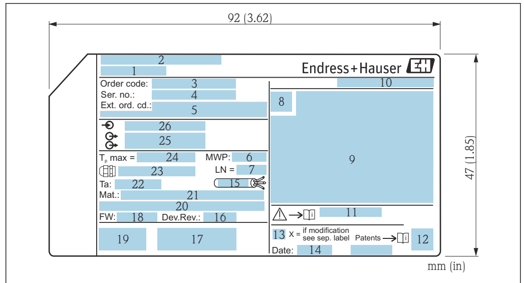
図 4 Micropilot の銘板
