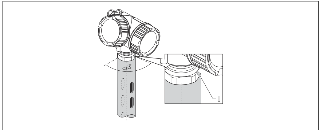
図 8 内筒管への設置
