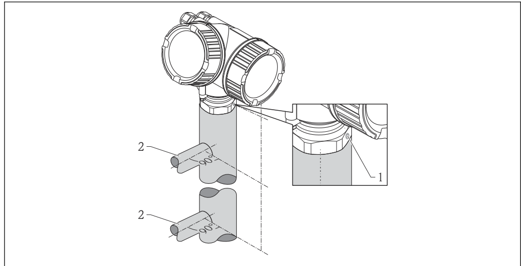
図 9 外筒管への設置
