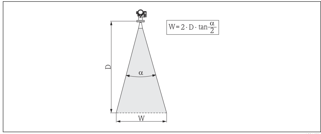
図 5 ビーム放射角 \alpha 、距離 D およびビーム幅 W の関係
