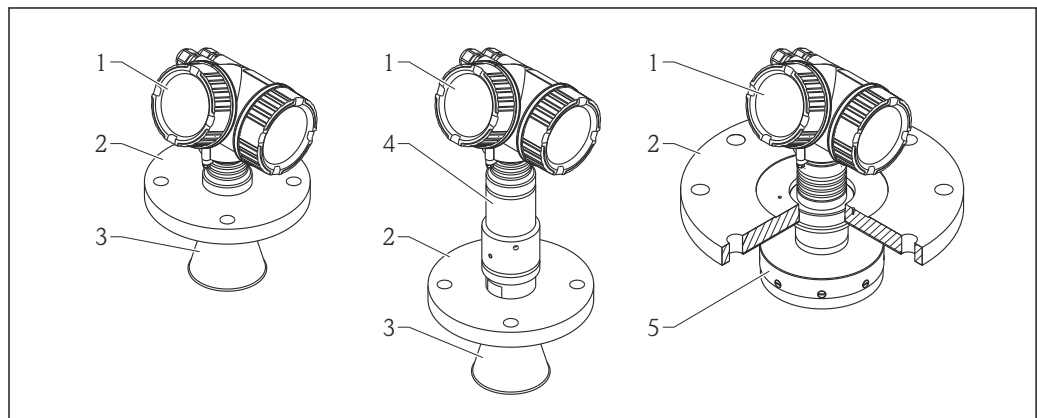
図 2 Micropilot FMR54 (6 GHz) の構成
