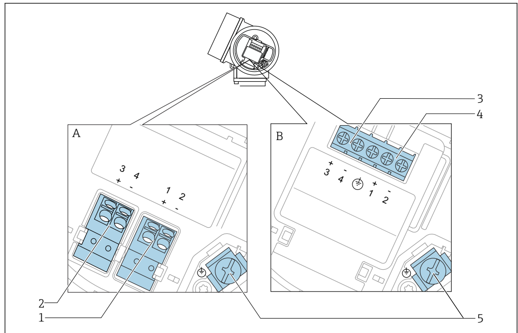
図 11 PROFIBUS PA/ FOUNDATION Fieldbus の端子割当
