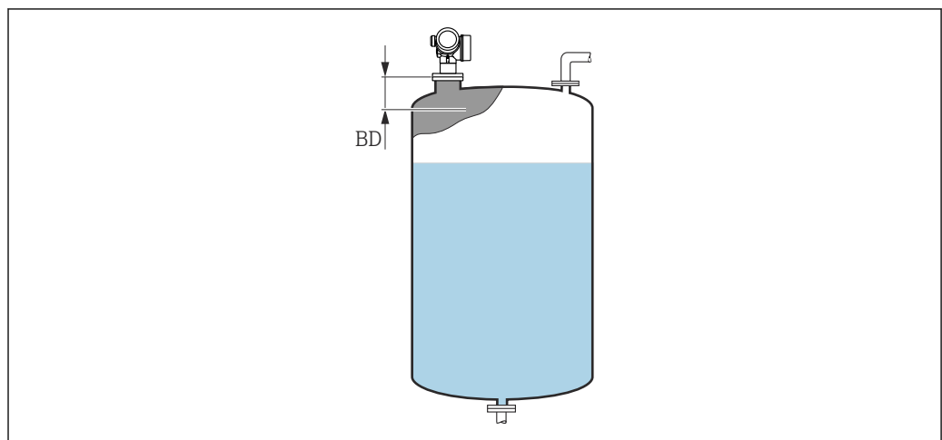
④ 34 液体計測の不感知距離 (BD)
