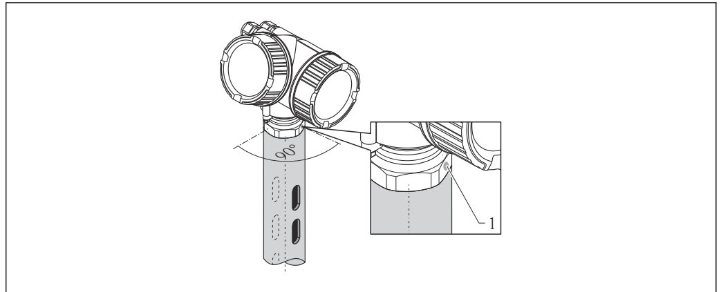
図 8 内筒管への設置
