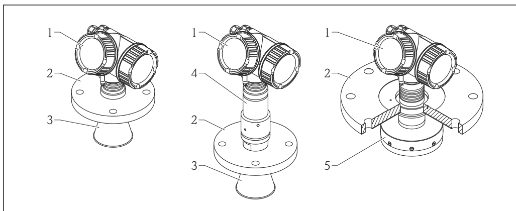
図 2 Micropilot FMR54 (6 GHz) の構成
