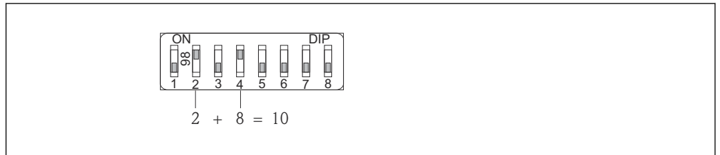
図 22 ハードウェアアドレス指定の例：スイッチ 8 を「オフ」位置にし、スイッチ 1～7 にアドレスを定義します。
