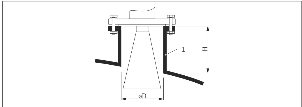
図 7 ホーンアンテナ (FMR54) のノズル高と直径
