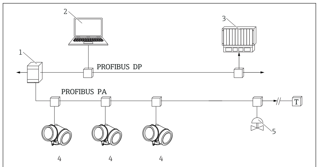
図 18 PROFIBUS PA プロトコルを介したリモート操作のオプション
