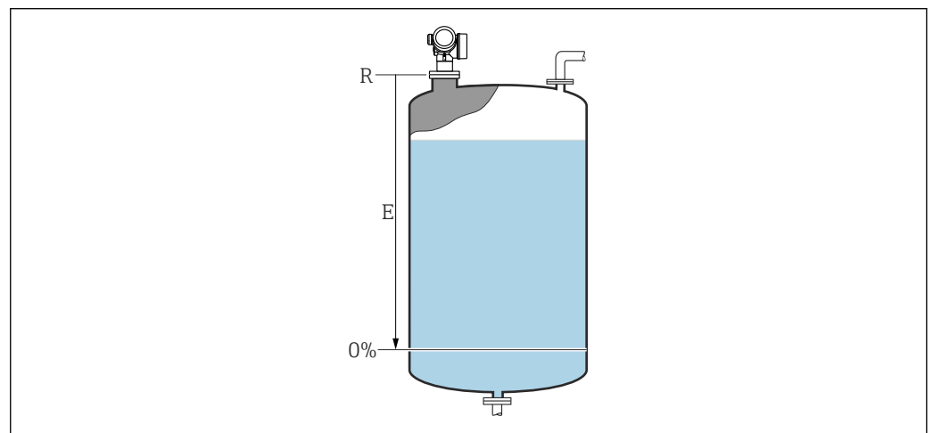
30 液体レベル測定用の空校正 (E)
