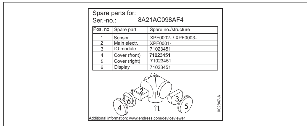
図 28 端子部カバーのスペアパーツ型式銘板の例
