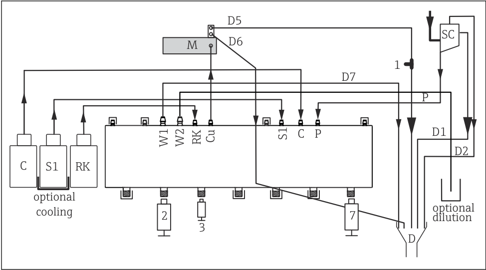
23 Liquiline System CA80NO, equipo de canal único
