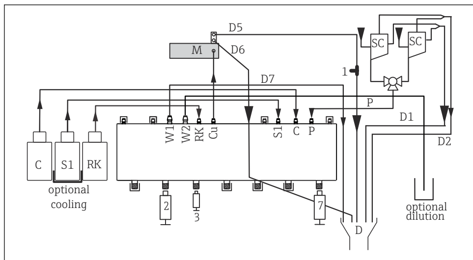
24 Liquiline System CA80NO, equipo a dos canales
