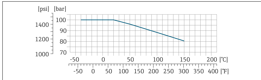
图 18 连接部件材质: 1.4404 (316/316L)
