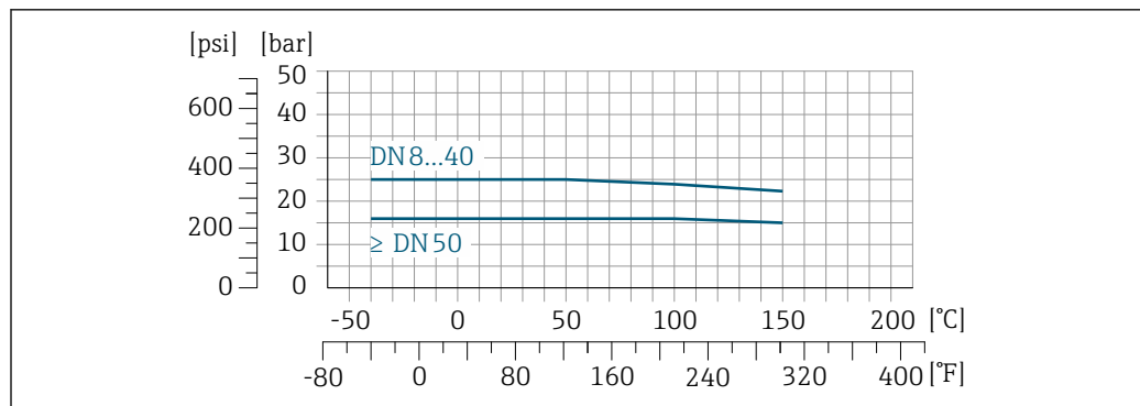
图 13 法兰材质: 1.4404 (316/316L)
