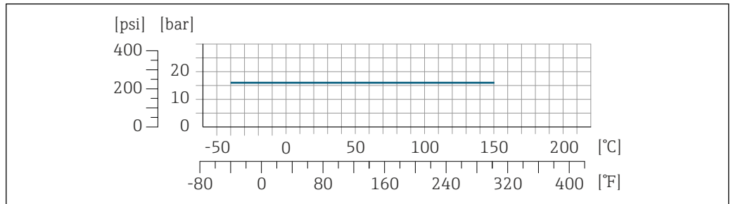
17 连接部件材质: 1.4404 (316/316L)
