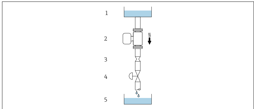
图 8 在竖直向下管道中安装(例如：批处理应用)
