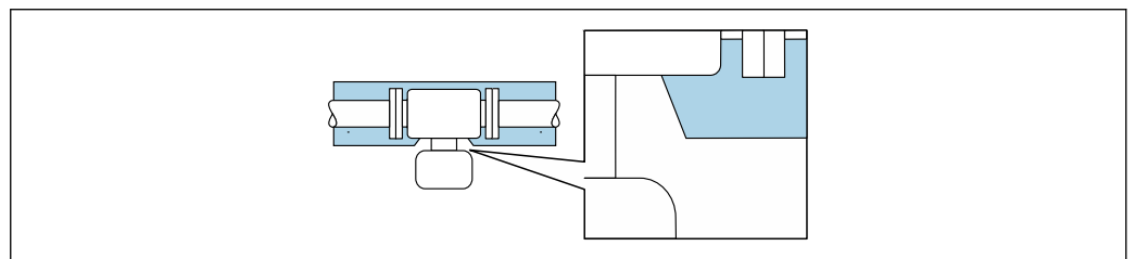
19 延长颈上无保温层覆盖
