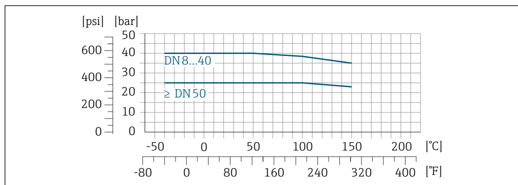
图 14 连接部件材质: 1.4404 (316/316L)
