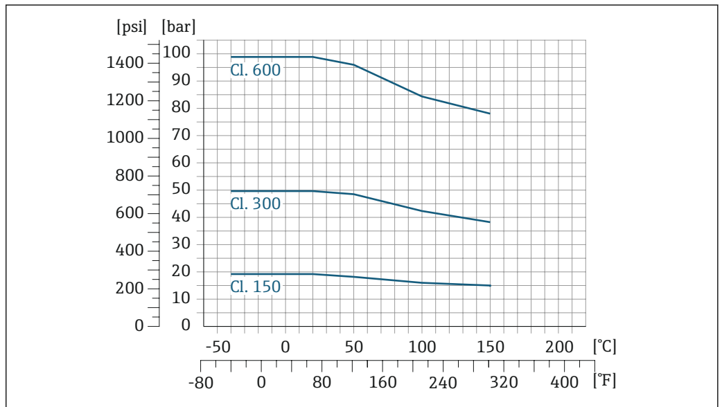
图 11 法兰材质: 1.4404 (F316/F316L)
