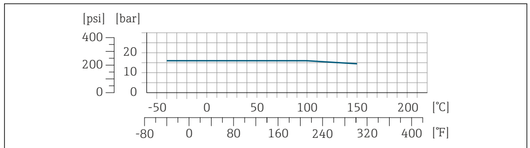
16 连接部件材质: 1.4404 (316/316L)
