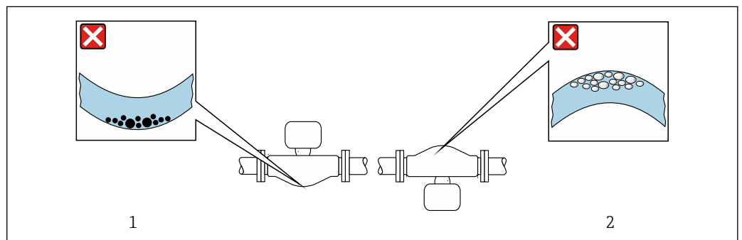
☒ 9 带弯测量管的传感器的安装方向
