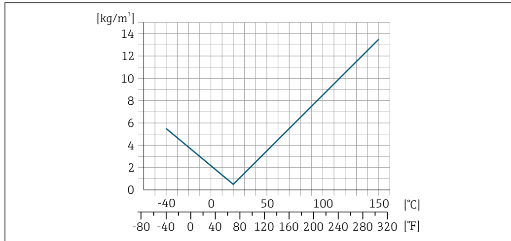
图 7 现场密度校准, 例如在 +20^{\circ}\text{C} ( +68^{\circ}\text{F} )时
