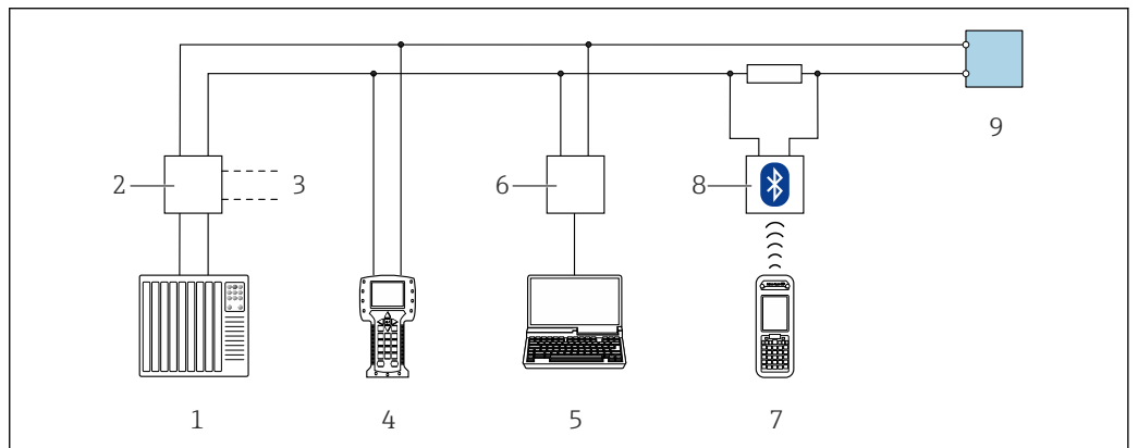
图 23 通过 HART 通信进行远程操作（无源信号）
