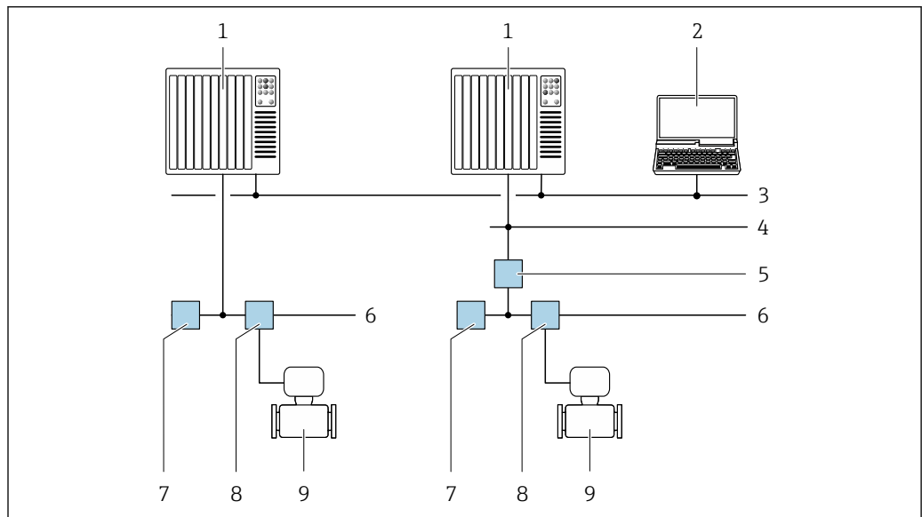
图 25 通过基金会现场总线(FF)网络进行远程操作
