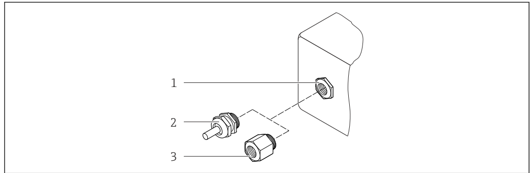
图 21 允许的电缆入口/缆塞
