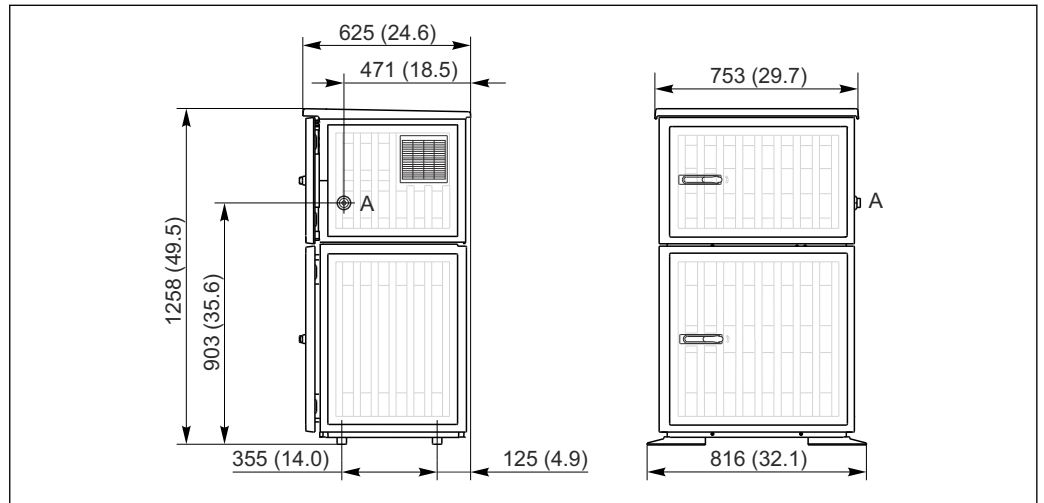
3 Dimensioni della versione in plastica di Liquistation CSF33 , dimensioni in mm (in)
