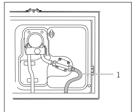
11 Tubo di aspirazione
