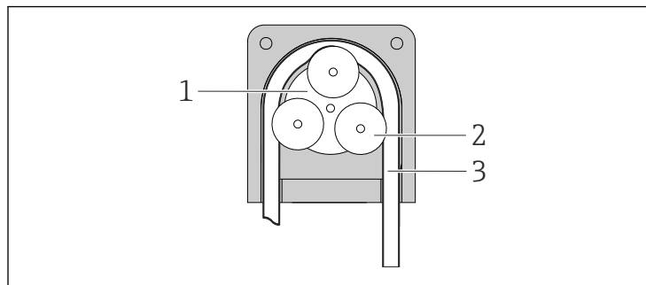
48 Vista interna della pompa peristaltica
