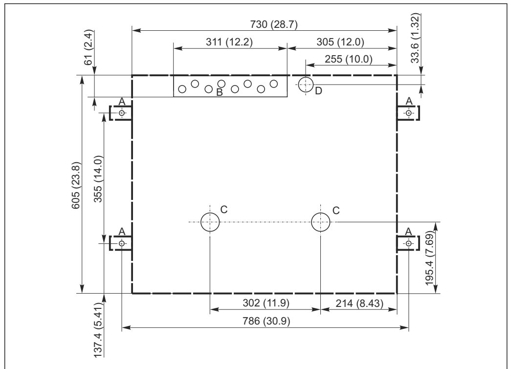
6 Disegno della base di ancoraggio
