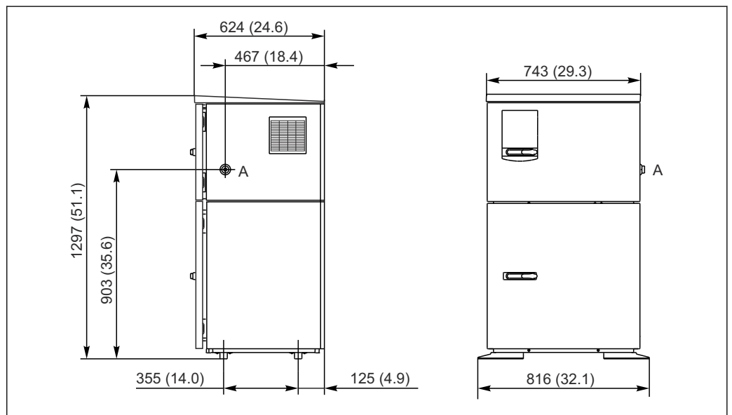
4 Dimensioni della versione in acciaio inox di Liquistation CSF33 , dimensioni in mm (in)
