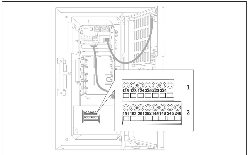
18 Posizione dei morsetti
