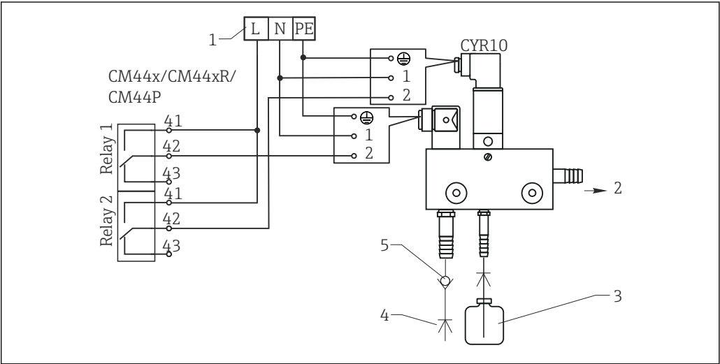
39 Connessione del sistema di pulizia con iniettore CYR10
