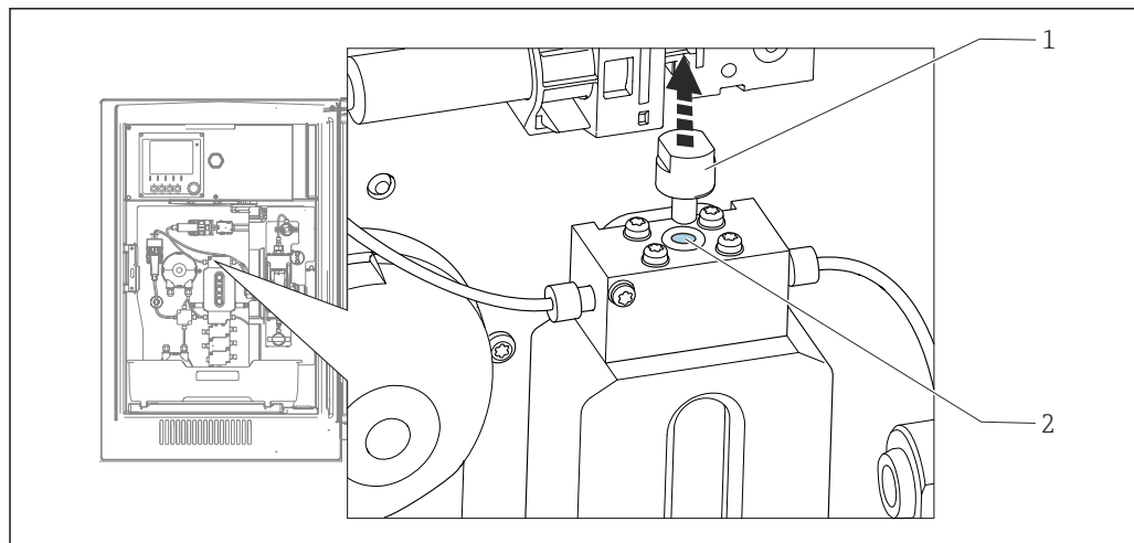
69 Unità di dosaggio con apertura per la pulizia
