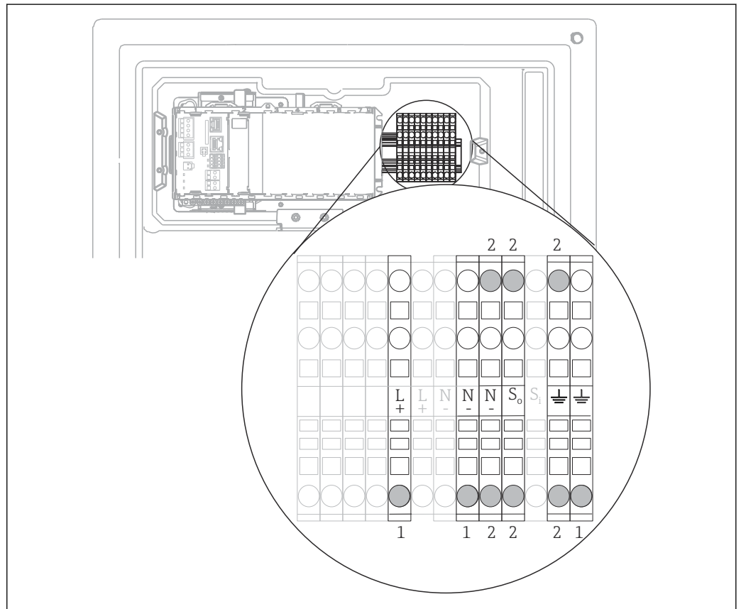
22 Assegnazione dei morsetti per la versione "outdoor"
