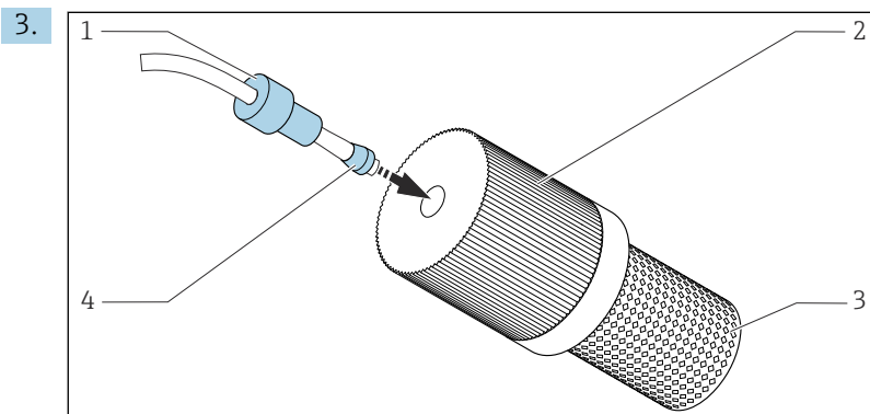
54 Montaggio del filtro di aspirazione (fornito) sul tubo flessibile di prelievo
