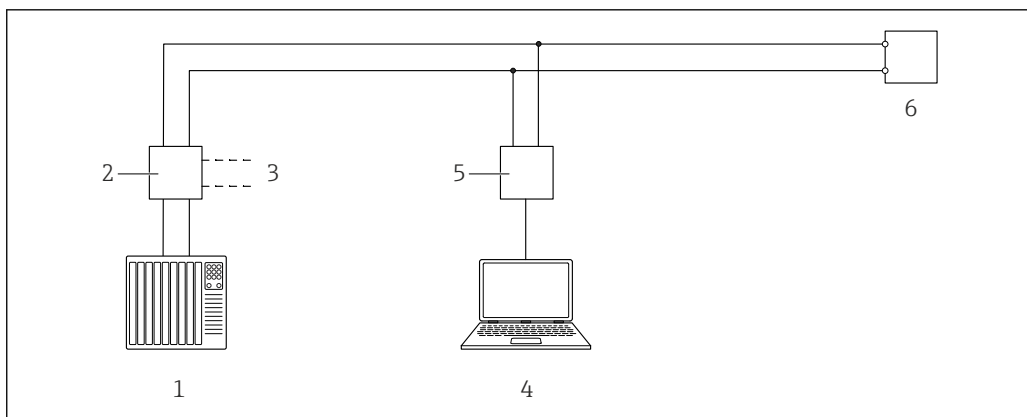
図 8 HART プロトコルによる遠隔制御
