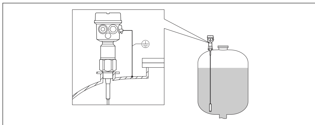
2 ローププローブ
