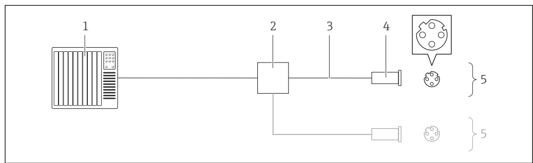
图 11 工业以太网(EtherNet/IP)的连接示例
