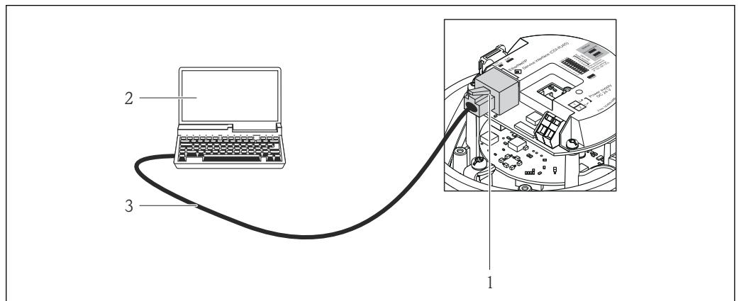
图 18 订购选项“输出”, 选型代号 N: 工业以太网 (EtherNet/IP)
