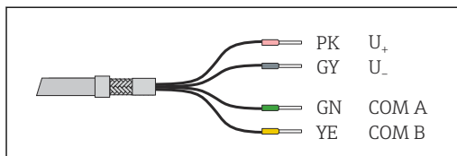
10 Pevně uchycený kabel senzoru se zakončenými kabelovými žilami
