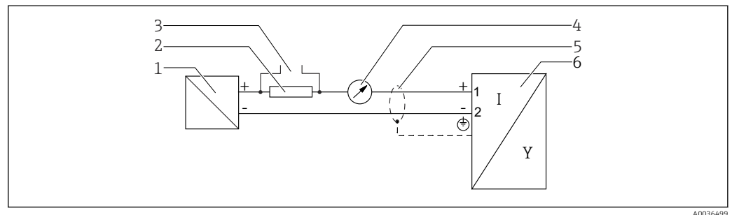
7 Diagramma a blocchi per dispositivo bifilare: 4-20 mA HART
