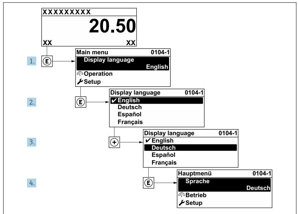
30 Esempio con il display locale
