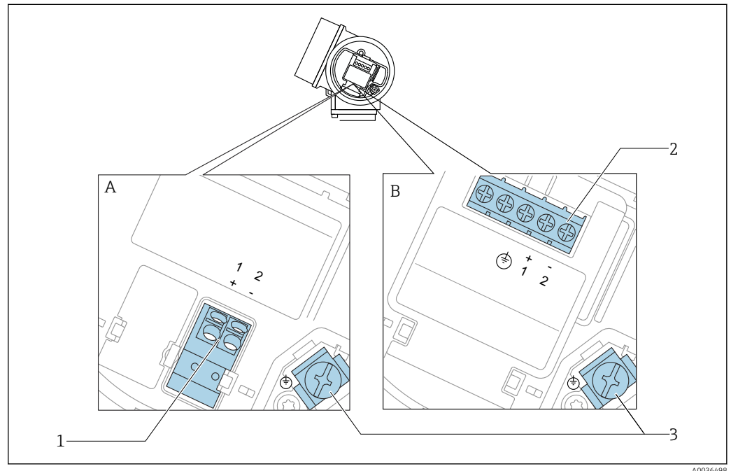
6 Assegnazione dei morsetti per dispositivo bifilare: 4-20 mA HART
