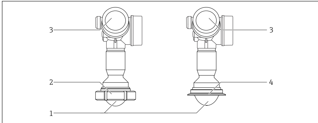
2 Costruzione del misuratore Micropilot FMR62
