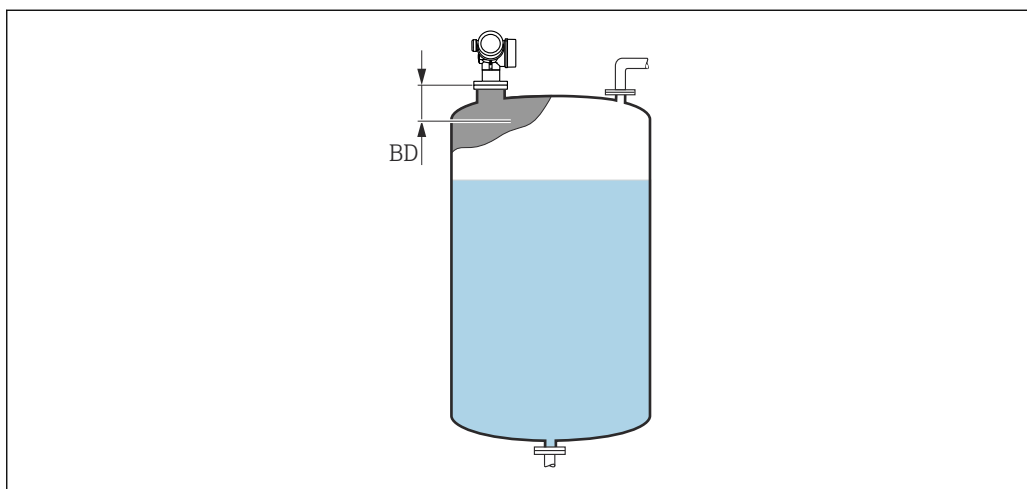
39 Distanza di blocco (BD) per misure di liquidi
