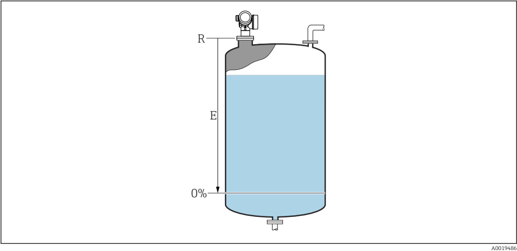
36 Calibrazione di vuoto (E) per misure di livello nei liquidi
