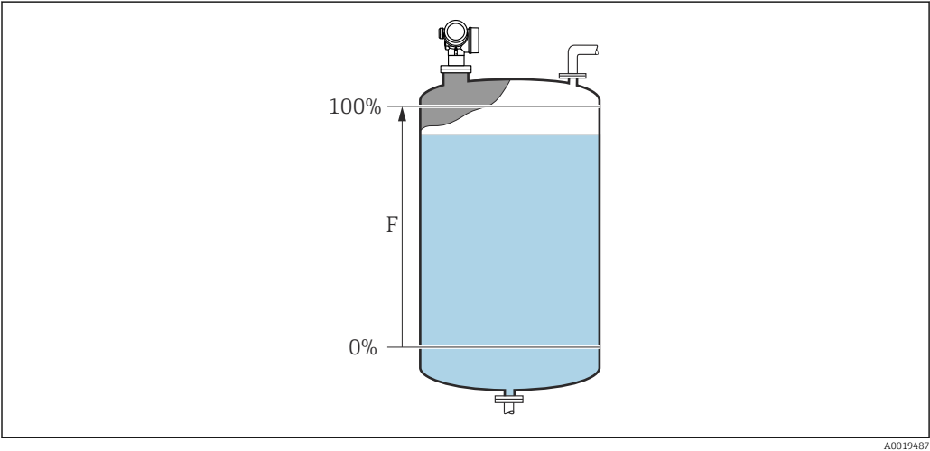
37 Calibrazione di pieno (F) per misure di livello nei liquidi
