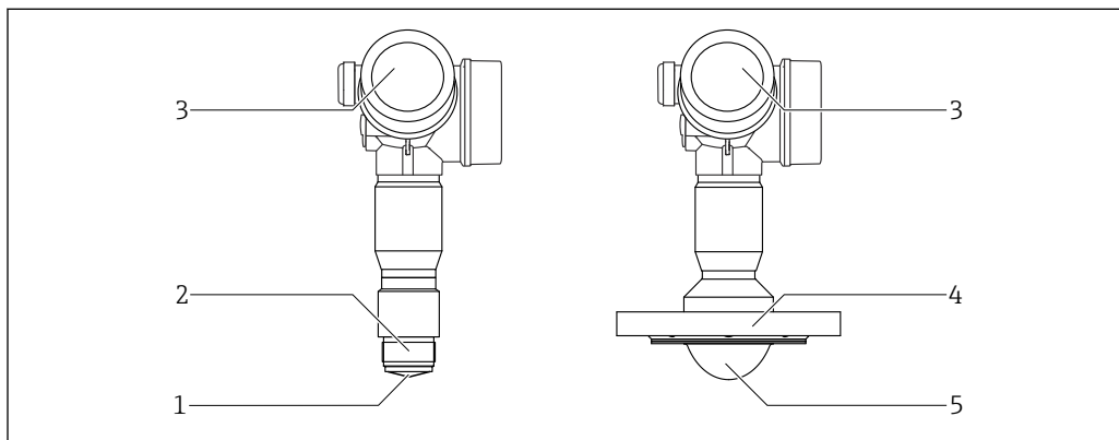
1 Costruzione del misuratore Micropilot FMR62
