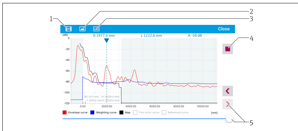
29 Visualizzazione della curva di involucro (esempio) in SmartBlue; vista iOS
