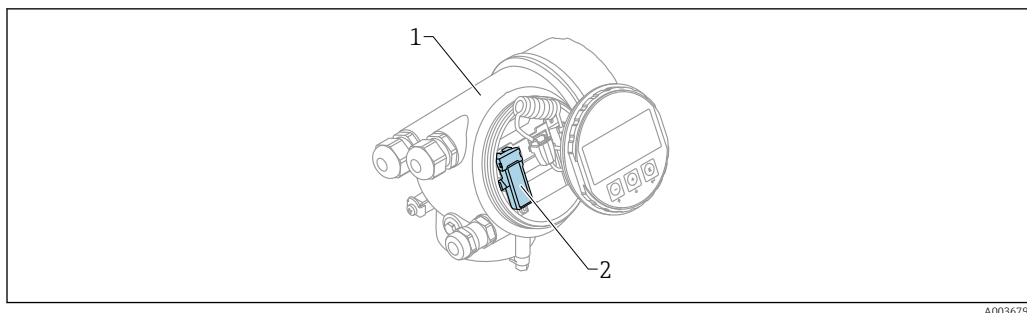
22 Dispositivo con modulo Bluetooth
