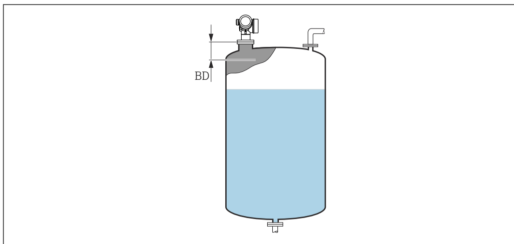
43 Distanza di blocco (BD) per misure di liquidi
