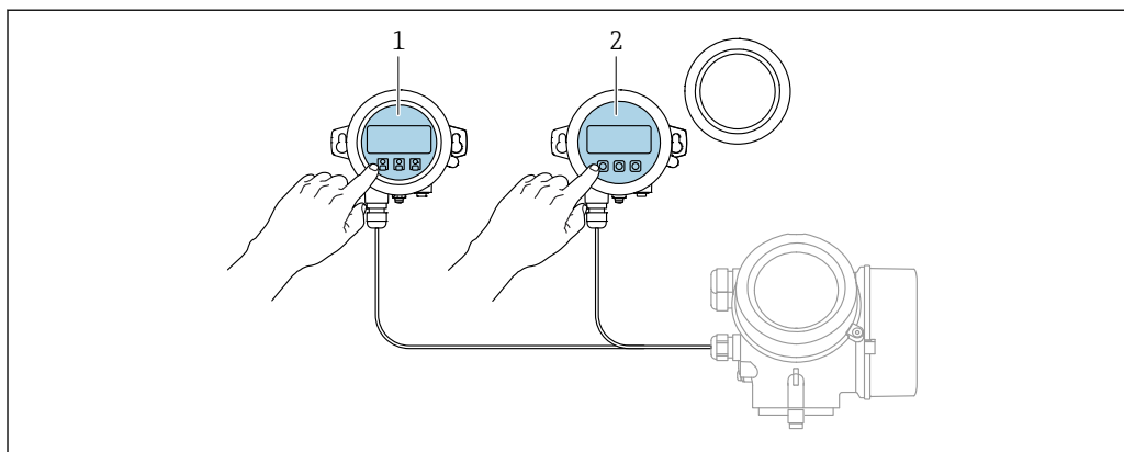
16 Opzioni operative FHX50
