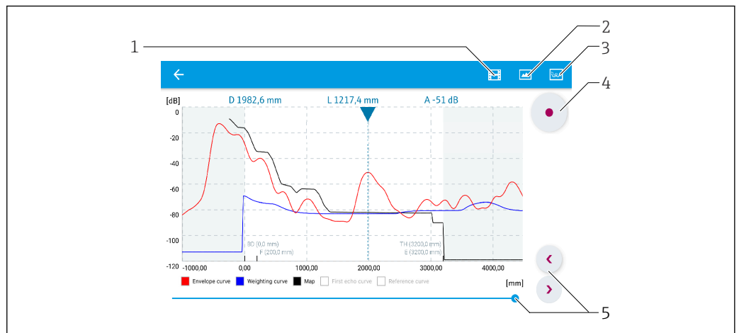
28 Отображение огибающей (пример) в приложении SmartBlue; устройство Android
