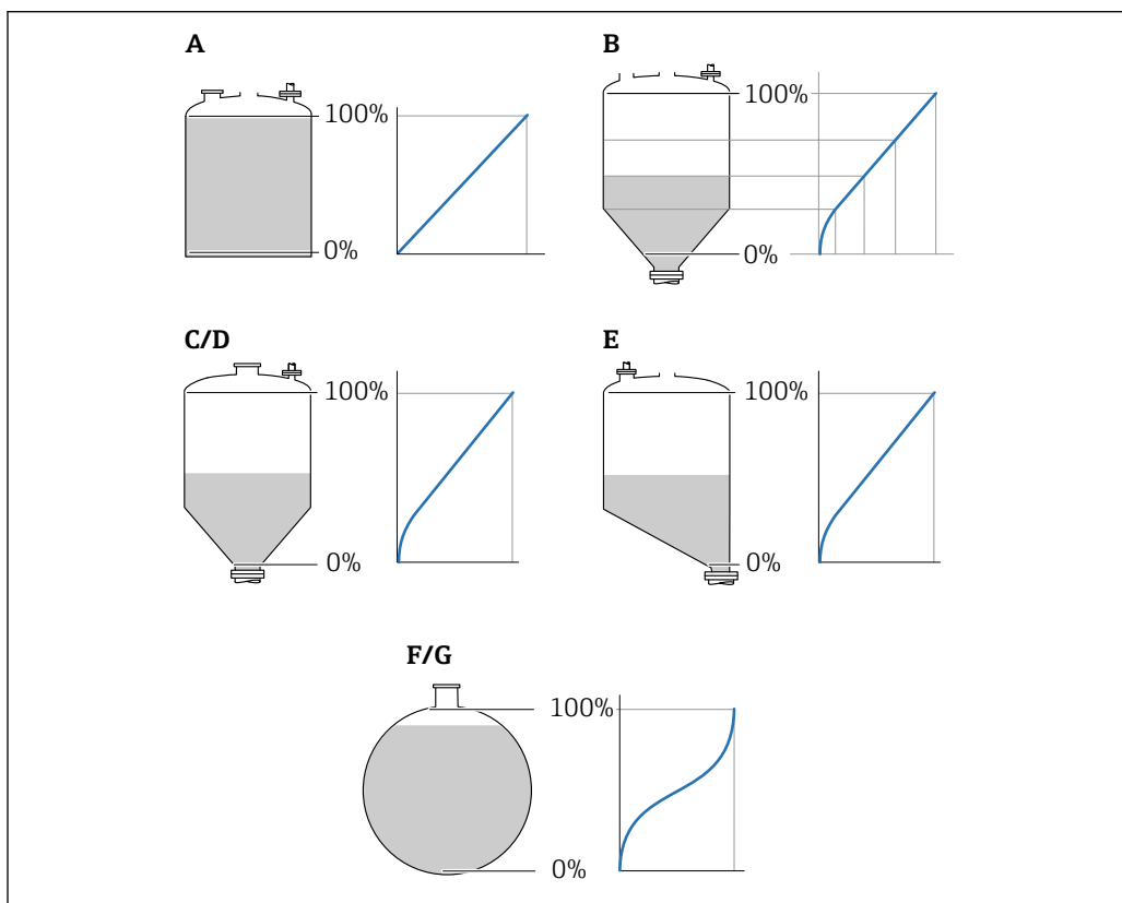
42 Типы линеаризации
