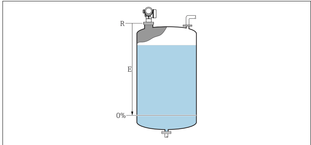
36 Калибровка пустой емкости (E) для измерения уровня жидких сред
