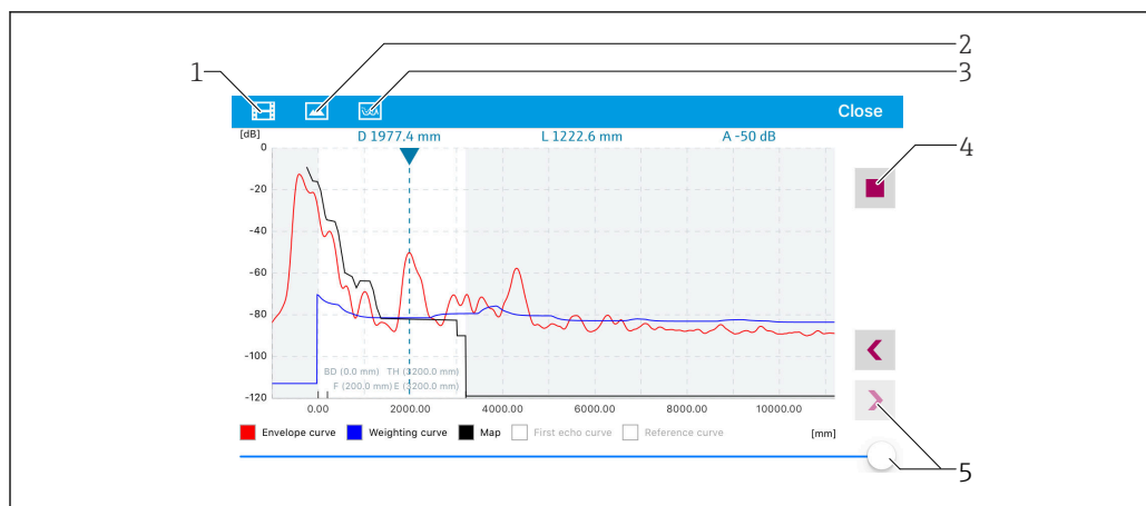
29 Отображение огибающей (пример) в приложении SmartBlue; устройство IoS
