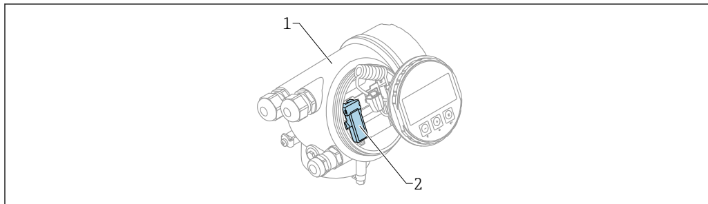
▣ 17 Прибор с модулем Bluetooth
