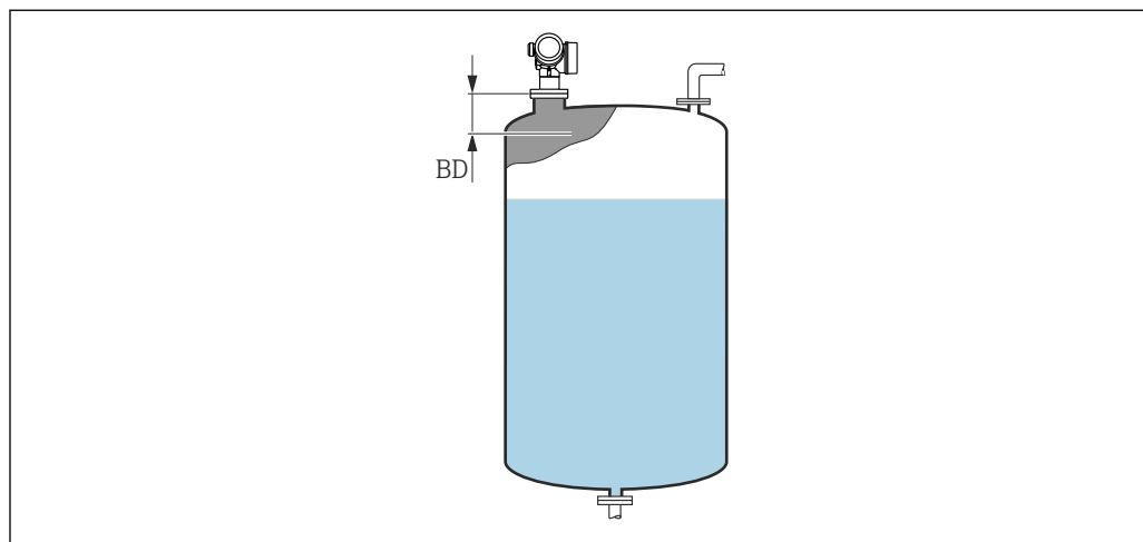
43 Блокирующая дистанция (BD) для измерения в жидких средах
