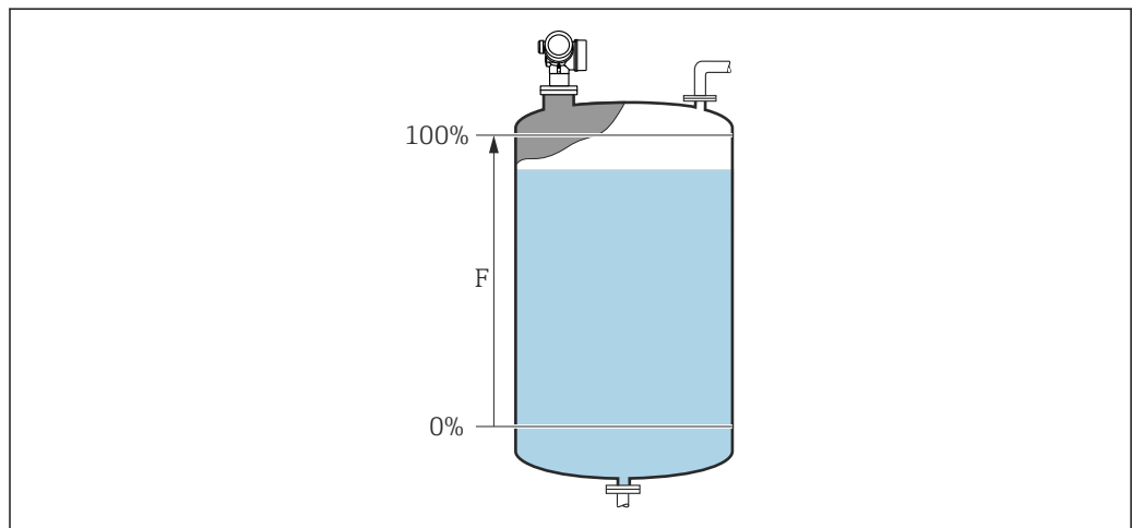
37 Калибровка полной емкости (F) для измерения уровня жидких сред
