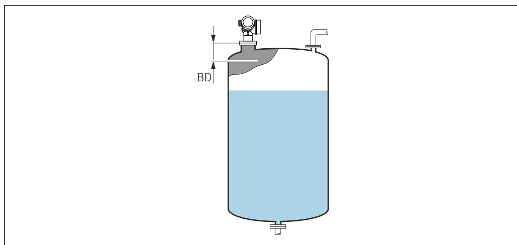
39 Блокирующая дистанция (BD) для измерения в жидких средах
