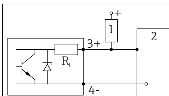
13 Подключение цифрового входа
