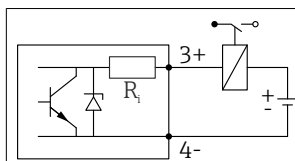
12 Подключение реле
