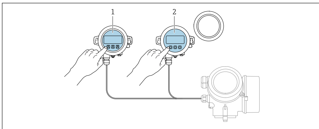
図 16 FHX50 操作オプション
