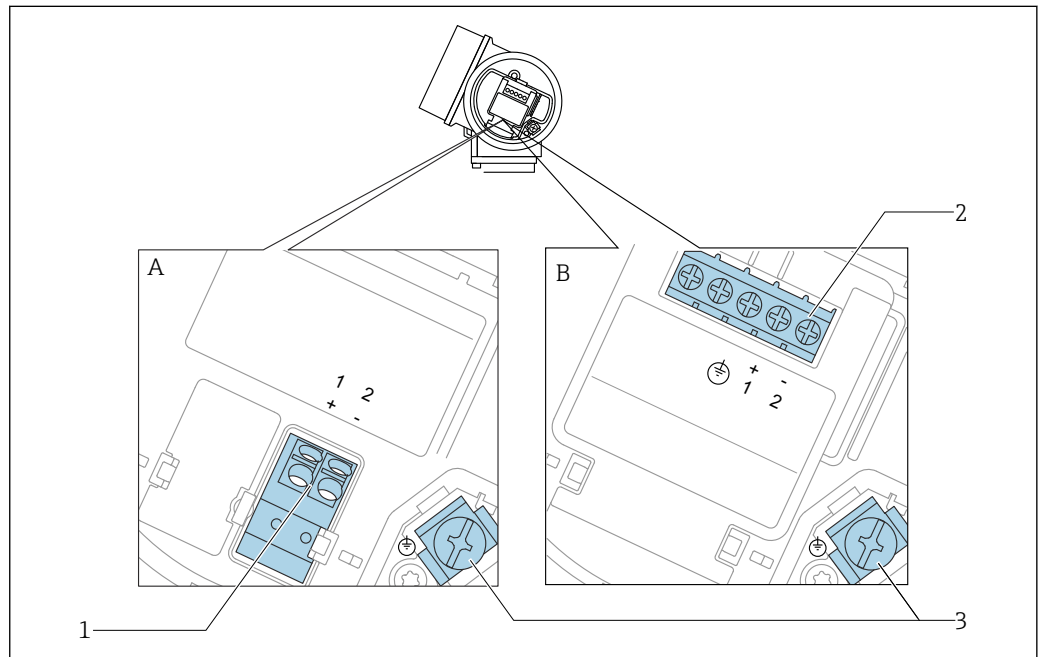
図 6 2 線式、4-20 mA HART の端子割当て
