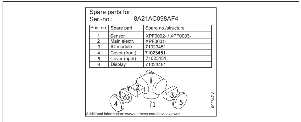
図 34 端子部カバーのスペアパーツ型式銘板の例
