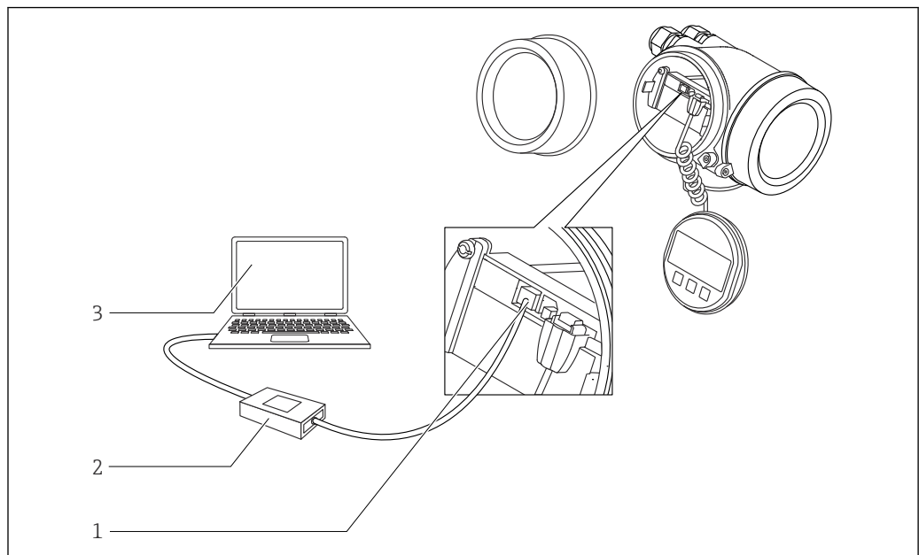
図 20 サービスインターフェイス (CDI) 経由の DeviceCare/FieldCare
