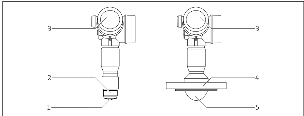
図 1 Micropilot FMR62 の構造
