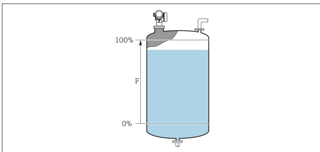
☒ 37 液体レベル測定用の満量校正 (F)
