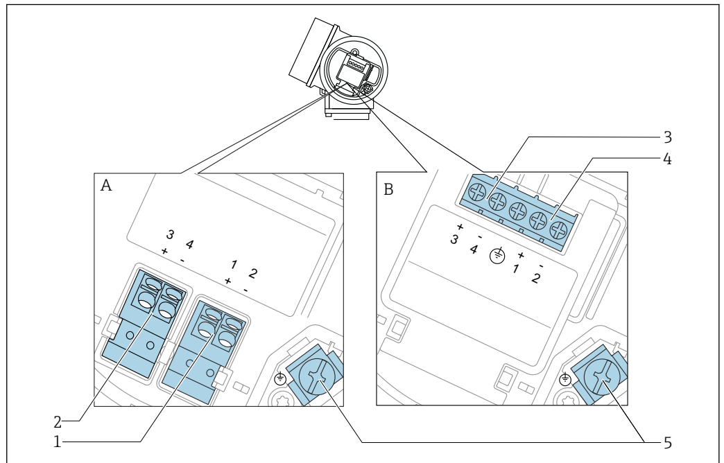
図 10 2線式、4~20 mA HART、4~20 mA の端子割当て
