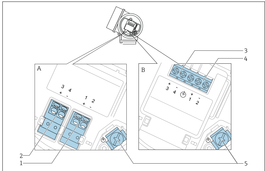
図 8 2線式、4~20 mA HART、スイッチ出力の端子割当て
