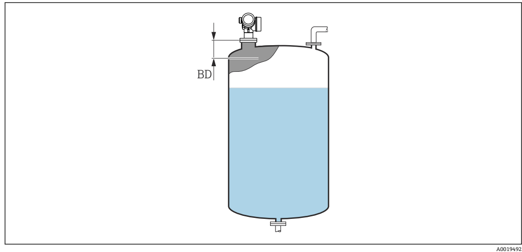
図 39 液体計測の不感知距離 (BD)
