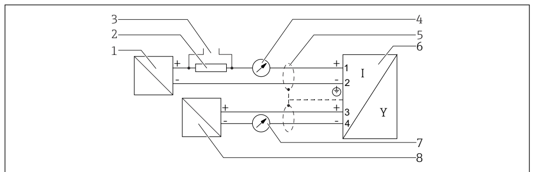
図 11 ブロック図：2線式、4~20 mA HART、4~20 mA
