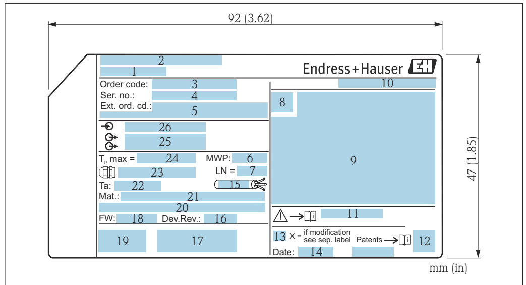
図 4 Micropilot の銘板
