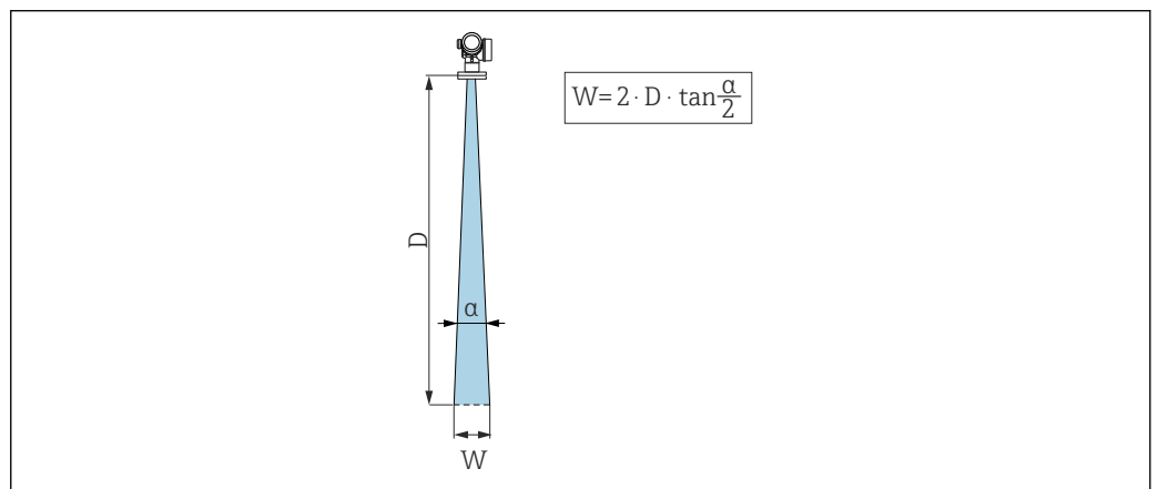
図 5 ビーム放射角 \alpha 、距離 D 、ビーム幅 W の関係
