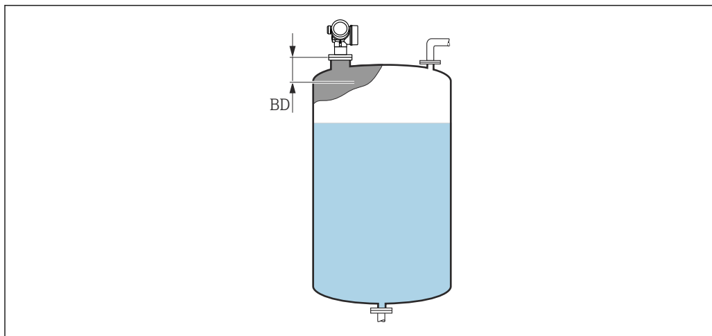
図 43 液体計測の不感知距離 (BD)
