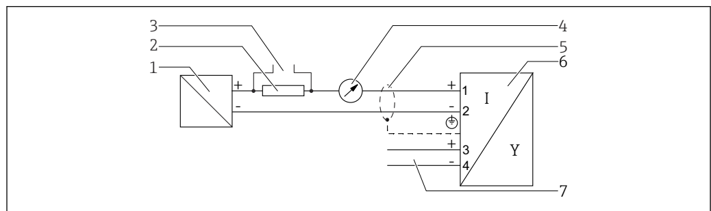
図 9 ブロック図：2線式、4~20 mA HART、スイッチ出力
