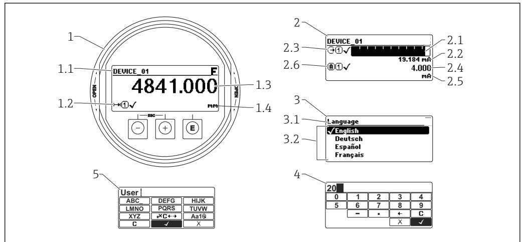
図 21 現場操作用の表示部および操作モジュールの表示
