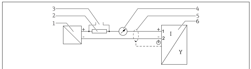
図 7 ブロック図：2 線式、4~20 mA HART
