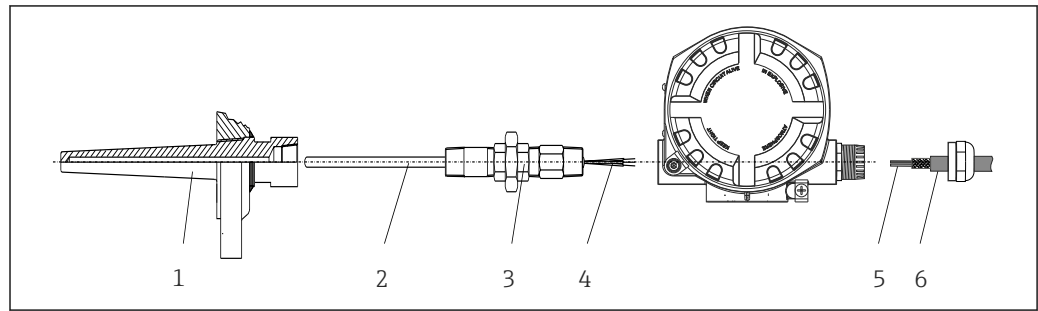
図4 センサにフィールド伝送器を直接取付け
