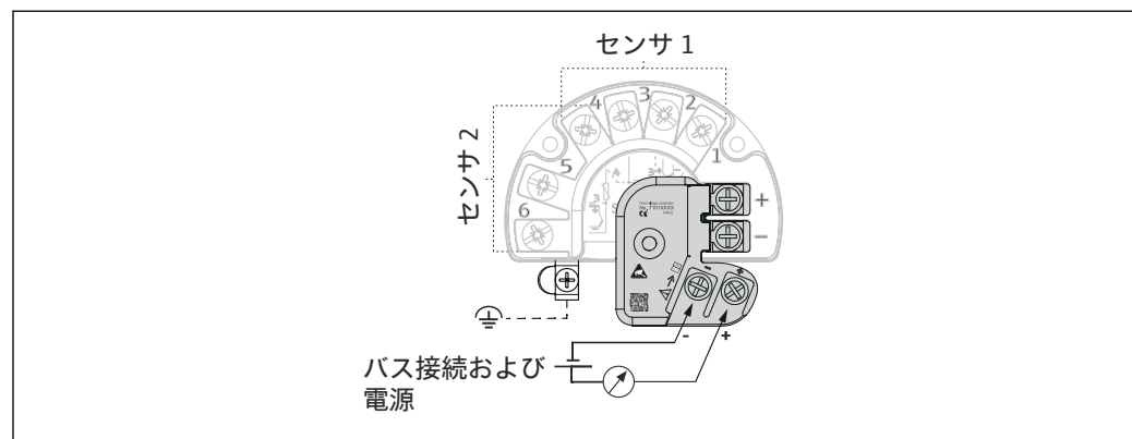
図 3 サージアレスタの電気接続
