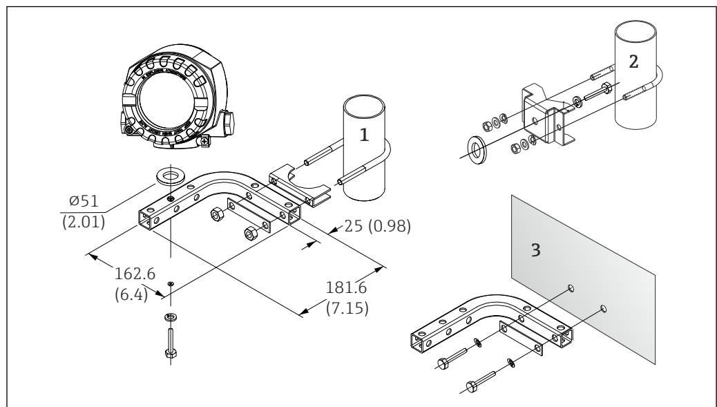
図5 取付ブラケットを使用したフィールド伝送器の設置（「アクセサリ」セクションを参照）。寸法単位：mm (in)
