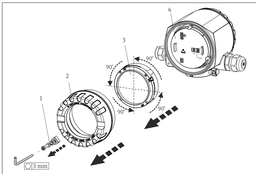
図 6 4 x ディスプレイの取付位置、90° 単位で脱着可能
