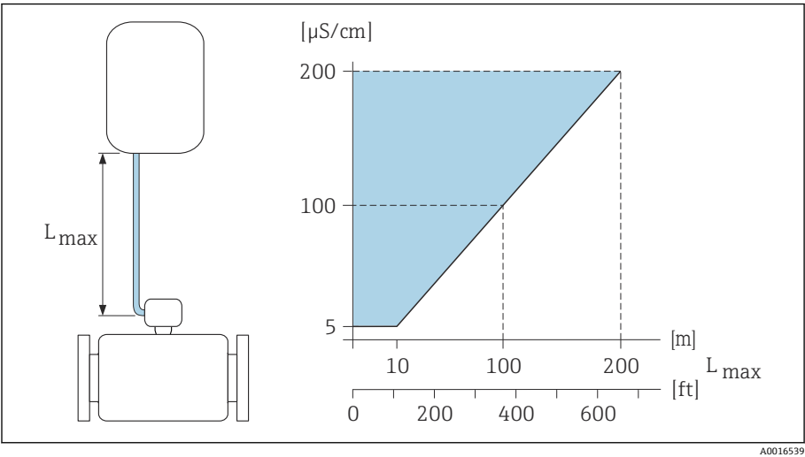
図 4 許容される接続ケーブル長
