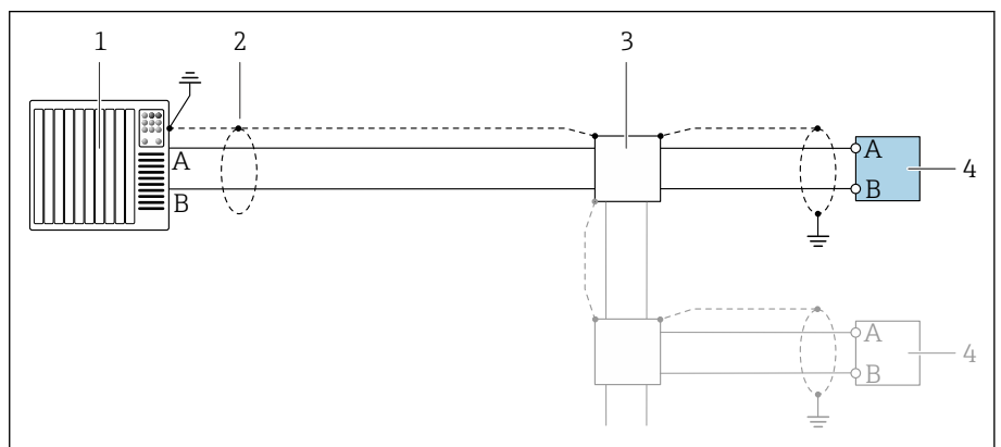
図 2 Modbus RS485（非危険場所および Zone 2 ; Class I、Division 2）の接続例
