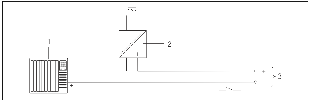
11 Esempio di connessione per l'uscita contatto (passiva)
