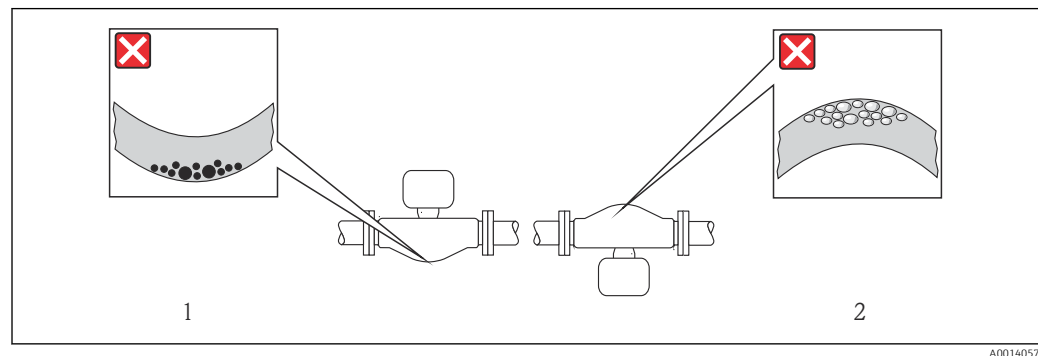
☒ 20 Orientamento del sensore con tubo di misura curvo
