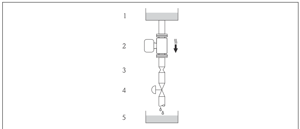
19 Installazione in un tubo a scarico libero (ad es. per applicazioni di dosaggio)
