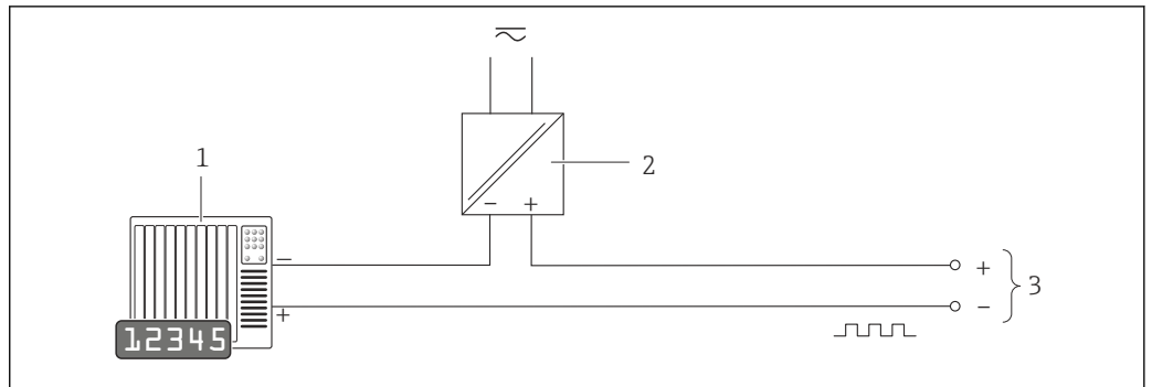
10 Esempio di connessione per l'uscita impulsi/frequenza (passiva)
