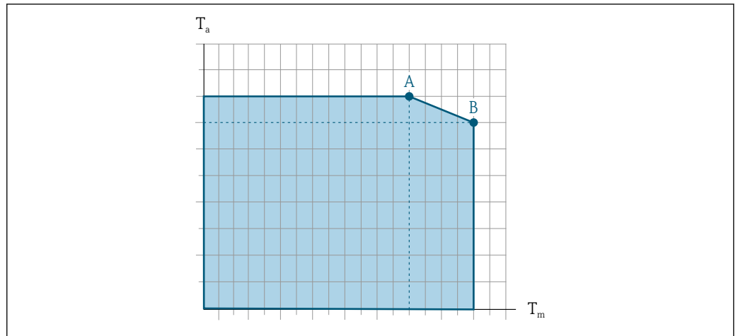
23 Rappresentazione esemplificativa, valori nella tabella sottostante.
