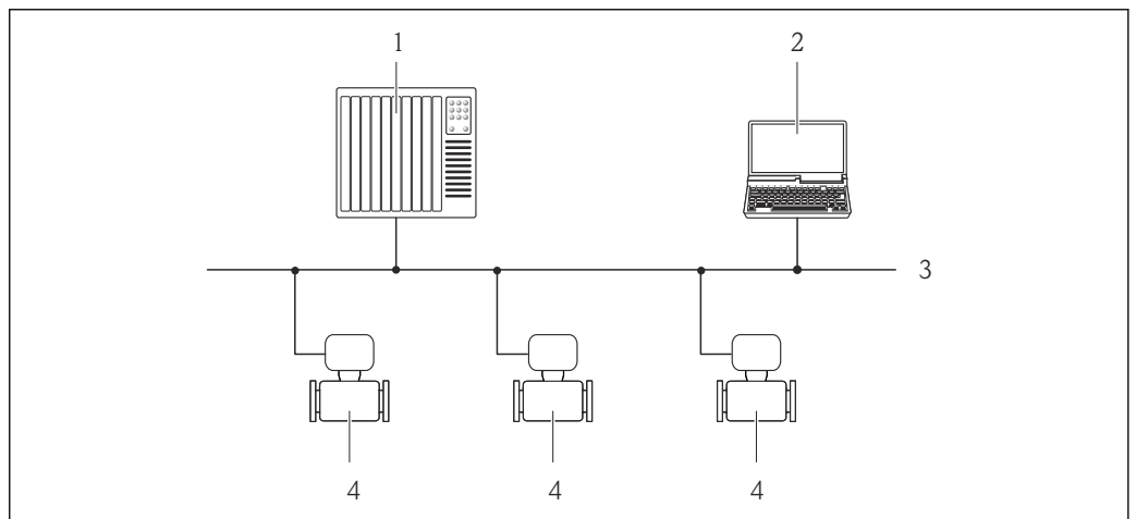
31 Opzioni per il funzionamento a distanza mediante rete PROFIBUS DP
