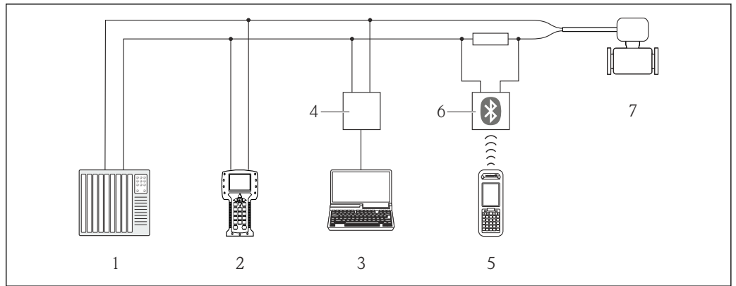
30 Opzioni per il funzionamento a distanza mediante protocollo HART
