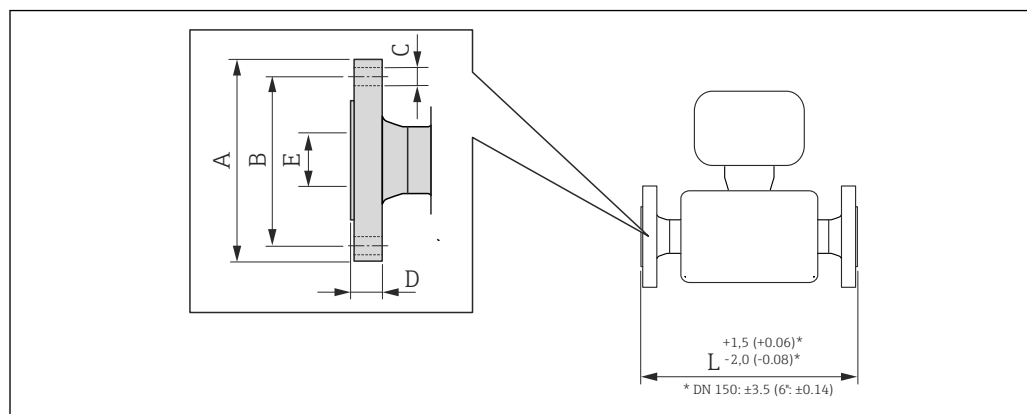
28 Unità ingegneristica, mm (in)
