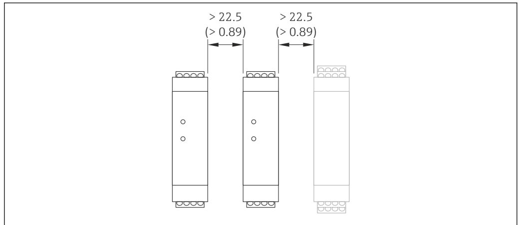
21 Distanza minima tra la Barriera di sicurezza Promass 100 o altri moduli. Unità ingegneristica mm (in)
