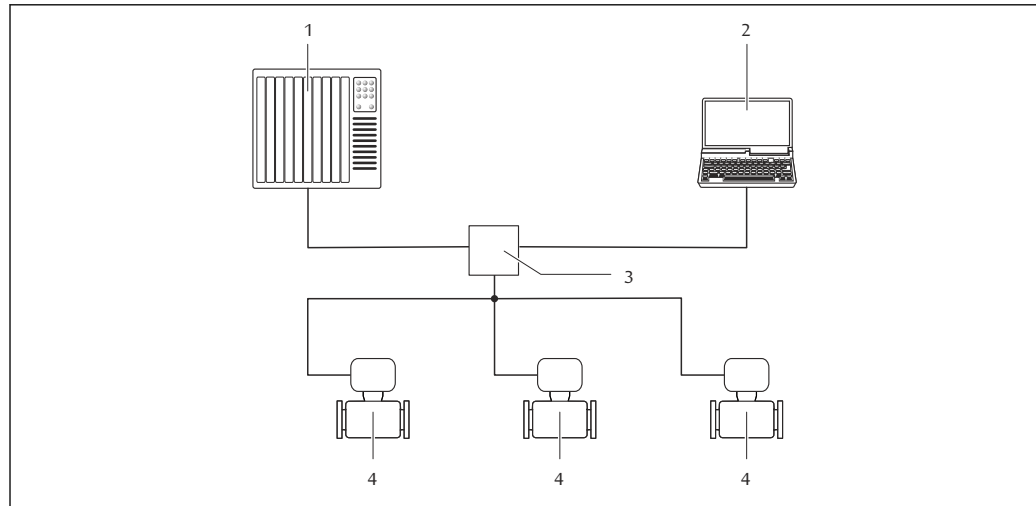
33 Opzioni per il funzionamento a distanza mediante rete PROFINET
