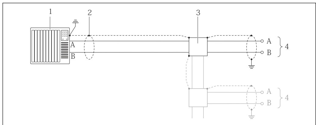
13 Esempio di connessione per Modbus RS485, area sicura e Zona 2/Div. 2
