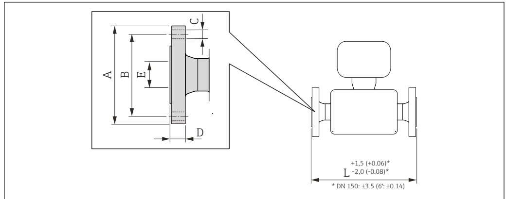
27 Unità ingegneristica, mm (in)
