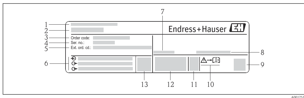
Fig. 2 Esempio di targhetta del trasmettitore
