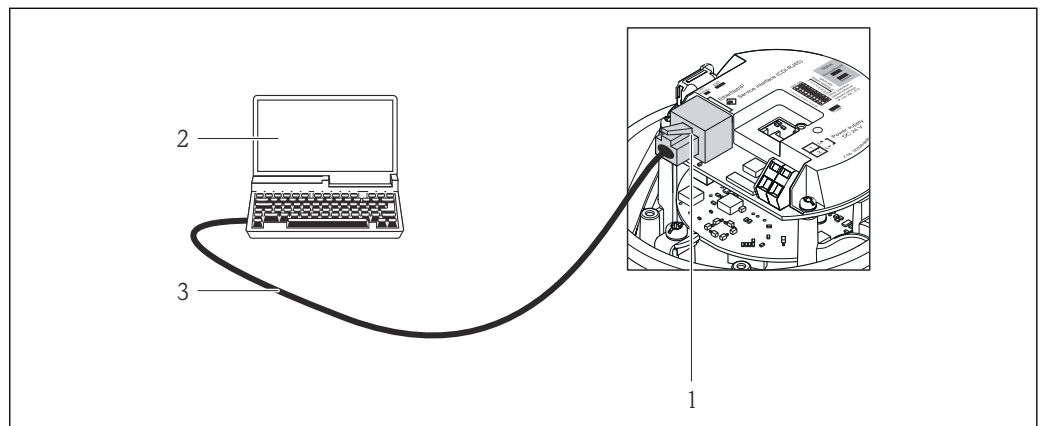
42 Raccordement pour variante de commande "Sortie", option N : EtherNet/IP
