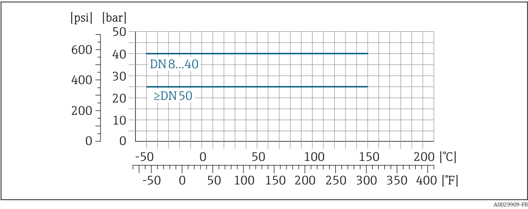
27 Avec matériau de bride 1.4435 (316L)
