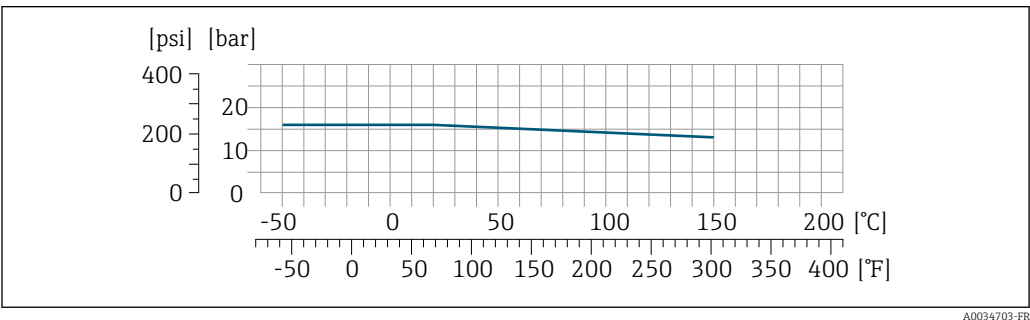
29 Avec matériau de raccord 1.4435 (316L)
