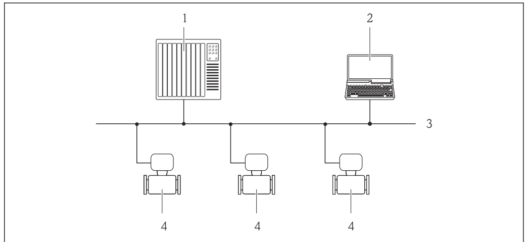
37 Possibilités de configuration à distance via réseau PROFIBUS DP
