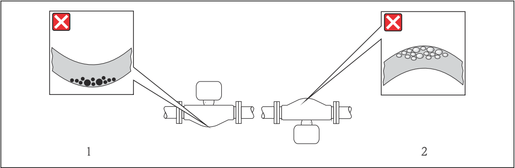
☒ 19 Orientation du capteur avec tube de mesure coudé
