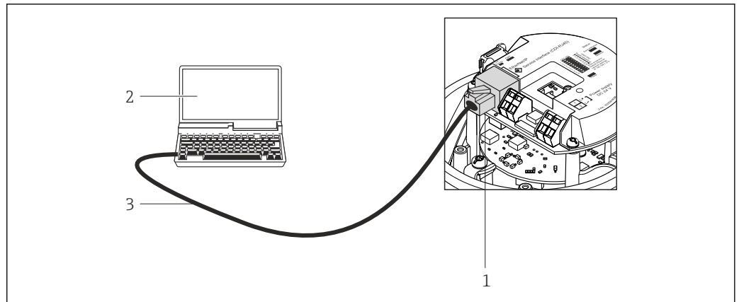
41 Raccordement pour variante de commande "Sortie", option L : PROFIBUS DP
