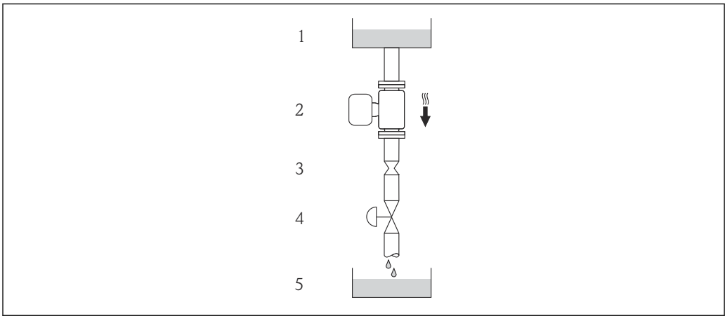
18 Montage dans un écoulement gravitaire (par ex. applications de dosage)
