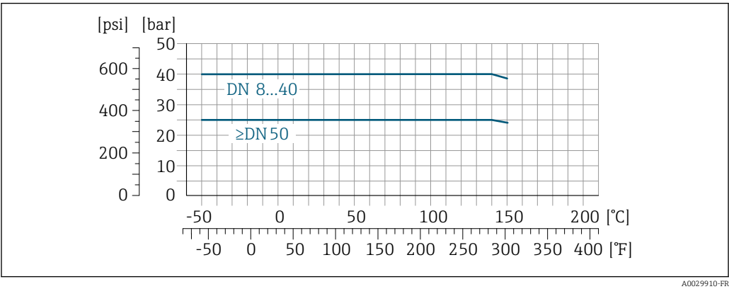
28 Avec matériau de raccord 1.4435 (316L)
