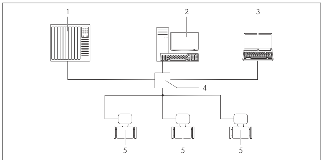
38 Options de configuration à distance via bus de terrain basé sur Ethernet
