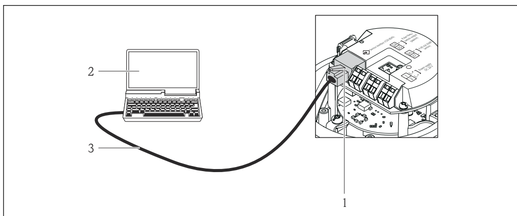
40 Raccordement pour variante de commande "Sortie", Option B : 4-20 mA HART, sortie impulsion/fréquence/tor
