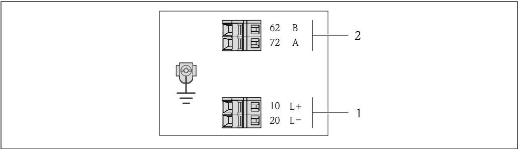
4 Occupation des bornes Modbus RS485, variante de raccordement pour l'utilisation en zone à sécurité intrinsèque (raccordement via barrière de sécurité Promass 100)
