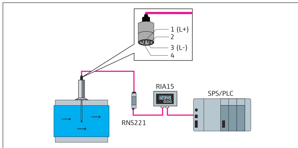
1 Conexión M12 con salida analógica de 4 ... 20 mA
