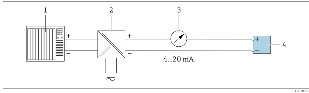
12 Esempio di connessione per uscita in corrente 4-20 mA (passiva)
