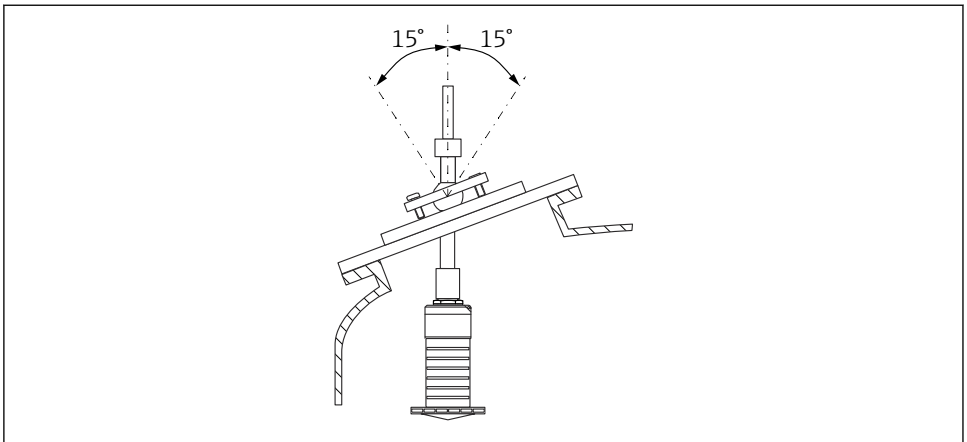
☞ 16 Micropilot FMR20 및 정렬 장치
