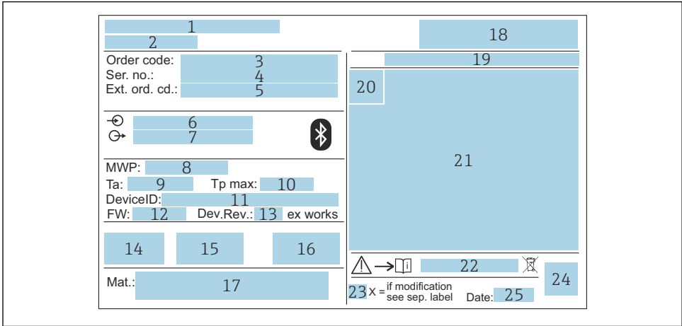
☐ 2 Micropilot 명판
