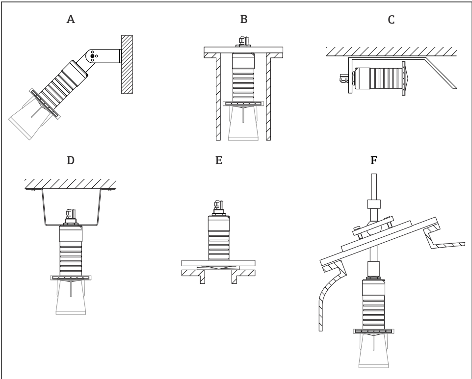
☞ 3 벽, 천장 또는 노즐 설치
