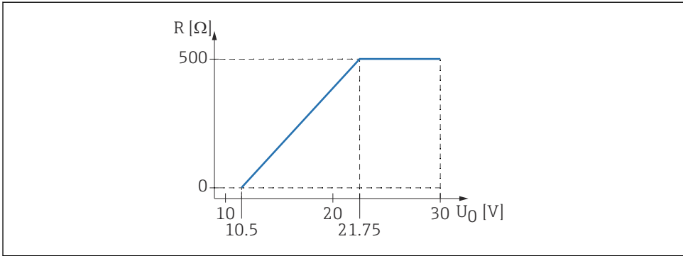
☞ 19 최대 부하 R, 전원 공급 장치의 공급 전압 U_0 에 따라 달라짐
