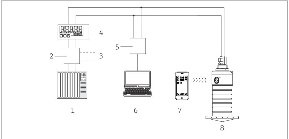
☐ 22 HART 프로토콜을 통한 원격 작동 옵션
