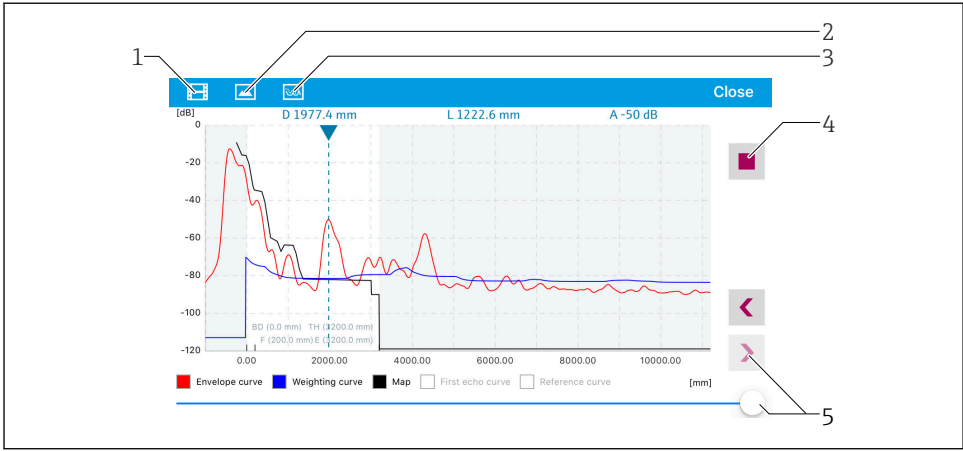
☐ 25 iOS용 SmartBlue에서 엔벨로프 커브 표시(예)
