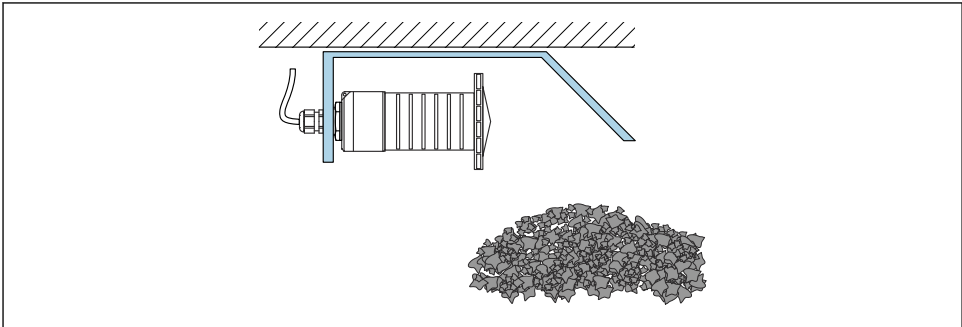
☐ 14 수평 설치 브래킷을 사용한 설치(침수 방지 튜브 없음)
