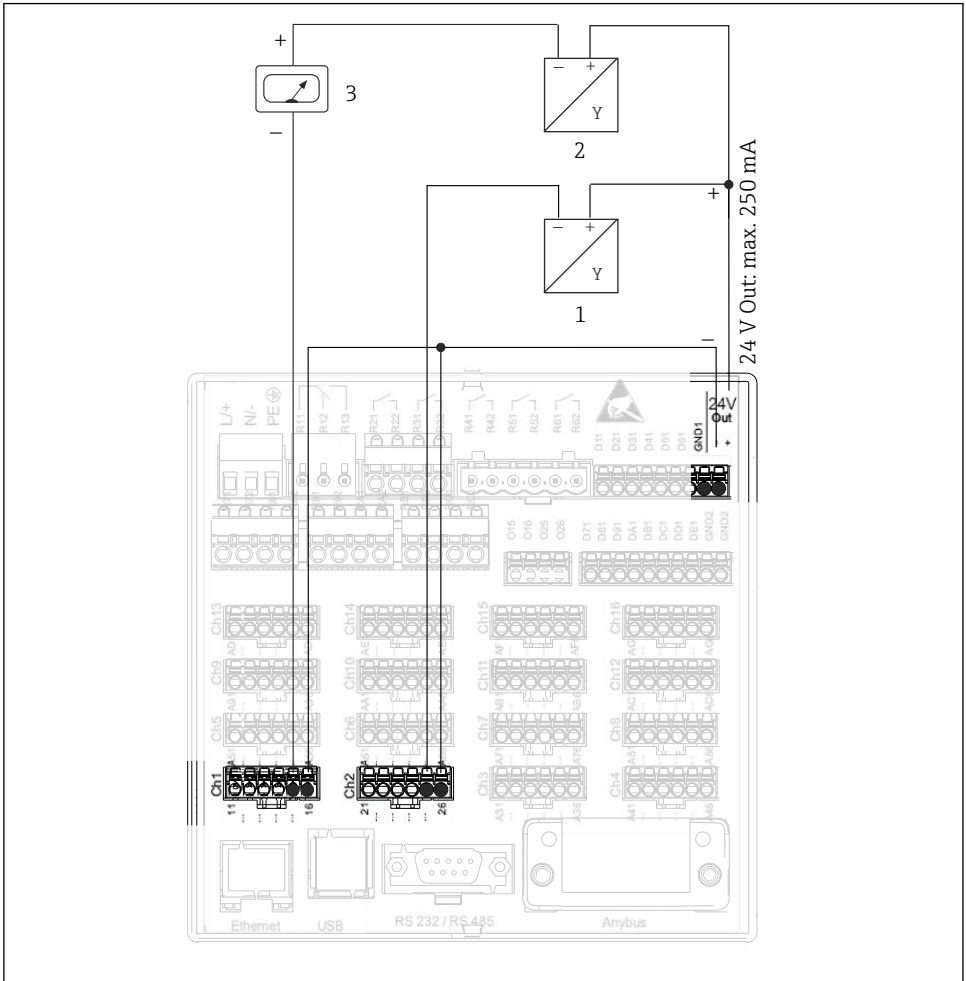
8 Anschluss des Hilfsspannungsausgangs bei Verwendung als Messumformerspeisung (MUS) für 2-Leiter-Sensoren im Strommessbereich
