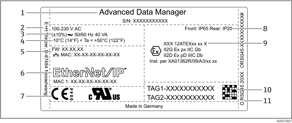
1 Typenschild des Gerätes (beispielhaft)
