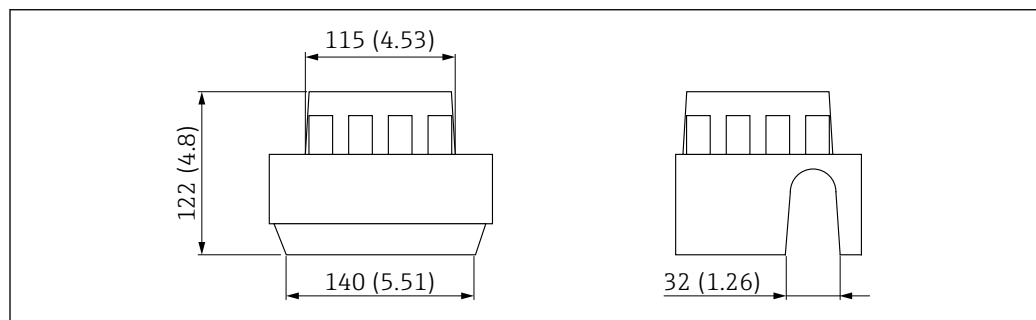
47 Pokrywa ochronna dla obudowy jednokomorowej, aluminium lub stal k.o. 316L. Jednostka miary mm (in)
