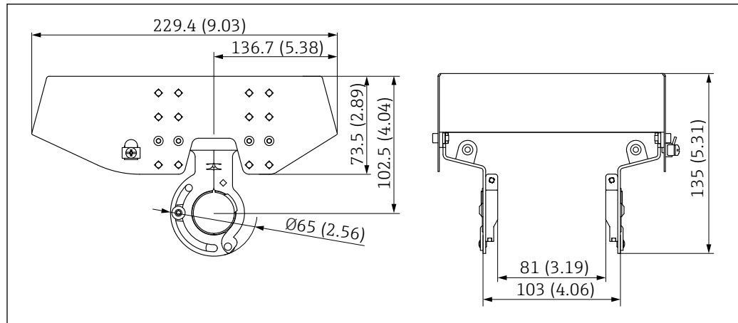
46 Osłona pogodowa do obudowy dwukomorowej, aluminium. Jednostka miary mm (in)
