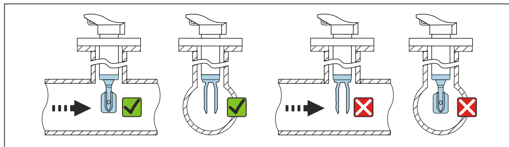
14 Montaż w rurociągach
