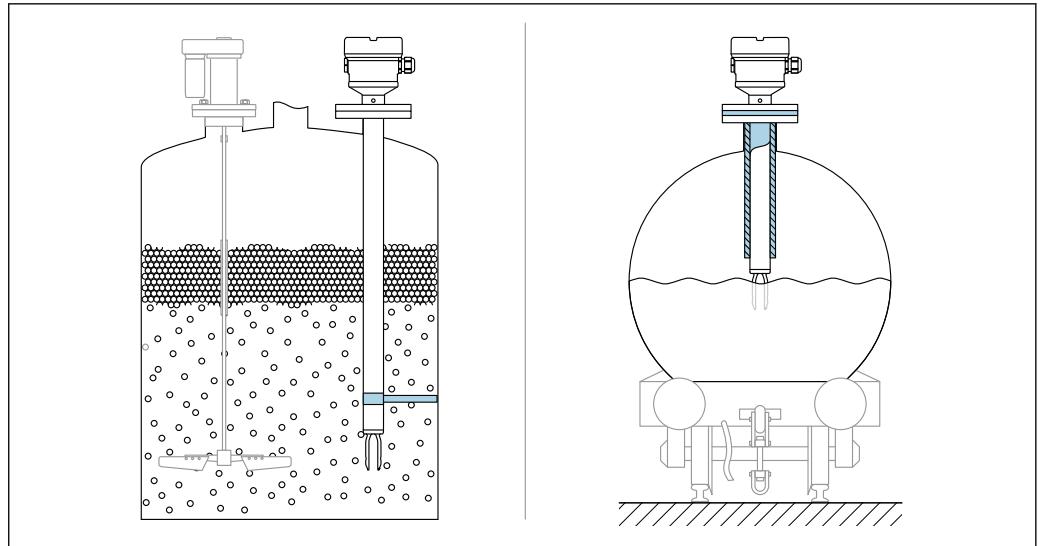
12 Przykładowe sposoby podparcia przy dużych obciążeniach dynamicznych
