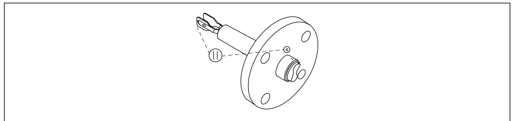
13 Znak na kołnierzu do ustawienia widełek sygnalizatora
