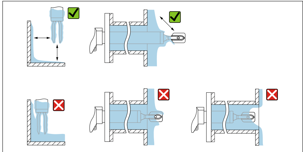
10 Przykłady montażu w medium procesowym o dużej lepkości
