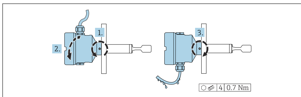
15 Obudowa z zewnętrznym wkrętem dociskowym
